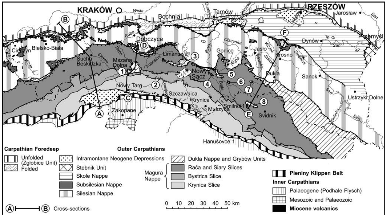
Fig. 1. Tectonic sketch of the Outer West Carpathians (based on Żytka et al. , 1989; simplified). Tectonic windows: 1 – Mszana Dolna, 2 – Szczawa, 3 – Kleczany–Pisarzowa, 4 – Grybów, 5 – Ropa, 6 – Uście Gorlickie, 7 – Świątkowa, 8 – Smilno
