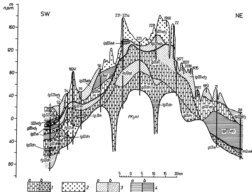
Fig. 3 Przekrój geologiczny poprzeczny (II) przez Przewężenie Karelskie. 1 – gliny zwalowe: a – wałdajskie, b – moskiewskie i dniewrowskie, 2 – żwiry, otoczaki i glaziki, 3 – piaski: a – limnoglacialne, b – fluwioglacialne, 4 – utwory limniczne: a – ily, mulki jeziorne i limnoglacialne wałdajskie, b – ily, mulki limnoglacialne przedwałdajskie. Zlodowacenie dniewrowskie: fgIIIdn – osady fluwioglacialne, gIIIdn – osady glacialne, lgIIIdn – osady limnoglacialne; zlodowacenie moskiewskie: lgIIIm – osady limnoglacialne, fgIIIm – osady fluwioglacialne, gIIIm – osady glacialne; zlodowacenie wałdajskie: gIIIvd1 – osady glacialne, IIIvd2 – osady limniczne, lgIIIvd3 – osady limnoglacialne
