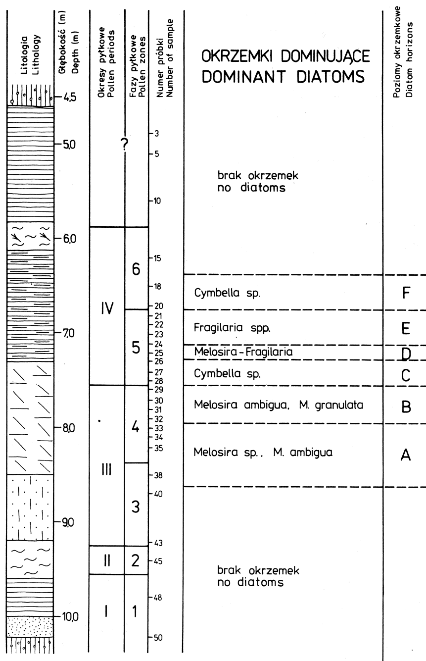
Fig. 4 Okrzemki dominujące w osadach interglacialnych stanowiska Fałęcice nad Pilicą. Litologia jak na Fig. 3
