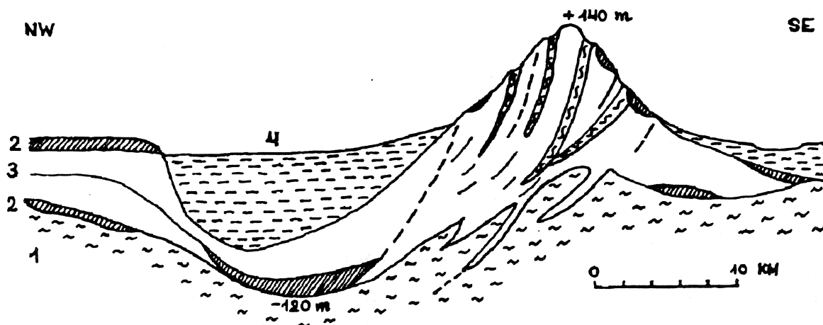
Fig. 16 Przekrój depresji Quakenbrück i grzbietu Dammer w Dolnej Saksonii (wg. Meyera, 1987, uproszczone) — przykład glaciotehtonopary w dużej skali. 1 — kreda i trzeciorzęd, 2-4 — czwartorzęd: 2 — gliny zwałowe, 3 — inne osady zlodowaceń starszych (głównie piaski), 4 — osady zbiornikowe (m.in. jeziorne) złożone wdepresjach, głównie z interglacjału eemskiego i zlodowacenia Wisły
