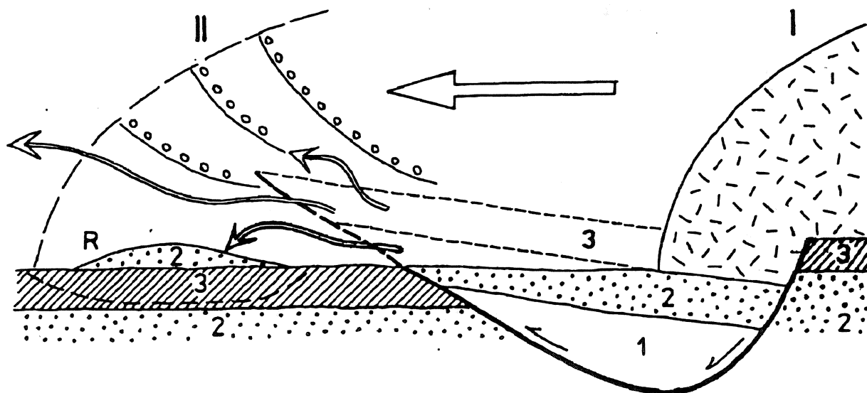
Fig. 20 Tworzenie kier typu glaciektonektonicznego w warunkach ścinania cylindrycznego. 1-3 – kolejne warstwy podłoża i przedpola lądolodu, R – kra glaciektonektoniczna o odwróconym następstwie stratygraficznym, I, II – kolejne zasięgi czoła lodu
