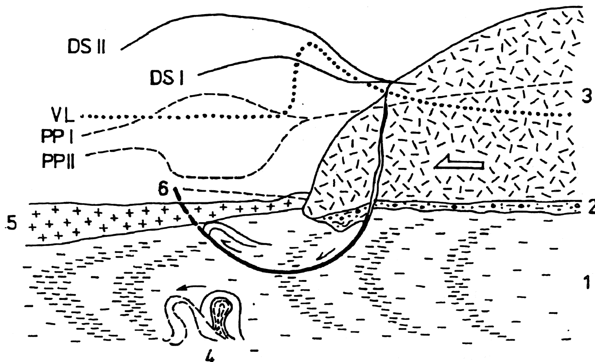
Fig. 18 Ścinanie cylindryczne u czoła lądolodu, w luźnym ośrodku ziarnistym reagującym dylatacyjnie i nasyconym wodą. 1 – podłoże niezamrożone, nasycone wodą wytłaczaną spod lądolodu, 2 – wytapiana morena denną, 3 – czoło lądolodu (w stanie stagnacji lub powolnej transgresji), 4 – fałdy diapirowe, 5 – wieloletnia zmarzlina, 6 – czoło ścinania cylindrycznego po przebiciu się ku powierzchni; oznaczenia literowe – orientacyjny obraz zmienności następujących charakterystyk podłoża: VL – poziomy gradient obciążenia pionowego, PP I, II – ciśnienie porowe przed i po przebiciu się ścinania cylindrycznego na powierzchnię, DS I, II – naprężenie dewiatorowe w dwu fazach j.w.
