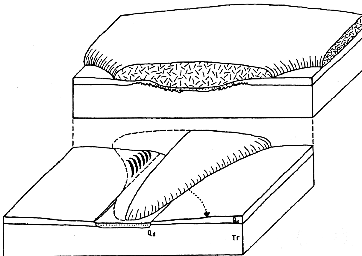
Fig. 9 Schemat koncepcji glacitektoniki krawędziowej w ujściu M. Bryczyńskiego (1982). Tr – trzeciorzęd, Q1 – czwartorzęd wysoczyzny, Q2 – osady rzeczne i rzecznołodowcowe w dolinie. Strzałką oznaczono kierunek transportu kier glacitektonicznych
