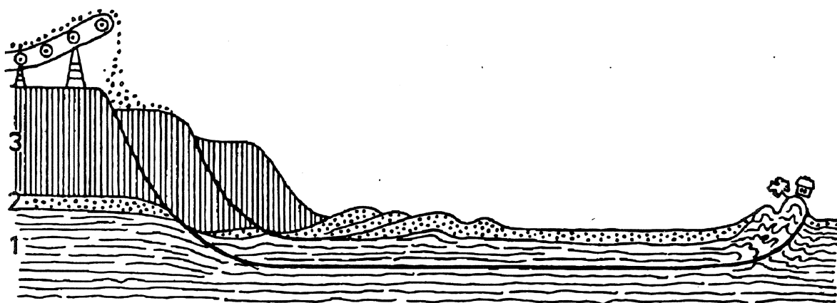
Fig. 14 Szkic deformacji koło kopalni Machów według interpretacji autora. 1 – iły krakowieckie (trzeciorzęd), 2 – piaski (czwartorzęd), 3 – zwał kopalni Machów
