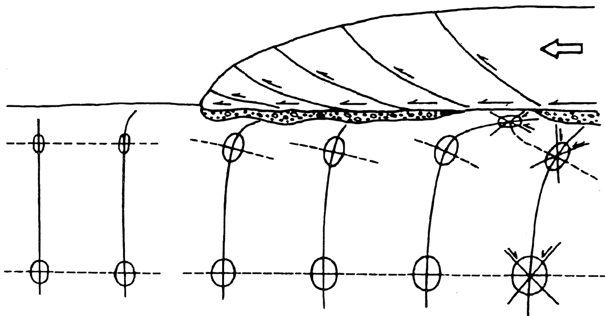
Fig. 1 Stan naprężeń pod strefą czołową lądolodu transgredującego na podłożu z niezamarzniętych osadów luźnych. Linie w podłożu lądolodu – trajektorie głównych naprężeń normalnych: linie ciągłe – największego ( \sigma_1 ), linie przerywane – najmniejszego ( \sigma_3 ); elipsy – schematyczny obraz przypuszczalnego tensora naprężeń
