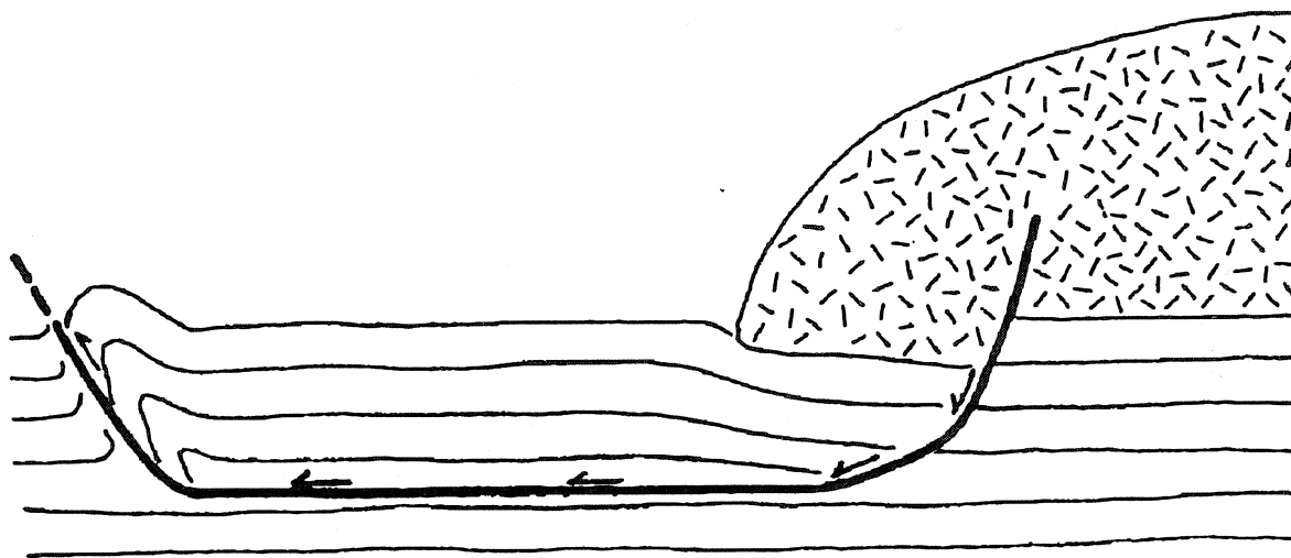
Fig. 12 Efekty strukturalne ścinania cylindrycznego u czoła lądolodu, w ośrodku anizotropowym
