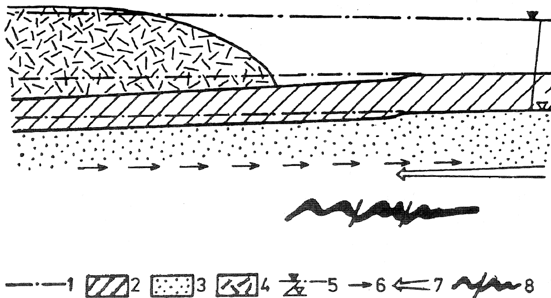
Fig. 10 Mechanizm hydroglacitektonicznej stymulacji dla zaburzeń glacitektonicznych (wg. Michalskiego, 1979). 1 – pierwotne położenie kompleksu wieloletniej zmarzliny, 2 – położenie tego kompleksu w trakcie nasuwania się lądolodu, 3 – utwory nie zmarznięte, 4 – lądolód, 5 – linia ciśnień piezometrycznych wód podzmarzlinowych, 6 – plastycznolepkie płynięcie gruntów pod lądolodem, 7 – odpór gruntu na przedpolu, 8 – strefa powstawania dużych deformacji glacitektonicznych
