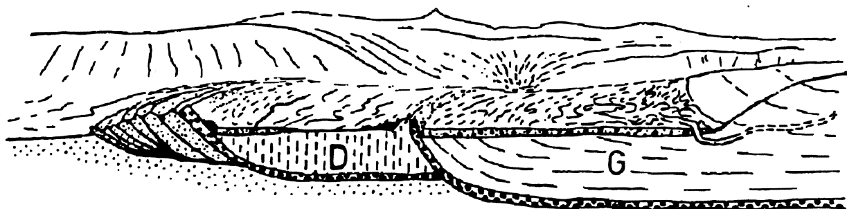
Fig. 3 Przekrój interpretacyjny przez czoło dolnego lodowca Usher na Spitsbergenie (wg. Grippa, 1975 fide Eissmann, 1987). G – lodowiec, D – lód martwy
