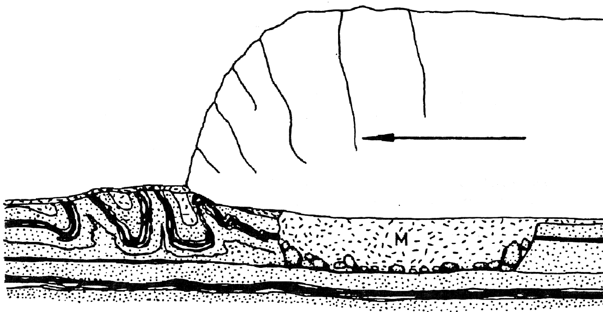
Fig. 2 Fałdowanie glacitektoniczne według J. Zwierzyckiego (1949). M – morena denną przymarznąłą do lodowca
