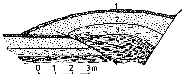
Fig. 13 Struktura z początkowej fazy wypory przedpola zwałowiska kopalni w Machowie (wg. Furmańskiego et al. , 1973). 1 – zadarniona gleba, 2-3 – piasek, 4 – il pylasty
