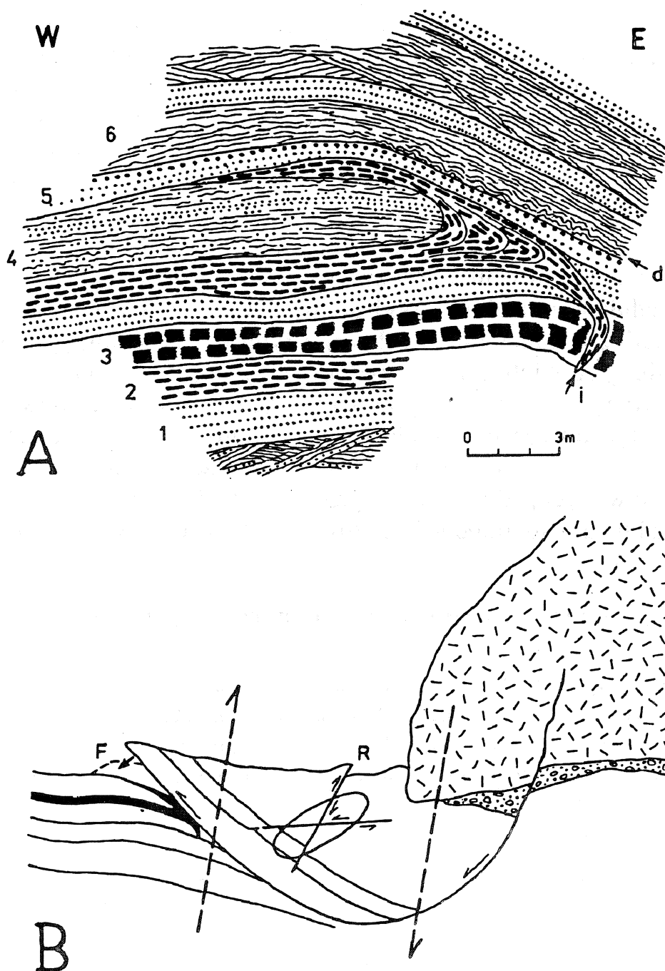
Fig. 21 Pochodzenie struktur glacitektonicznych o wstecznej wergencji. A – glacitektoniczny pseudofałd leżący w utworach miocenijskich Dobrzyń nad Wisłą (Góra Zamkowa, sytuacja z r. 1960). 1 – piasek pylasty, 2 – mułek węglisty, 3 – węgiel brunatny z partiami lignitowymi, 4 – mułek piaszczysty, 5 – piasek średnioziarnisty z wkładką drobnego żwiru, 6 – mułek lokalnie piaszczysty; d – strefa fałdeków typu ciążnionego, i – iniekcja mułku węglistego w przedłużeniu przegubu fałdu. B – wyjaśnienie genezy pseudofałdu dobrzyńskiego (F) i wstecznych uskokuw inwersyjnych (R)
