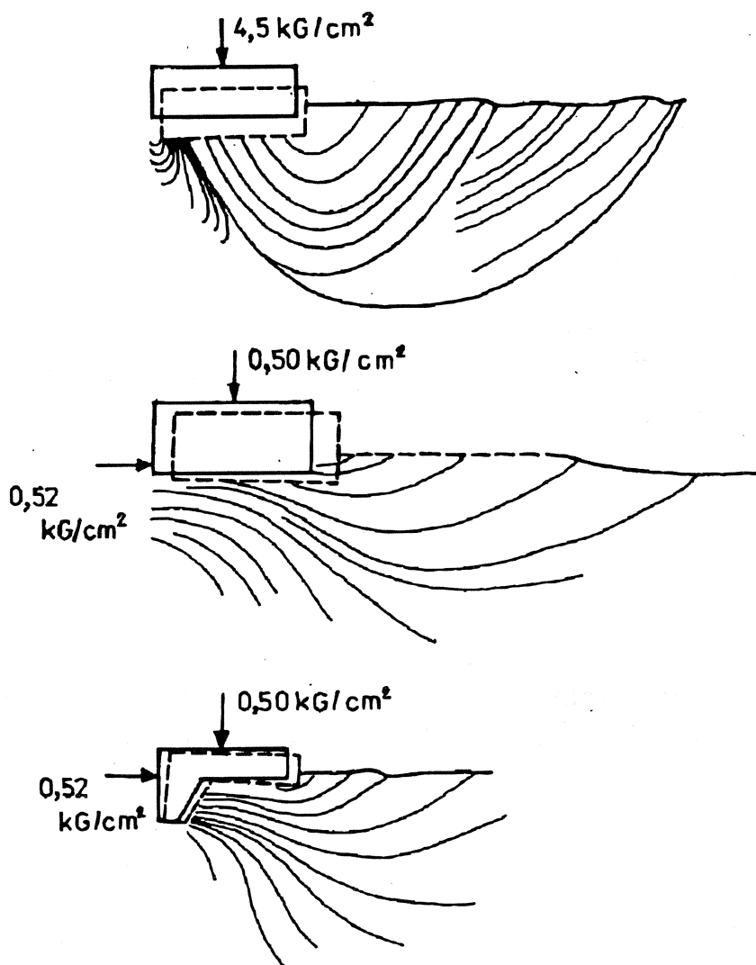
Fig. 15 Powierzchnie ścinania cylindrycznego uzyskane doświadczalnie w piasku, przy różnych warunkach obciążenia (wg. Florina, 1961)
