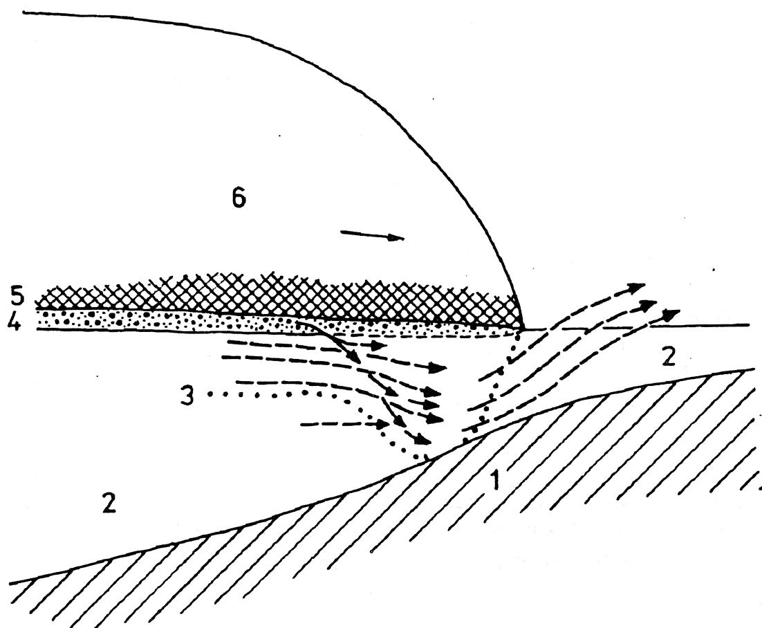
Fig. 4 Schemat powstawania depresji glaciotektonicznych według H. Ruszczyńskiej-Szenajch (1976). 1 – twarde podłoże, 2 – miękkie podłoże, 3 – szkieletowy układ naprężeń, 4 – świeżo wytopiona, nieskonsolidowana morena denna, 5 – morena denna wmarznięta w lód, 6 – transgredujący lądolód; strzałki – wyciskanie materiału miękkiego podłoża przed czoło lądolodu oraz wciskanie takiego materiału i odmarniętej moreny do tworzącej się depresji
