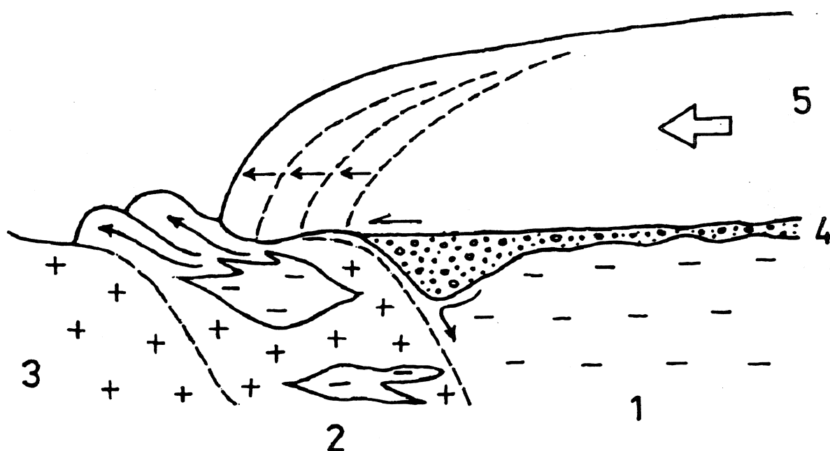
Fig. 5 Ewentualny mechanizm tworzenia depresji glaciotektonicznych przez zdrapywanie osadów wleczonych przez lądolód u brzegu obszaru wieloletniej zmarzliny. 1 – podłoże odmarzniete, 2 – strefa pośrednia, 3 – wieloletnia zmarzlina, 4 – osady transportowane pod lodem (morena denną, kry glacialne), w trakcie wytapiania, 5 – lądolód i kolejne linie jego zasięgu
