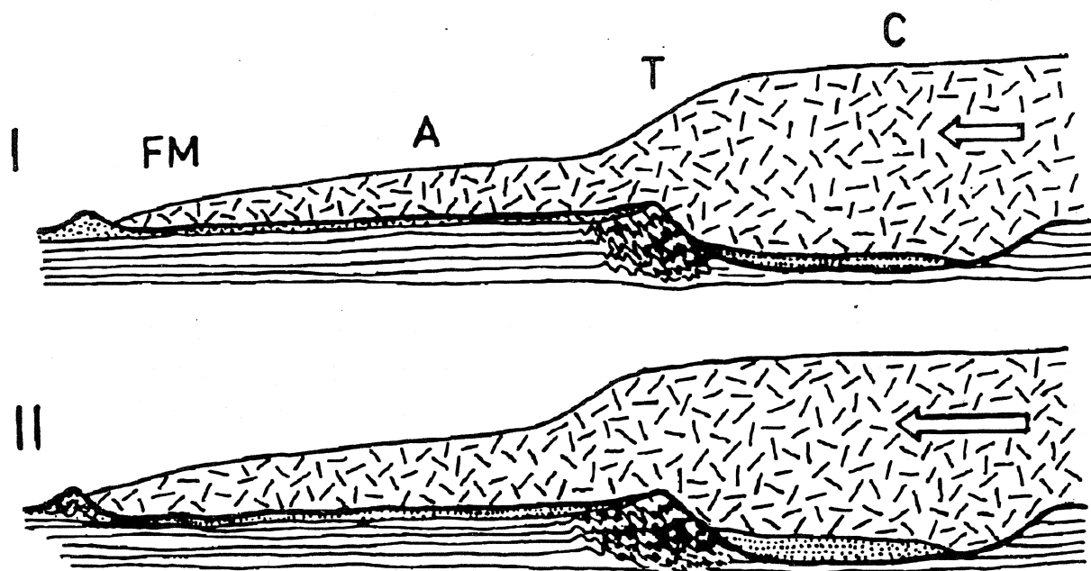
Fig. 7 Lokalizacja głównych stref zaburzeń glacitektonicznych według K. Brodzikowskiego (1980, fragment). I, II – stadia rozwoju deformacji w okresie transgresji, FM – strefa czołowa i marginalna, A – strefa ablacyjna, T – strefa przejściowa, C – centralne pole lądolodu
