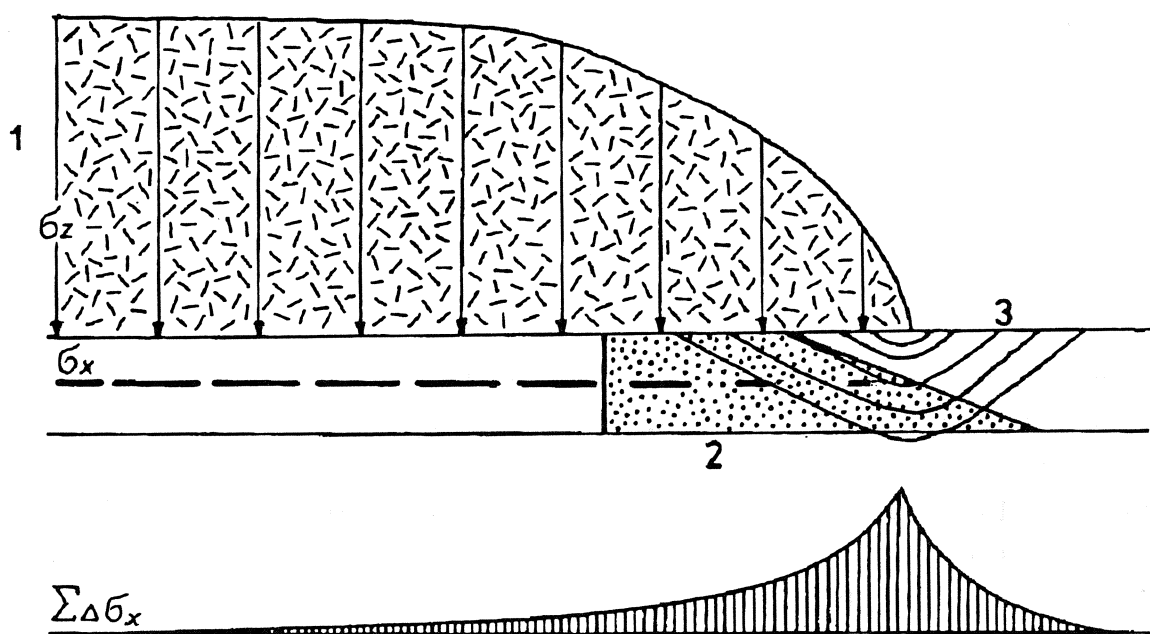
Fig. 6 Okoliczności powstawania wielkich deformacji glacitektonicznych według K. Rotnickiego (1974, uproszczone). 1 – lądolód, 2 – strefa powstawania wielkich fałdów, 3 – powierzchnie ślizgowe; \sigma_z – nacisk statyczny lądolodu, \sigma_x – naprężenia poziome, \Sigma\Delta\sigma_x – przyrost nacisku bocznego (suma przyrostu różnic naprężeń poziomych)
