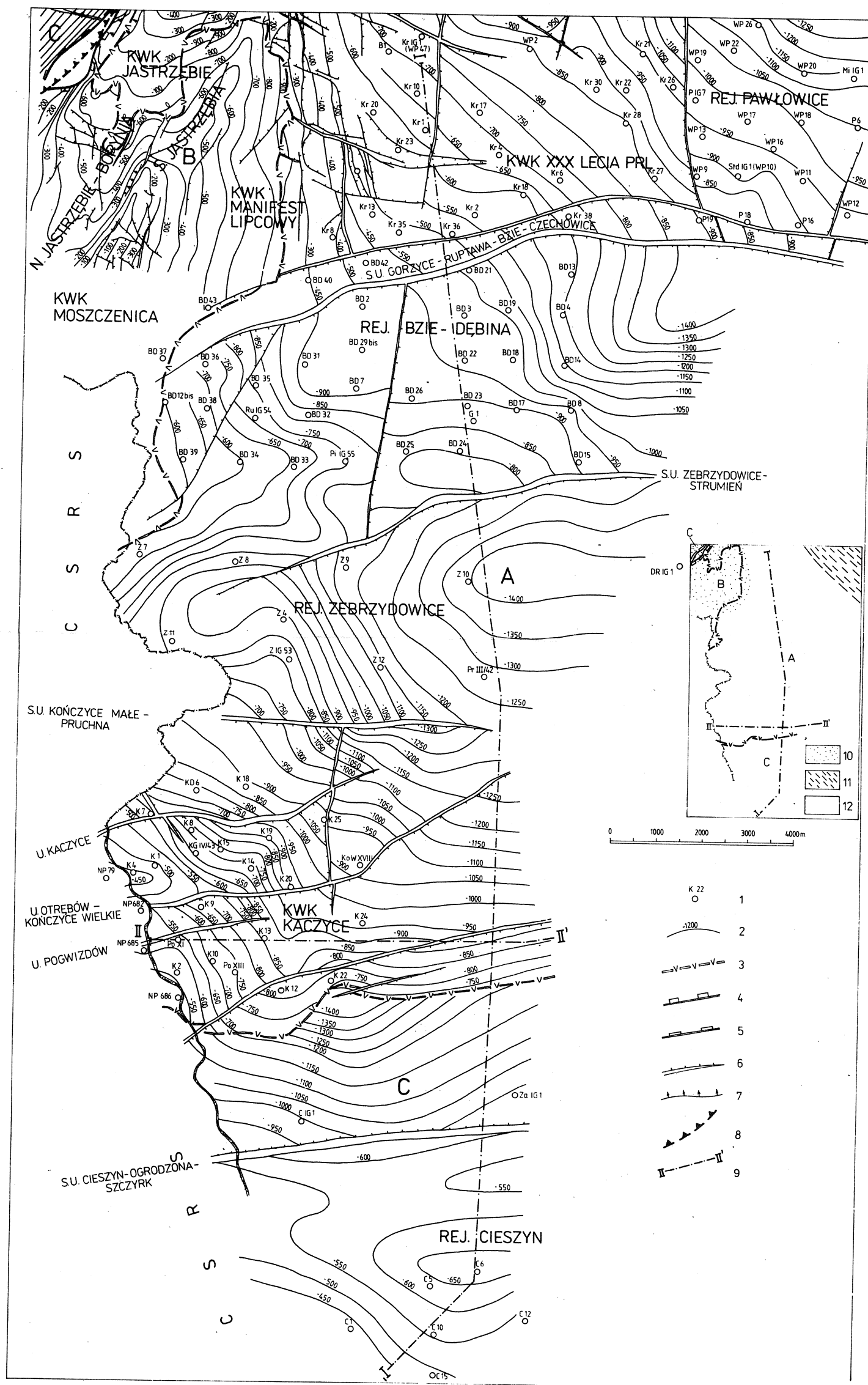
Fig. 2. Mapa strukturalna utworów karbonu górnego (odwzorowano spąg wybranych poziomów). 1 - otwory wiertnicze wykorzystane przy sporządzaniu mapy (nie zaznaczono otworów położonych na obszarach górniczych większości czynnych kopalń węgla kamiennego), 2 - izohipsy: w strefie A izohipsy spągu pokładu 405, w strefie B izohipsy spągu pokładu 510, w strefie C izohipsy spągu warstw jakłowieckich, 3 - wychodnia pokładu 405, 4 - wychodnia pokładu 510, 5 - wychodnia pokładu 722, 6 - uskoki normalne, 7 - uskoki odwrocone, 8 - nasunięcie boguszowickie, 9 - linie przekrojów geologicznych, 10 - strefa tektoniki fałdowej, 11 - strefa tektoniki uskoku, 12 - strefa tektoniki fałdowo-uskokowej; U. - uskok, S.U. - strefa uskoku, S. - siodło, N. - niecka, KWK - kopalnia węgla kamiennego, Rej. - rejon
