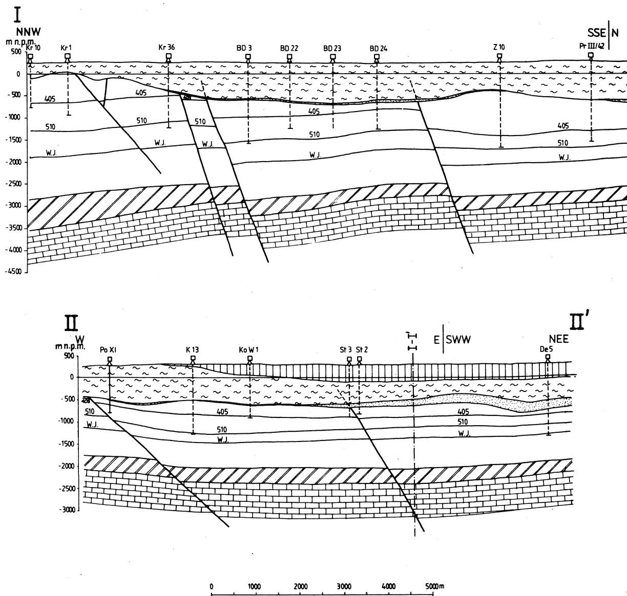
Fig. 4. Przekroje geologiczne (przekrój I–I' prowadzono wzdłuż profilów sejsmicznych 3-IV-77 PPG wiertnicze ( a – leżące w płaszczyźnie przekroju, b – rzutowane), 2 – flisz karpacki, 3 – miocen autochtoniczny i warstwy poddębowieckie (karpat), 5 – utwory produktywne karbonu górnego (405 – pokład 405, namuru A oraz wizenu górnego, 7 – utwory węglanowe wizenu i turneju
