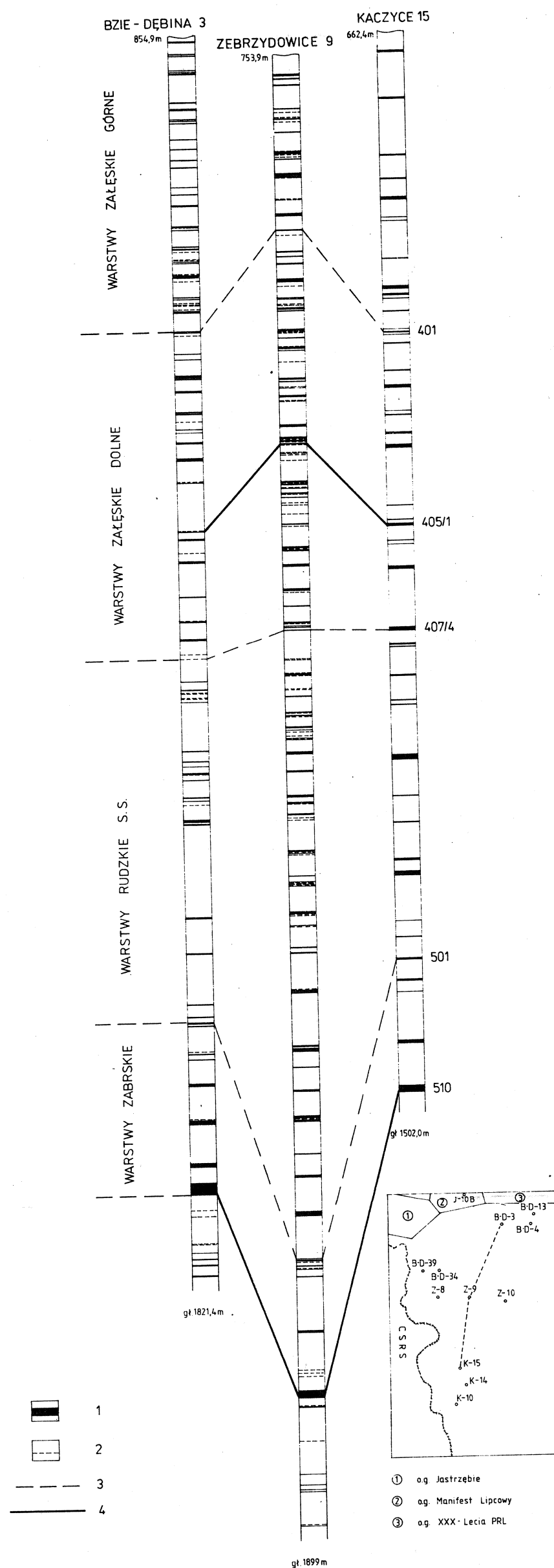
Fig. 1. Zmiany grubości serii węglonośnej i pozycja przewodnich pokładów węgla w wybranych profilach wiertniczych. 1 – pokład węgla, 2 – łupek węglowy, 3 – granice ogniw litostratigraficznych, 4 – linie korelacyjne przewodnich pokładów węgla, o.g. – obszar górniczy, 501 – numeryczne nazwy pokładów
