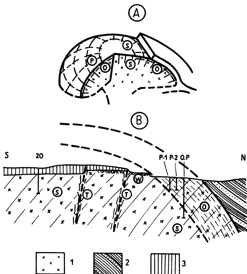
Fig. 7. Schematy ilustrujące dwuwarstwowość lakołitu załaskiego. A – spękania termiczne wg Dżułyńskiego (1955). S – cios stożkowy, P – cios promienisty, O – cios obwodowy, T – cios tektoniczny, B – Dwuwarstwowość lakołitu. 1 – porfiry permskie, 2 – iłolupki i piaskowce karbonu, 3 – piaski, piaskowce, wapień i margle jury
