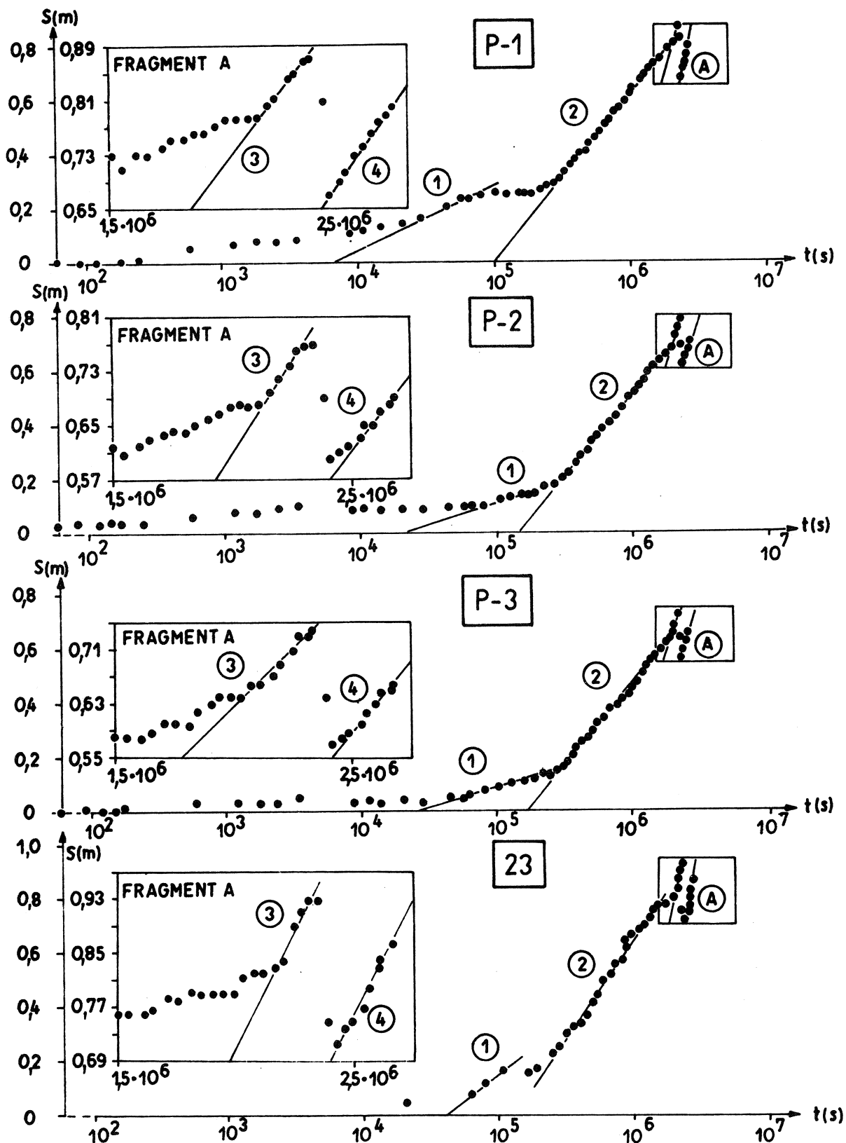
Fig. 5. Wykresy wskaźnikowe opadania zwierciadła w piezometrach P-1, P-2, P-3 oraz w otworze 23
