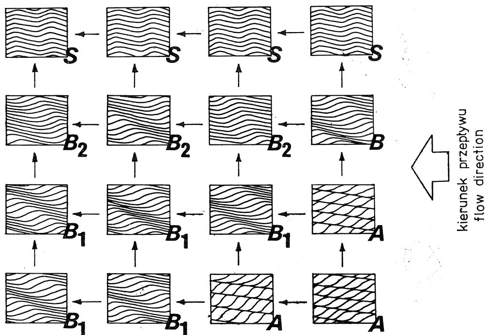
Fig. 2. Schemat sekwencji strukturalnych w centralnej części wypełnienia rozmycia erozyjnego — człon c (przekrój podłużny). Strzałki wskazują kierunek zmian strukturalnych sekwencji
