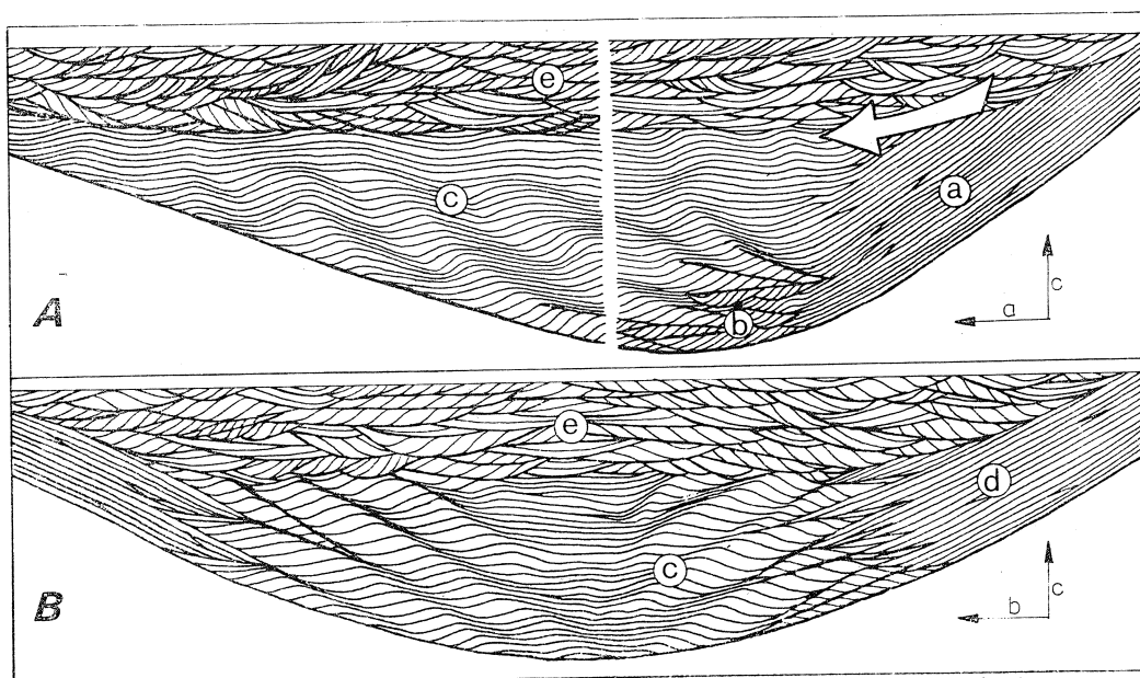
Fig. 4. Zbiorczy schemat struktur osadów wypełniających rozmycia erozyjne. Skala 1 : 25. A — w przekroju podłużnym; B — w przekroju poprzecznym. Opis w tekście Fig. 4. Compiled structural scheme of sediments infilling erosional washouts. Scale 1 : 25. A — in longitudinal section; B — transverse-section. Description in text
