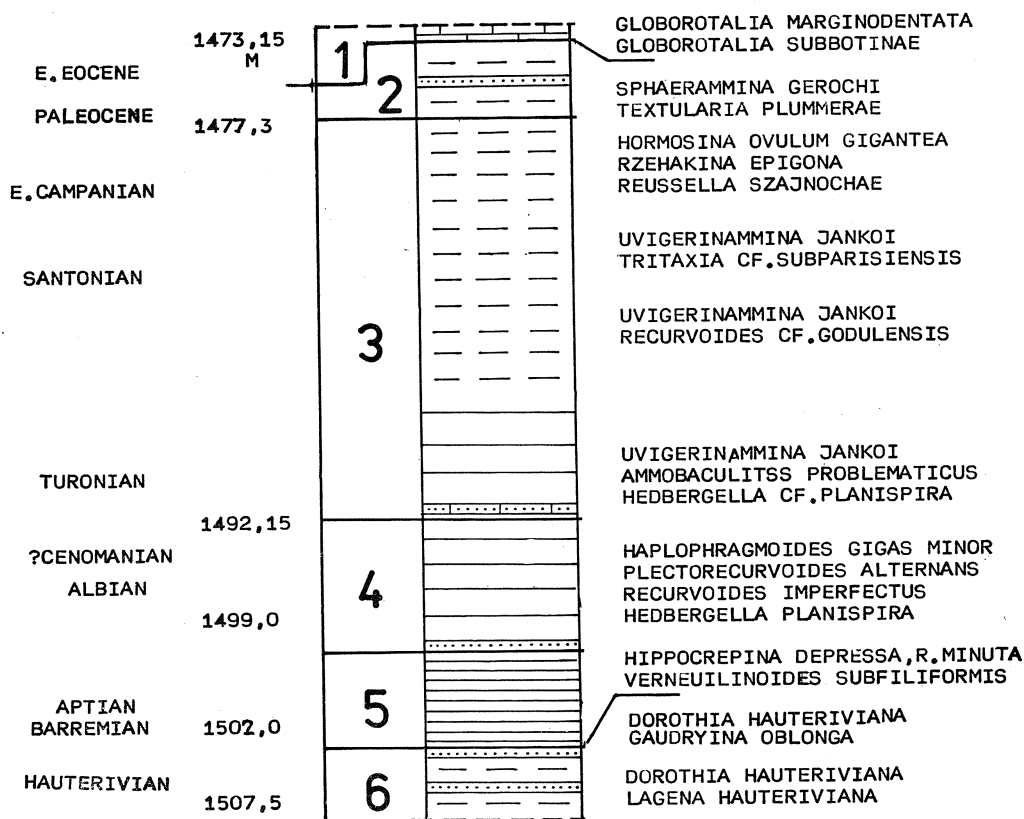
Fig. 5. Profil litostratygraficzny płaszczowiny śląskiej „zewnątrznej” w otw. Łodygowice IG-1. 1 — margle pstre; 2 — łupki szare; 3 — łupki pstre; 4 — warstwy łgockie łupkowe; 5 — warstwy wierzowskie; 6 — warstwy grodziskie łupkowe
