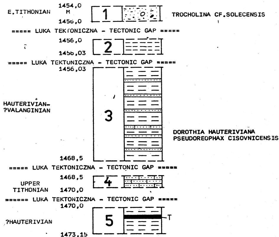
Fig. 4. Profil litostratigraficzny płaszczowiny śląskiej cieszyńskiej w otw. Łodygowice IG-1. 1 — łupki cieszyńskie dolne; 2 — margle pstre; 3 — łupki cieszyńskie górne; 4 — wapienie cieszyńskie; 5 — łupki cieszyńskie górne z cieszyńskim syłem (T)
