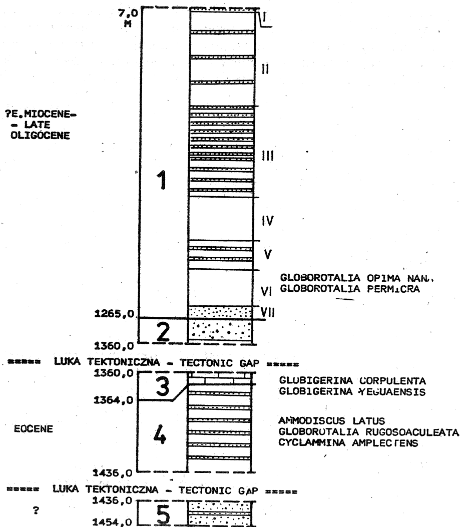
Fig. 3. Profil litostratigraficzny płaszczowiny śląskiej-godulskiej w otw. Łodygowice IG-1. 1 — warstwy krośnieńskie; I—VII — kompleksy litologiczne w obrębie warstw krośnieńskich; 2 — piaskowce gródeckie; 3 — margle globigerynowe; 4 — warstwy hieroglifowe; 5 — ?warstwy godulskie
