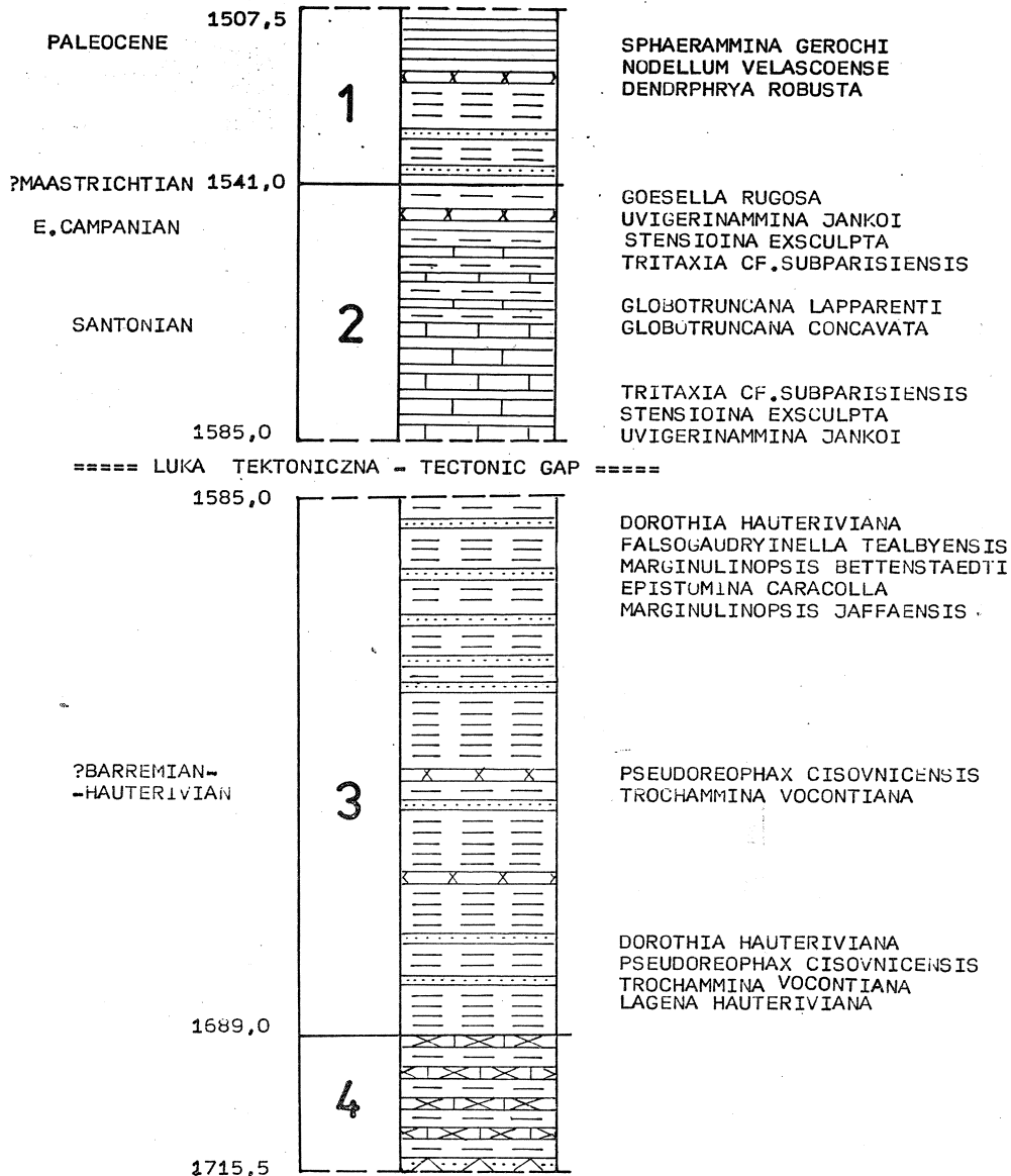
Fig. 6. Profil litostratigraficzny płaszczowiny podśląskiej w otw. Łodygowice IG-1. 1 — łupki szare; 2 — łupki zielone z wkładkami margli jasnozielonych; 3 — warstwy grodziskie łupkowe; 4 — warstwy gezowe dolne
