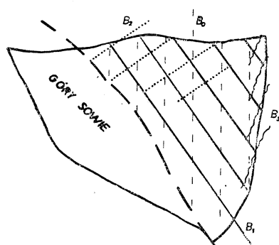
Fig. 1. Rozkład intensywności ruchów fałdowych B_0 , B_1 , B_2 i B_3 na obszarze przedgórskim bloku sowiogórskiego wg Grocholskiego (rysunek prezentowany na odczycie PTG we Wrocławiu w dniu 5. 12. 1968). B_0 — system reliktowy; B_1 — system najwyraźniejszy, fałdowanie główne o wergencji SW; B_2 — system rozwinięty głównie w N części bloku; B_3 — system rozwinięty tylko w części E bloku, w obrębie Wzgórz Gumińskich
