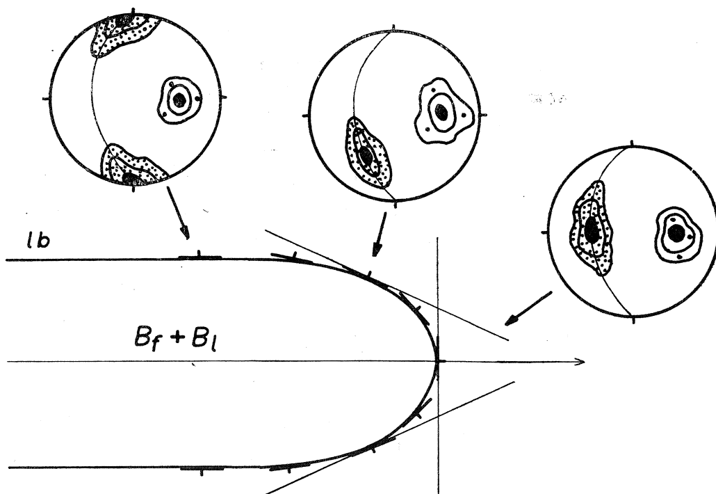
Fig. 6B — Mapa antykliny o osi wychylonej z położenia poziomego B_f + B_1 — oś fałdu + B — lineacja; l_b — linia biegu (poziomica foliacji). Na diagramach przedstawiono lineację (rzadka szrafura) i foliację (gęsta szrafura) w zależności od miejsca wykonywania pomiarów (wskazanych strzałkami)
