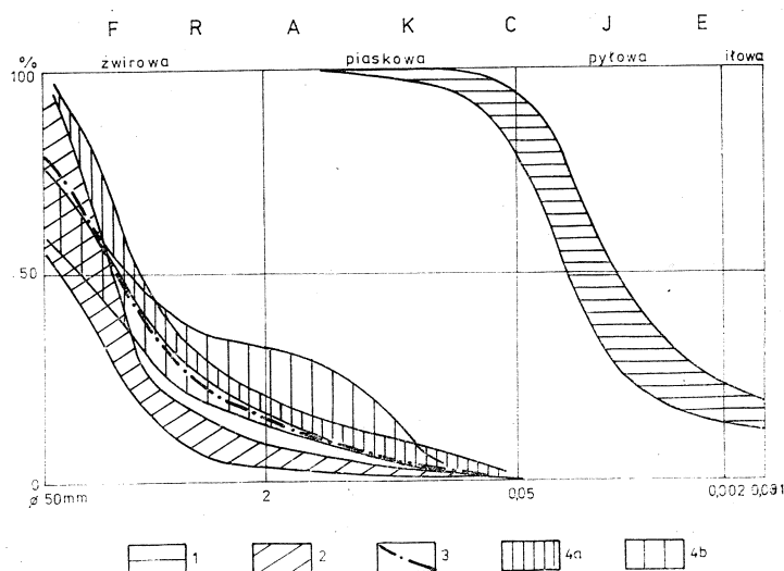
Fig. 7. Skład uziarnienia utworów plejstoceńskich. 1 — wykres przedziału składu ziarnowego lessów i utworów lessopodobnych; 2 — wykres przedziału składu ziarnowego osadów rzecznych z okresu zlodowacenia północnopolskiego (otwory OG-7 i OG-2); 3 — krzywa składu ziarnowego osadów rzecznych z okresu zlodowacenia środkowopolskiego (otwór OG-6); 4 — wykres przedziału składu ziarnowego osadów rzecznych z okresu zlodowacenia południowopolskiego: a — osady bez otoczek kwarcowych (otwory OG-4 i OG-5), b — osady z otoczkami kwarcu (otwór OG-10)
