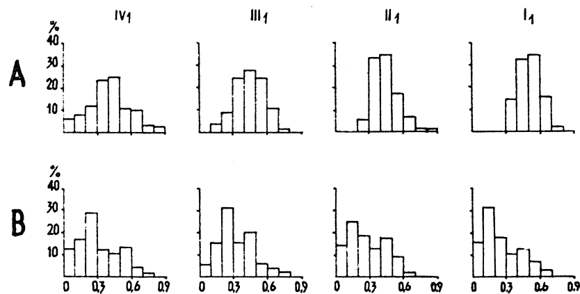
Fig. 8. Histogramy obtoczenia zespołu głazowo-żwirowego gliny zwałowej (II—IV) i bruku głazowego (I). A — materiał frakcji 10—4 mm; B — materiał frakcji 4—2 mm
