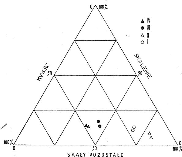
Fig. 6. Skład mineralno-petrograficzny frakcji 1—1,5 mm w projekcji trójkąta równobocznego. II—IV — poziomy gliny zwałowej; I — poziom bruku gładowego
