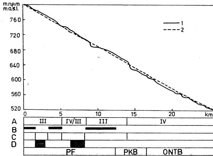
Fig. 6. Profil podłużny Białki. Objaśnienia — jak do ryc. 2, 4
