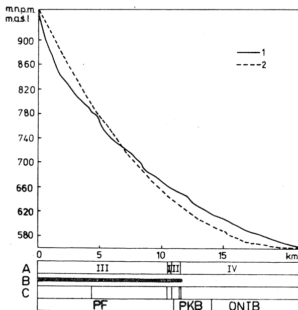
Fig. 5. Profil podłużny Leśnicy. Objaśnienia — jak do ryc. 2
