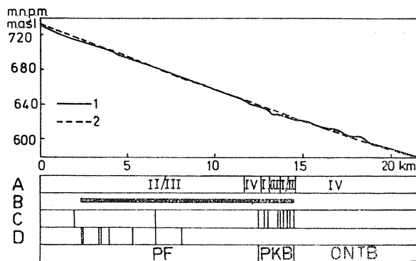
Fig. 4. Profil podłużny Białego Dunajca. D — rejon występowania osuwisk na zboczach doliny, pozostałe objaśnienia jak do ryc. 2 Fig. 4. Longitudinal profile of the stream Biały Dunajec. D — landslides zones, for other explanations — see fig. 2
