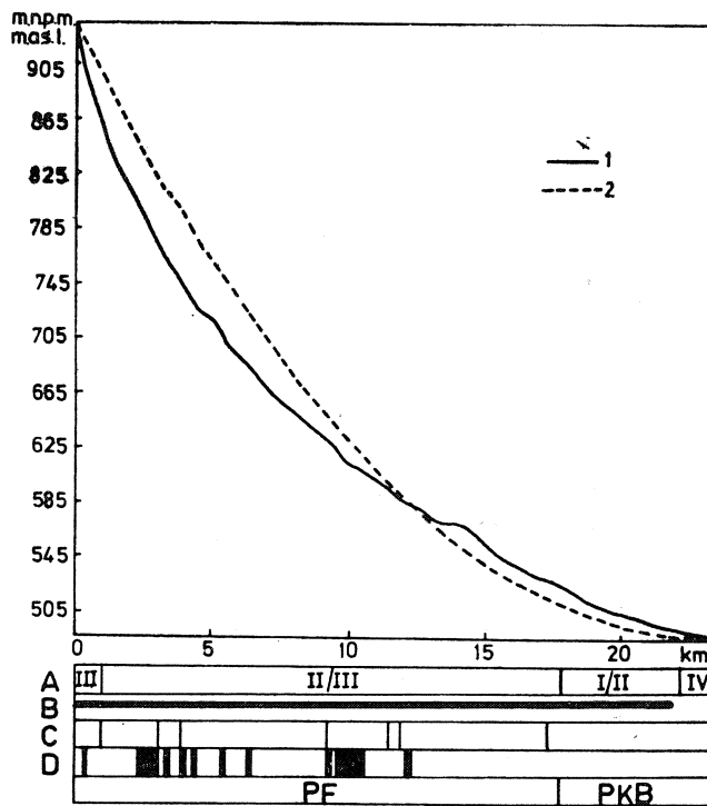
Fig. 7. Profil podłużny Łapszanki — Niedziczanki. Objaśnienia — jak do ryc. 2, 4
