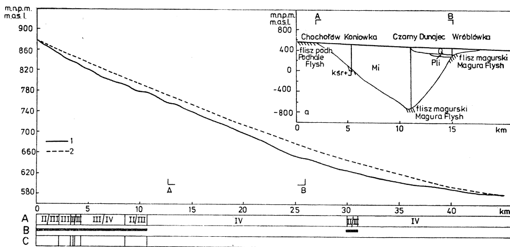
Fig. 2. Profil podłużny Czarnego Dunajca. 1 — linia profilu topograficznego; 2 — linia profilu równowagi obliczonego metodą Iwanowa. A — odporność skał podłoża: I—IV; B — wychodnie skał podłoża w korycie; C — ważniejsze strefy uskoko- we. PF — flisz podhalański; PKB — Pieniński Pas Skalkowy; ONTB — Kotlina Orawsko-Nowotarska
