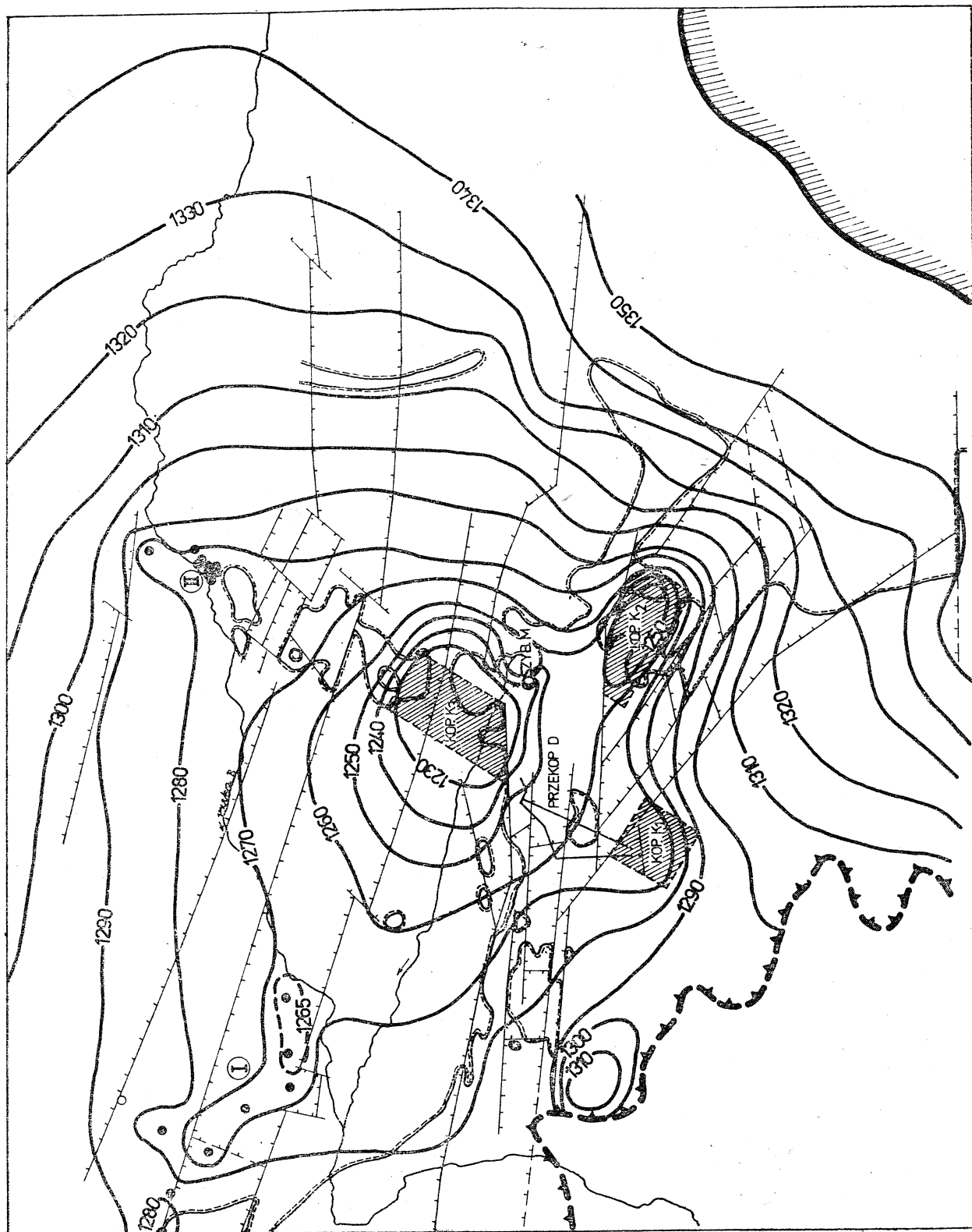
Fig. 8. Prognozowany układ pola hydrodynamicznego według stanu na 1. 04. 1985 dla I wariantu rozbudowy kopalni K 3 . Objaśnienia jak do fig. 2 i 5
