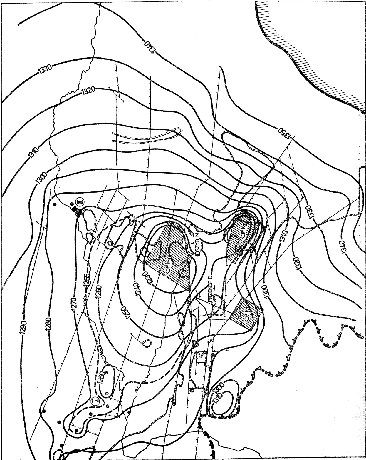
Fig. 7. Prognozowany układ pola hydrodynamicznego według stanu na 1. 04. 1980 dla I wariantu rozbudowy kopalni K 8 . Objaśnienia jak do fig. 2 i 5
