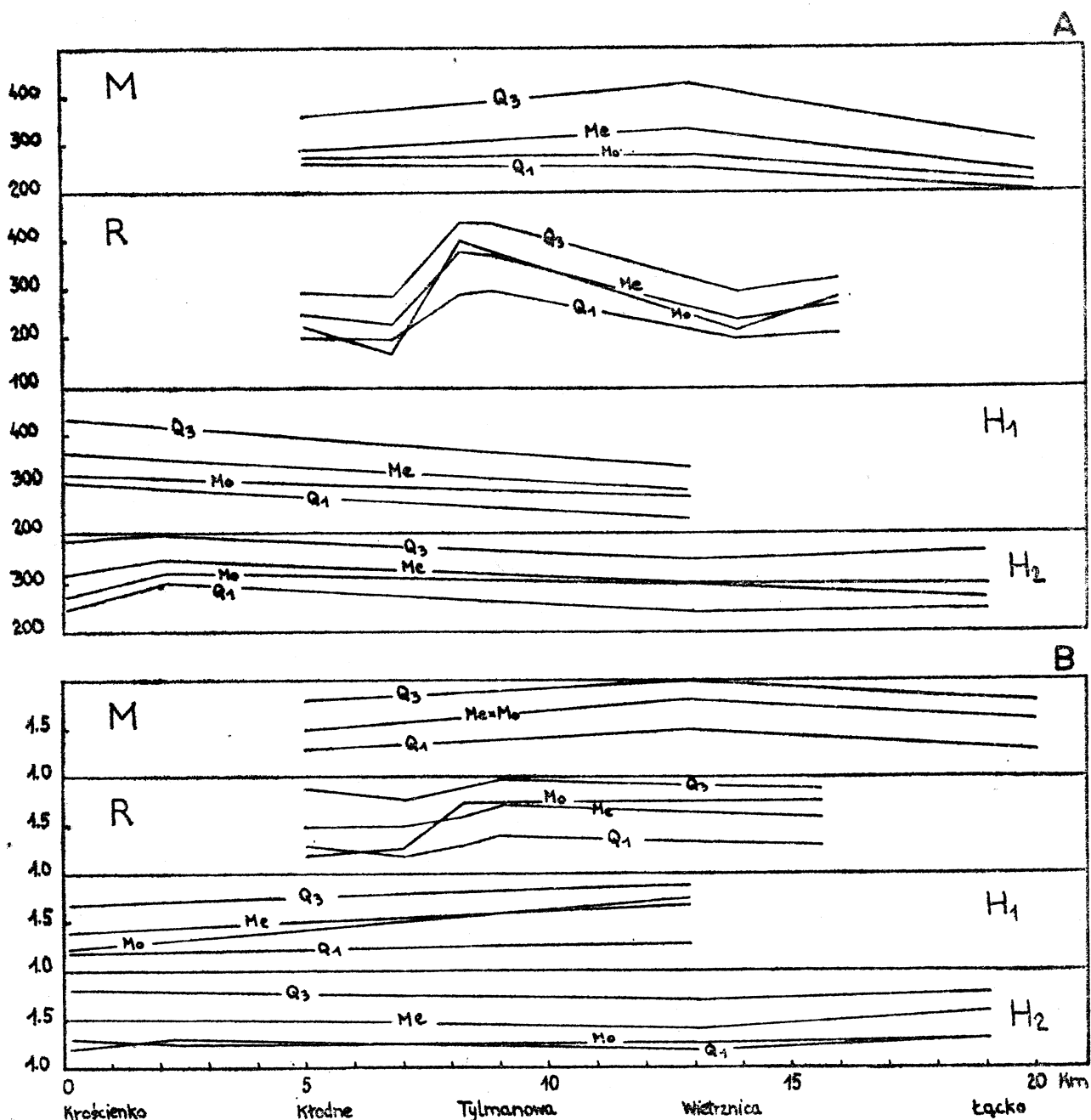
Fig. 4. Cechy morfoskopowe otoczków granitowych (4–6 cm średnicy) czwartorzędowych teras Dunajca (Krościenko — Łącko). A — współczynnik zaokrąglenia (wg Cailleux); B — współczynnik spłaszczenia (wg Cailleux); M — terasa ze zlodowacenia krakowskiego; R — terasa ze zlodowacenia środkowopolskiego; H 1 — terasa nadzalewowa; H 2 — kamieniec; Me — mediana; Q 1 — kwartyl pierwszy; Q 3 — kwartyl trzeci; Mo — wartość modalna
