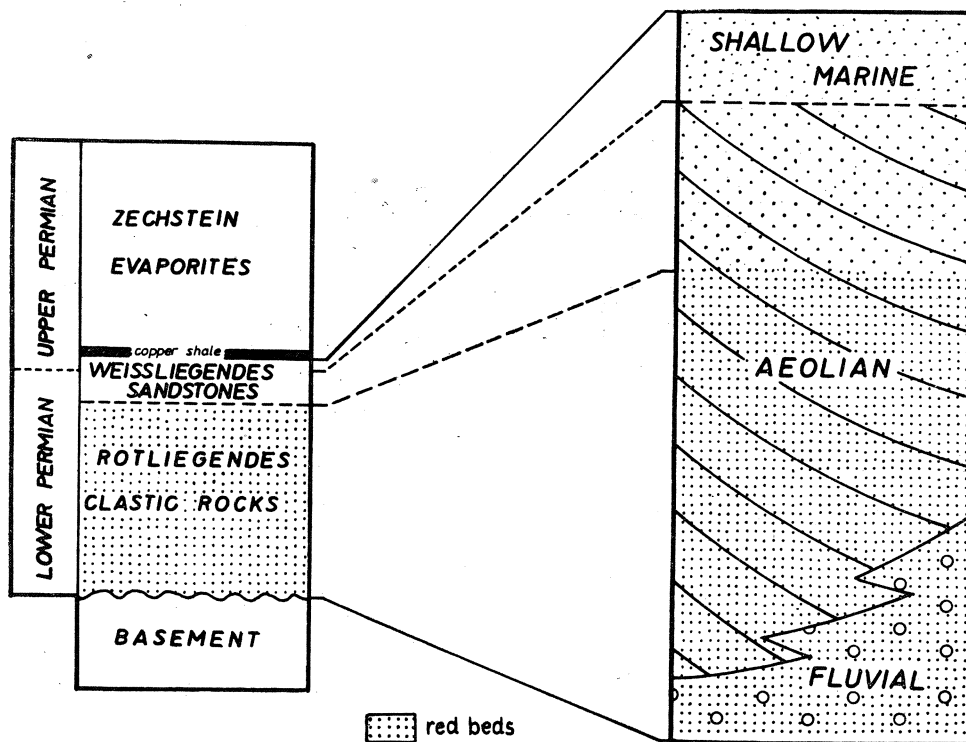
Fig. 1. General stratigraphy of the Permian, Fore-Sudetic Monocline; no scale Fig. 1. Zgeneralizowany profil stratygraficzny utworów permjskich monokliny przed-sudeckiej; bez skali
