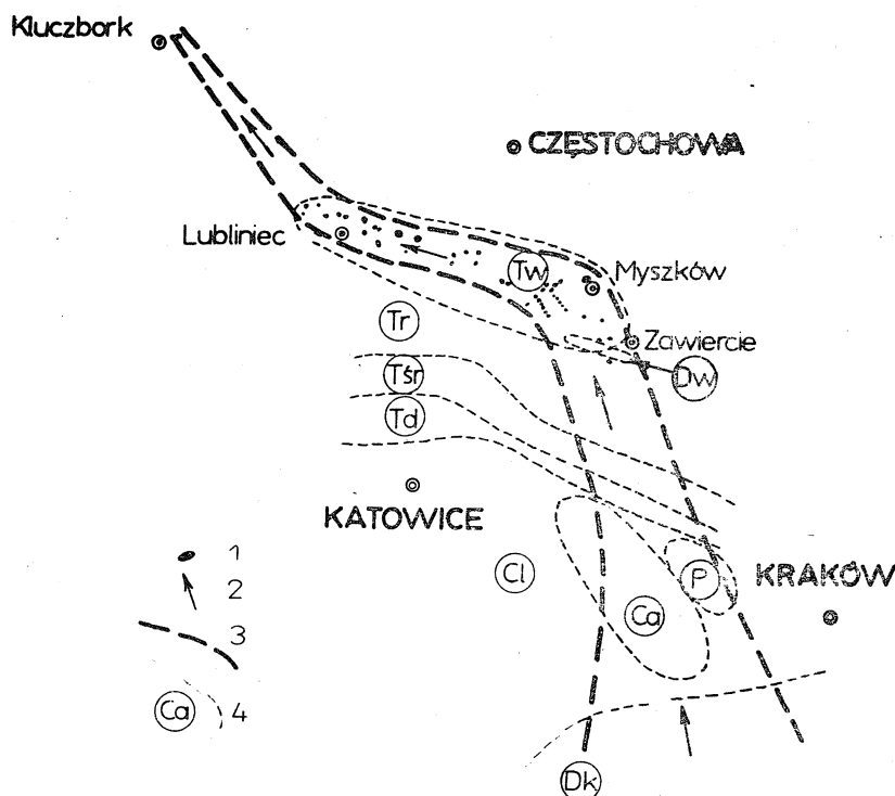
Fig. 5. Położenie obszarów źródłowych oraz doliny rzeki w górnym toarku. 1 — osady Formacji Połomskiej; 2 — kierunek transportu materiału; 3 — prawdopodobny obszar doliny rzecznej; 4 — prawdopodobne obszary źródłowe; Dk — zlepienie i piaskowce dewonu; Dw — wapienie dewonu; Cl — warstwy libiąskie (karbon); Ca — arkoza kwaczalska (karbon); P — permjskie skały wylewne; Td — zlepienie triasu dolnego; Tsr — wapienie triasu środkowego; Tr — pstre osady ilaste retyku; Tw — wapienie woźnickie
