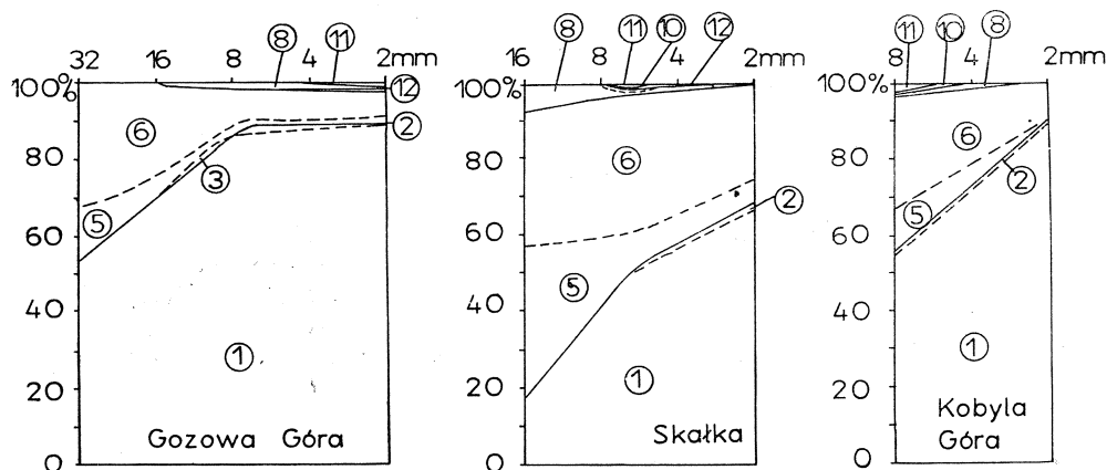
Fig. 3. Zmienność składu petrograficznego żwirów w procentach wagowych w zależności od uziarnienia, próby z warstw podwęglowych: 1 — kwarc mleczny; 2 — kwarc różowy; 3 — zlepienie; 5 — piaskowiec kwarcytowy; 6 — kwarcyt krystaliczny; 8 — skrzemionkowany wapień; 10 — piaskowiec arkozy; 11 — łupki kwarcytowy; 12 — rogowiec
