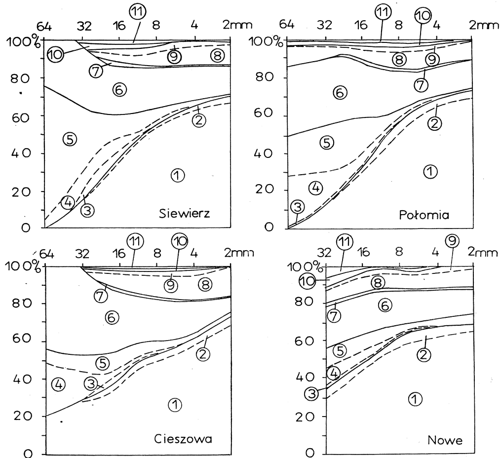
Fig. 4. Zmienność składu petrograficznego żwirów w procentach wagowych w zależności od uziarnienia, próby z formacji połomskiej (fm): 1 — kwarc mleczny; 2 — kwarc różowy; 3 — zlepienie; 4 — piaskowiec polimiktyczny; 5 — piaskowiec kwarcytowy; 6 — kwarcyt krystaliczny; 7 — jaspilit; 8 — wapień skrzemionkowy typu woźnickiego; 9 — skrzemionkowane wapień środkowotriasowe; 10 — piaskowiec arkozowy; 11 — inne skały
