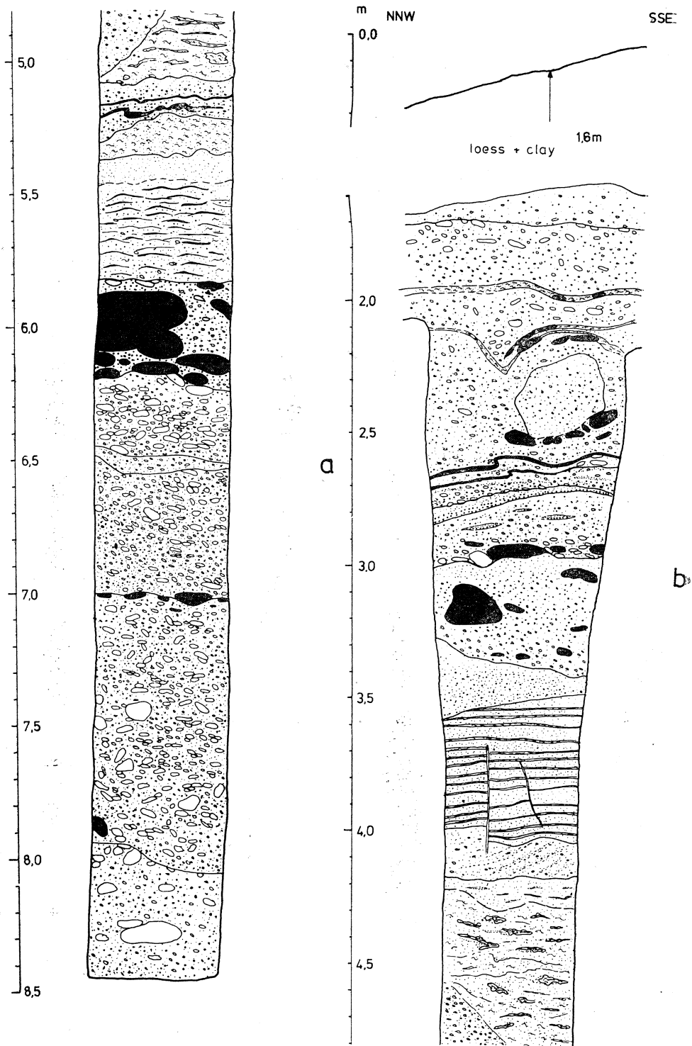
Fig. 14. Profil wkopu nr 10. Oznaczenia jak na fig. 3 Fig. 14. Drawing of excavation 10. Explanations — see Fig. 3
