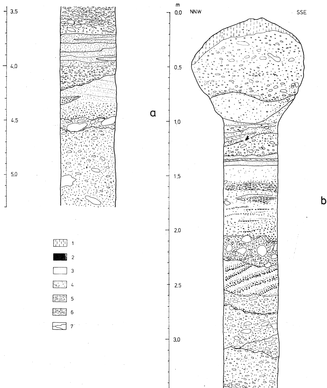
Fig. 3. Profil wkopu numer 11. a — niższa część wkopu, b — wyższa część wkopu; 1 — less, 2 — il; 3 — piasek zailony; 4 — piasek drobnoziarnisty; 5 — piasek ze żwirkiem; 6 — żwir średniotoczakowy; 7 — ostre granice warstw.
