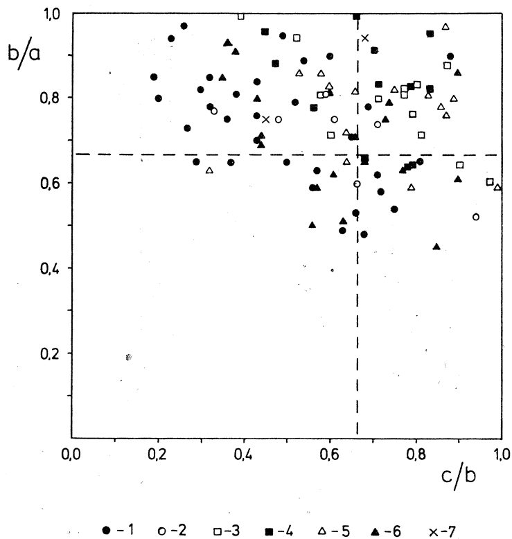
Fig. 8. Diagram kształtu otoczków (na podstawie 100 otoczków próba nr 2). 1 — piaskowce; 2 — kwarcyty; 3 — kwarc; 4 — skały krzemionkowe; 5 — wapienie; 6 — wapienie litotamniowe; 7 — skały inne
