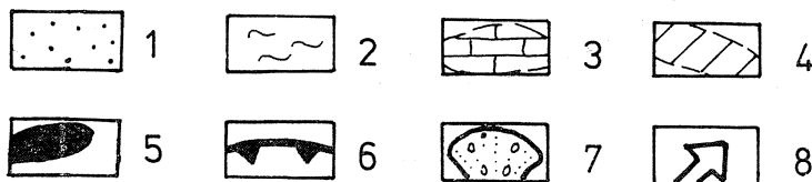
Fig. 17. Schemat drogi transportu materiału oraz obszaru depozycji osadów z Łek Górnych .1 — utwory fliszowe; 2 — drobnoziarniste osady miocenu; 3 — miocén- skie wapienie litotamniowe; 4 — obszar występowania warstw z egzotykami; 5 — skałka Podraza; 6 — brzeg Karpat; 7 — miocénskie osady gruboklastyczne; 8 — kierunek transportu
