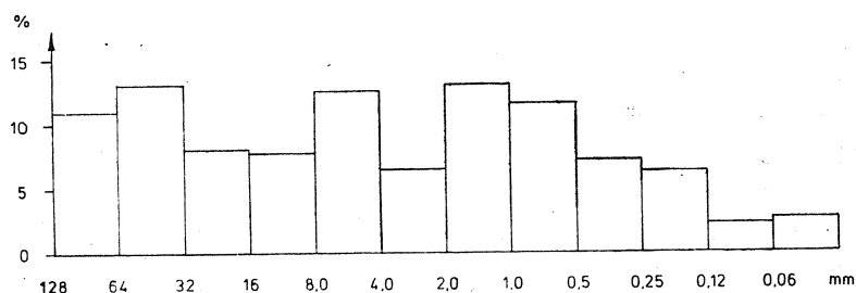
Fig. 5. Histogram uziarnienia osadu żwirowo-piaszczystego (próba nr 27) Fig. 5. Histogram showing grain-size distribution in sandy gravels (sample 27)
