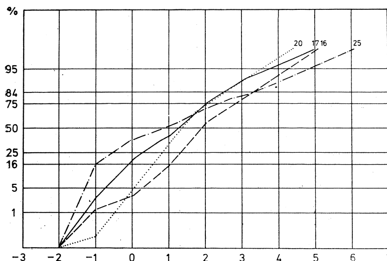
Fig. 7. Krzywe uziarnienia reprezentatywnych prób osadów piaszczystych (cyfry oznaczają numery prób)
