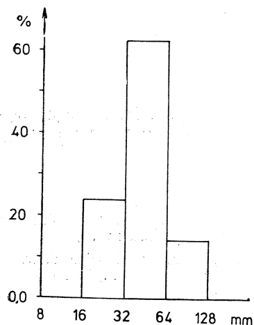
Fig. 6. Histogram uziarnienia otoczków wypreparowanych ze zlepieńców (300 szt., próba nr 1, 2 i 3)
