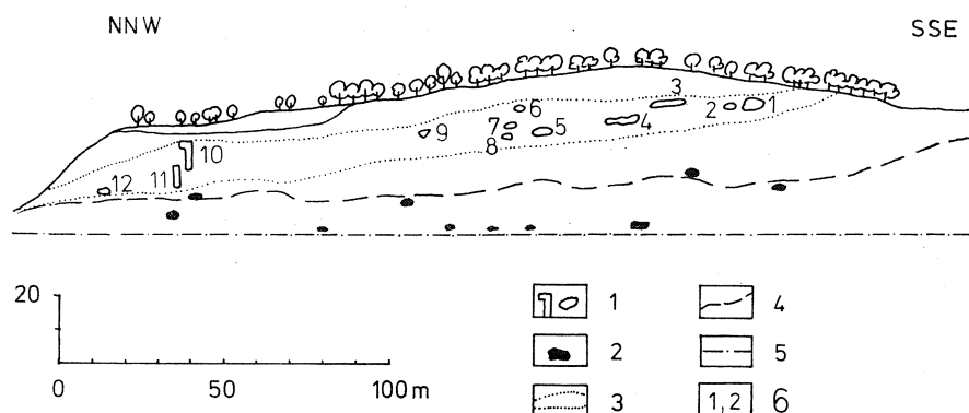
Fig. 2. Lokalizacja odsłonięć w „skałce Podraży”. 1 — odsłonięcia (wkopy) i ich orientacyjny kształt i wielkość; 2 — luźne bloki zlepieńców; 3 — zasięg występowania osadów żwirowych; 4 — droga; 5 — poziom potoku Dulcza; 6 — numery odsłonięć
