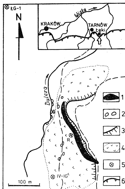
Fig. 1. Mapka sytuacyjna odsłonięcia w Łękach Górnych. 1 — zasięg występowania naturalnych odsłonięć osadów żwirowych; 2 — luźne przemieszczone bloki zlepieńców; 3 — skarpa „skałki Podraży”; 4 — osuwisko; 5 — otwory wiertnicze; 6 — brzeg Karpat
