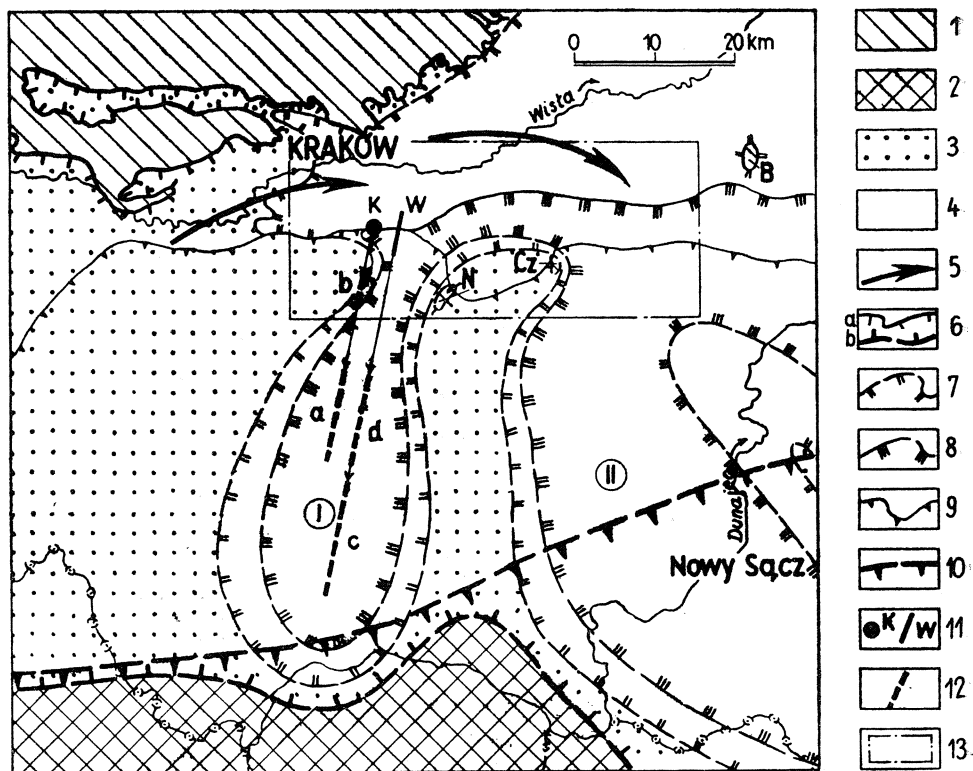
Fig. 2. Szkic paleogeograficzny badeńskiego zbiornika salinarnego na wschód od Krakowa. 1 — ład małopolski i wyspy przedgórzia Karpat stwierdzone wierceniami: N — Niżowej; Cz — Czyżyczki; B — Borzęcina; 2 — ład karpaccy; 3 — utwory dolnego badenu i klastyczne odpowiedniki ewaporatów; 4 — ewaporaty; 5 — kierunki dopływu wód do zatok salinarnych; 6 — zasięg utworów badenu (a — obecny, b — zrekonstruowany); 7 — przypuszczalny zasięg facji siarczanowej; 8 — przypuszczalny zasięg facji chlorkowej; 9 — dzisiejszy brzeg Karpat fliszowych; 10 — przypuszczalny brzeg Karpat fliszowych w badenie; 11 — stanowiska ewaporatów (K — otwór Krzyszkowice H2; W — przekrój przez złożę soli kamiennej w Wieliczce); 12 — przypuszczalne miejsce ewaporatów przed sfałdowaniem i przemieszczeniem (a — złoża soli kamiennej w Baryczu; b — gipsów elementu Krzyszkowic; c — bryłowego piętra złoża wielickiego; d — warstwowego piętra złoża wielickiego); 13 — obszar przedstawiony na fig. 1B. Elementy basenu salinarnego: I — zatoka barycko-wielicka; II — zatoka bocheńska
