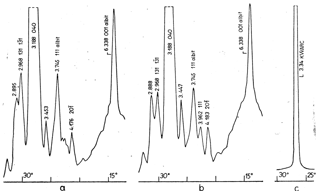
Fig. 6. Dyfraktogramy skaleni potasowych w przedziale 12—33° 2θ, Cu Kα: a — ska- leń potasowy pegmatytu z Lutonii; b — skał potasowy pegmatytu kordierytowe- go; c — kwarc
