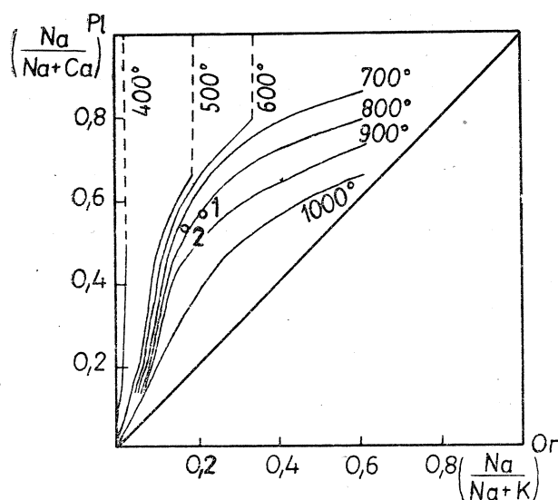
Fig. 2. Diagram równowagi fazowej w systemie plagioklaz (Pl) — skałen potasowy (Or), p = 1 kbar (wg Perczuka, Riabczikowa, 1968). 1 — skalenie z pegmatytu kordierytowego; 2 — skalenie z pegmatytu z Lutonii
