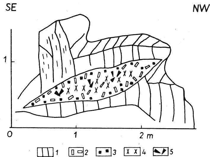
Fig. 1. Pegmatyt kordierytowy przecinający serpentynit (Lubachów); szkic odsłonięcia: 1 — serpentynit; 2 — nagromadzenia kordierytu, 3 — strefa wzbogacona w biotyt, 4 — strefy przerostów pismowych kwarcowo-skaliowych, 5 — skupienia turmalinu
