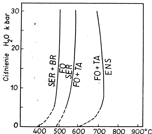
Fig. 4. Równowaga fazowa w systemie MgO-SiO_2-H_2O (wg Kitahara, Takenouchi, Kennedy, 1966 — fide Minerały, Sprawocznik , 1974). SER — serpentyn; FO — forsteryt; TA — talk; ENS — enstatyt
