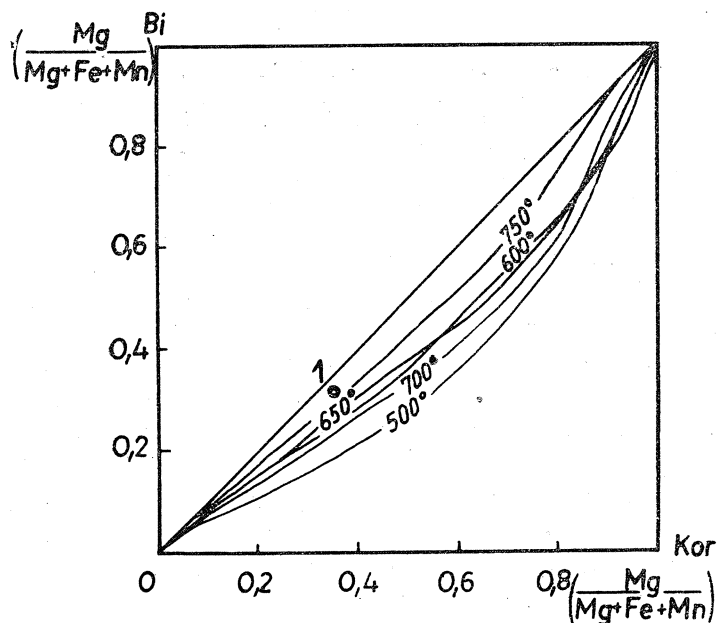
Fig. 3. Rozdział magnezu w asocjacji biotyt-kordieryt w zależności od temperatury (Perczuk, 1970): 1 — biotyt-kordieryt z pegmatytu kordierytowego (Lubachów)
