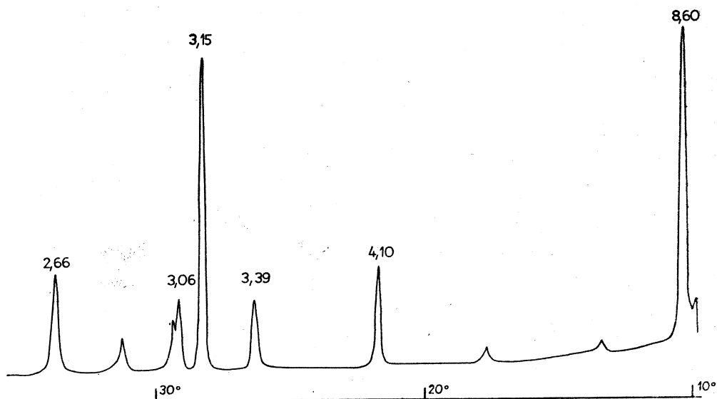
Fig. 5. Dyfraktogram kordierytu z pegmatytu w Lubachowie w przedziale 10—35° 2θ, Cu Kα.
