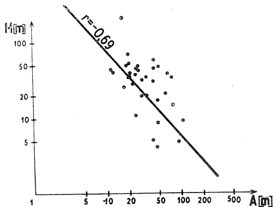
Fig. 7. Wykres zależności pomiędzy miąższością strefy aeracji (A) i miąższością osadów podanhydrytowych (M) dla centralnej części synklinorium miechowskiego.
