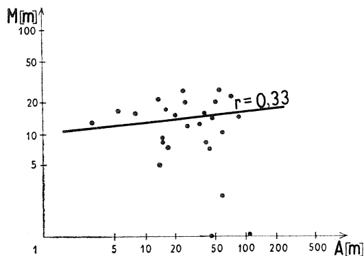
Fig. 8. Wykres zależności pomiędzy miąższością strefy aeracji (A) i miąższością osadów podanhydrytowych (M) dla rejonu Dąbrowy Tarnowskiej — Partyni-Podborza. Objąsnienia jak na fig. 5
