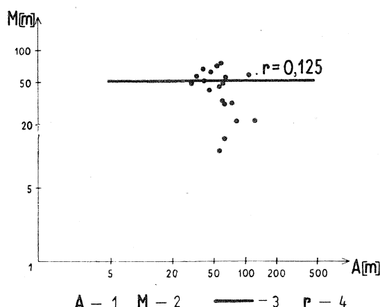
Fig. 5. Wykres zależności pomiędzy miąższością strefy aeracji (A) i miąższością osadów podanhydrytowych (M) dla obszaru położonego na wschód od Krakowa po Wyniesienie Puszczy: 1 — miąższość strefy aeracji w m; 2 — miąższość osadów podanhydrytowych w m; 3 — krzywa regresji; 4 — współczynnik korelacji
