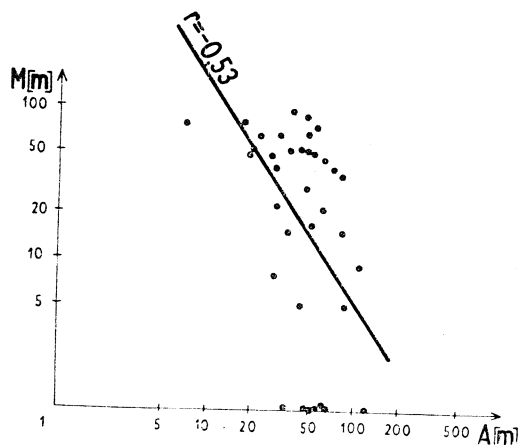
Fig. 9. Wykres zależności pomiędzy miąższością strefy aeracji (A) i miąższością osadów podanhydrytowych (M) dla peryferyjnej części zapadliska (na N od Wisły). Objaśnienia jak na fig. 5
