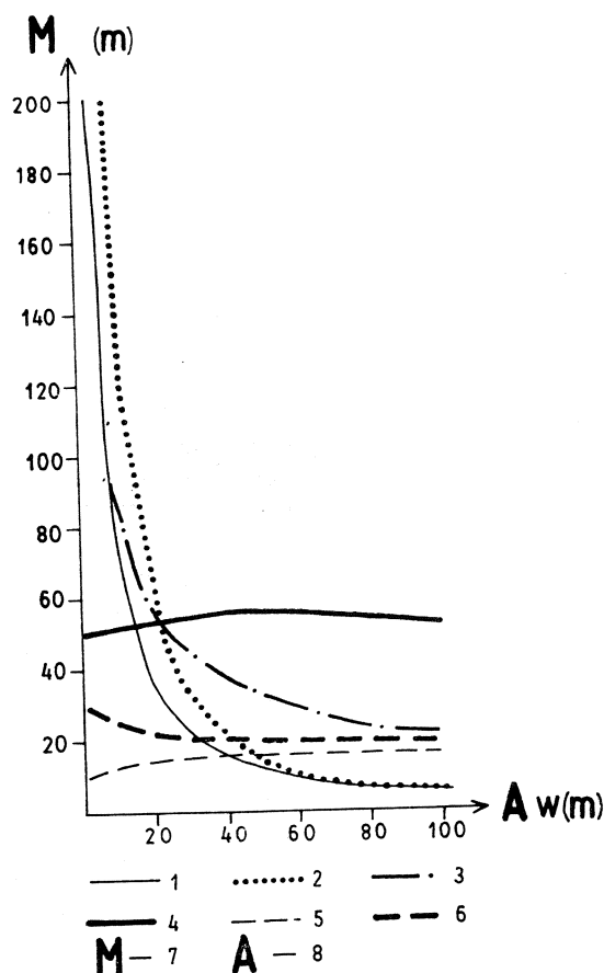
Fig. 11. Zestawienie zależności pomiędzy miąższością strefy aeracji (A) i miąższością osadów podanhydrytowych (M): 1 — centralna część synklinorium miechowskiego; 2 — peryferyjna część zapadliska (na N od Wisły); 3 — Wyniesienie Puszczy oraz rejon Grobla-Pławowice; 4 — Obszar na E od Krakowa po Wyniesienie Puszczy; 5 — Rejon Dąbrowy Tarnowskiej — Partyni Podborza; 6 — część zapadliska położona na S od Wisły
