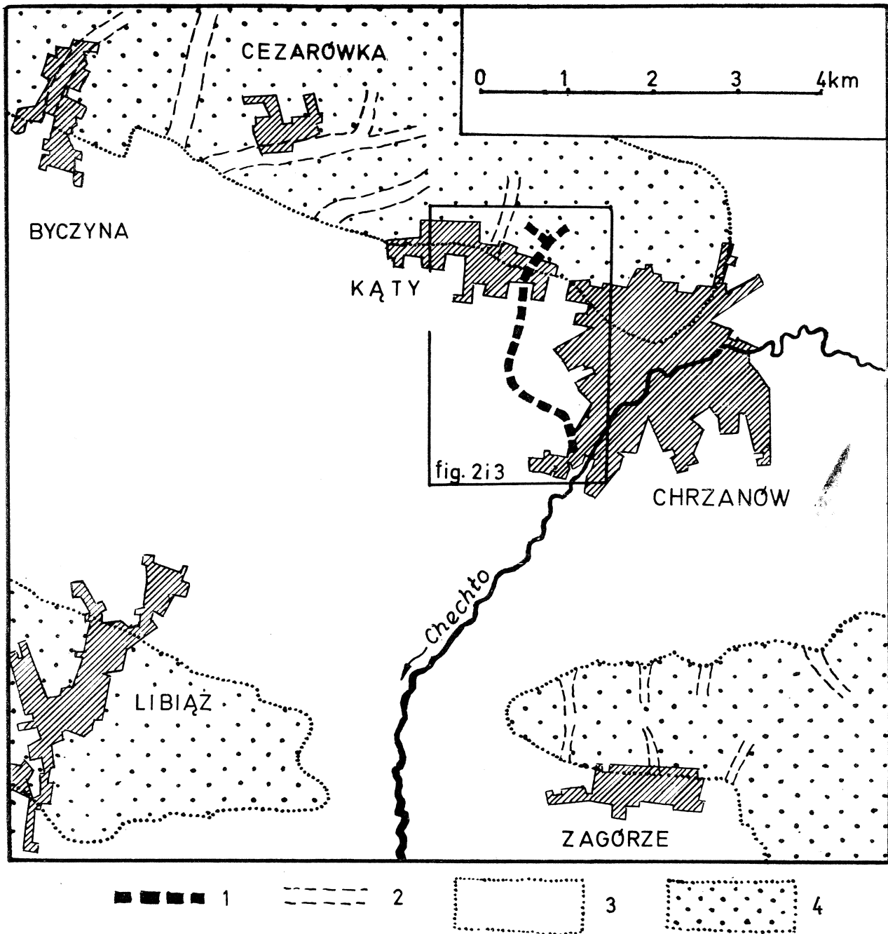
Fig. 1. Schematyczna mapa okolic Chrzanowa: 1 — kopalna dolina erozyjna, 2 — współczesne doliny erozyjne; 3 — utwory tortońskie; 4 — wychodne skał starszych od tortonu
