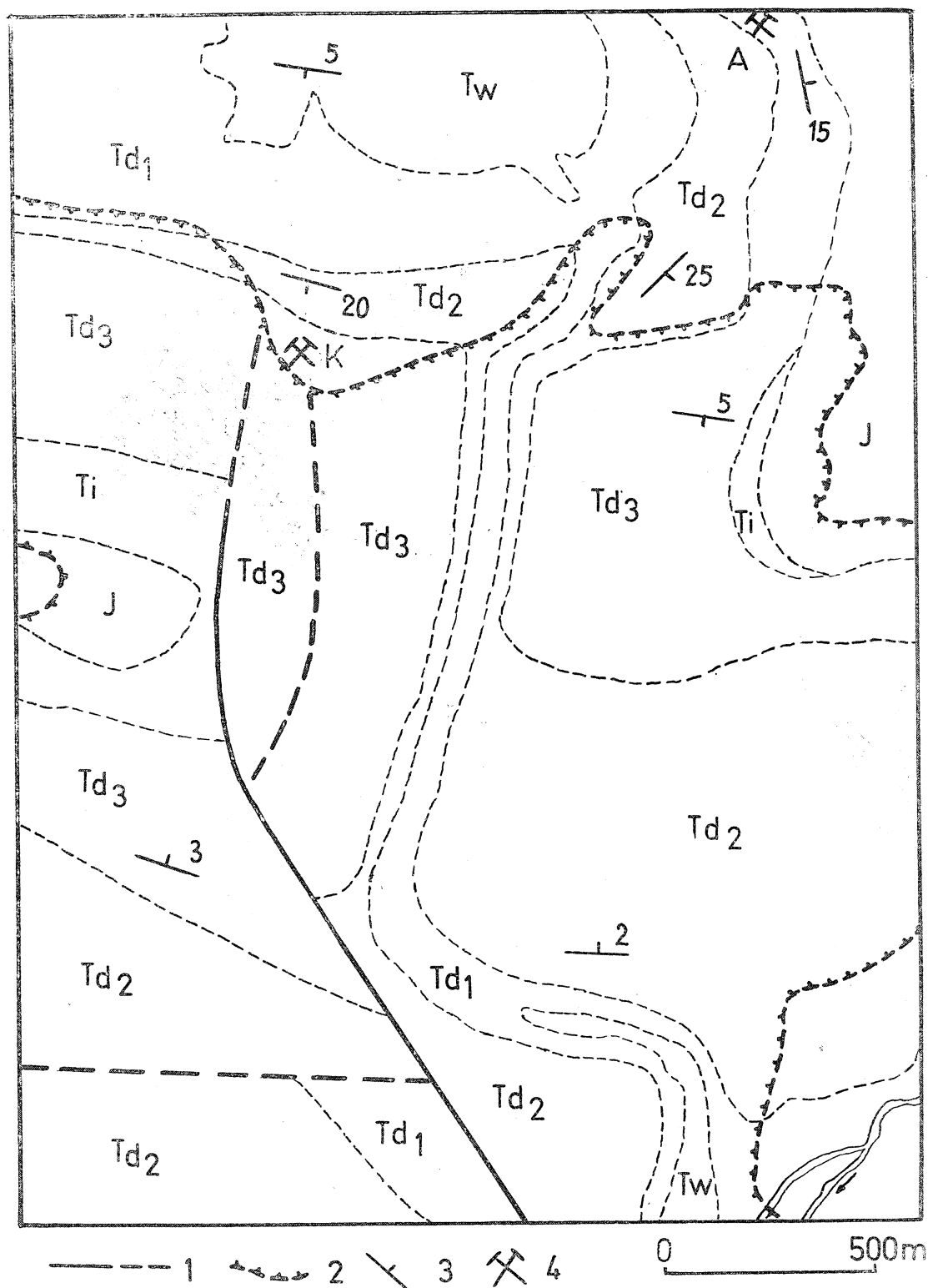
Fig. 2. Mapa geologiczna badanego obszaru: 1 — uskoki; 2 — zasięg utworów tortońskich; 3 — bieg i upad warstw triasowych; 4 — szyby kopaliń: K — Karol, A — Aleksander; skały starsze od tortonu: J — jura: wapienie i margle; T_i — kajper i warstwy boruszowickie: iłowce i mułowce; T_{d3} — warstwy tarnowskie: dolomity; T_{d2} — dolomity diploporowe; T_{d1} — dolomity kruszconośne; T_w — warstwy gogolińskie: wapienie i margle
