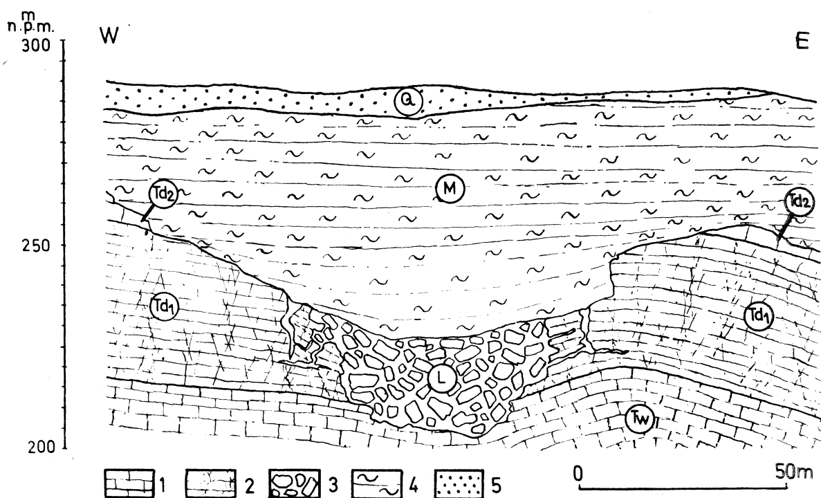
Fig. 4. Przekrój geologiczny przez kopalną dolinę erozyjną A—A': 1 — wapienie; 2 — dolomity; 3 — brekcje zawałowe; 4 — warstwowane ły i margle piaszczyste; 5 — piaski; Q — pleistocen; M — morskie utwory tortonu; L — lądowe utwory trzeciorzędowe; T d2 — dolomity diploporowe; T d1 — dolomity kruszconośne; T w — warstwy gogolińskie
