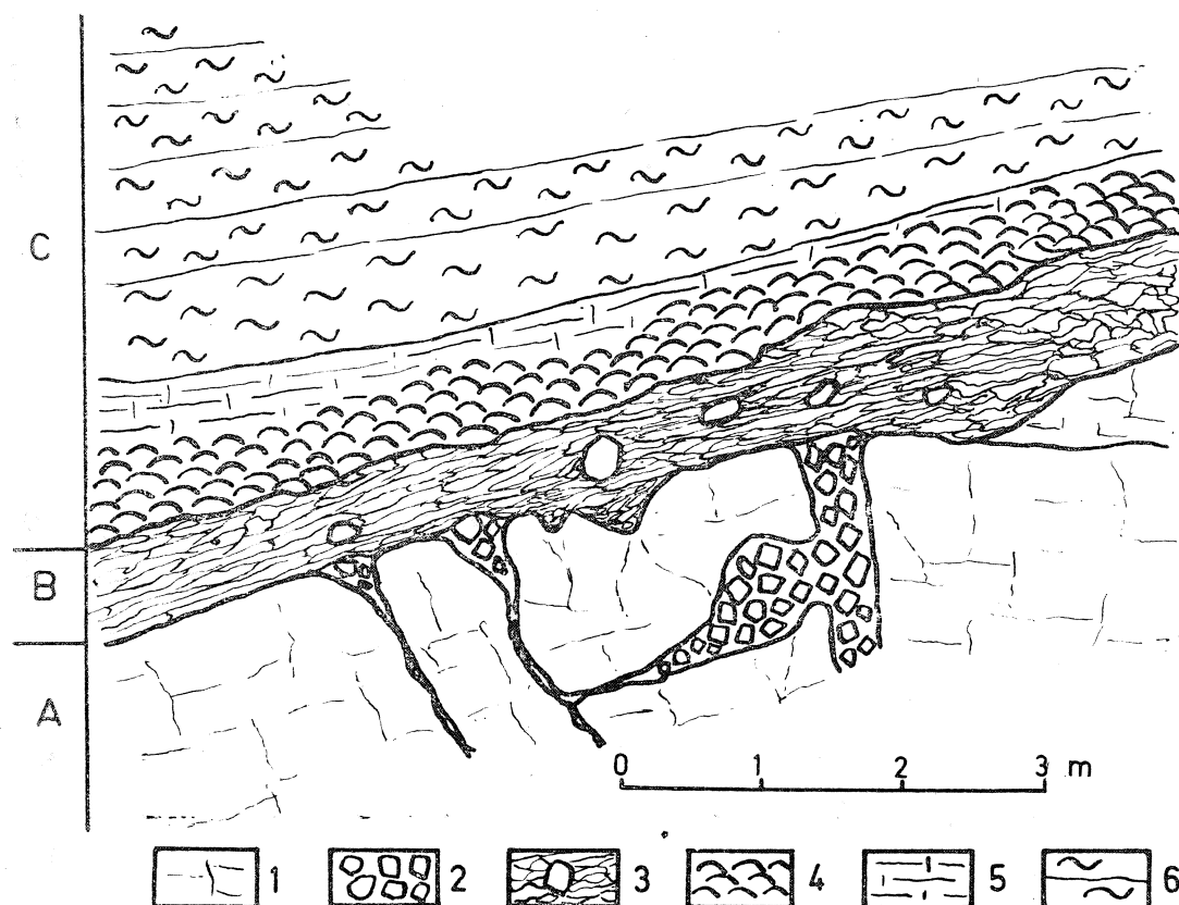
Fig. 15. Spągowa część morskich osadów tortonu: A — trias; B — torton (lądowy); C — torton (morski); 1 — dolomit; 2 — paleogeńskie gliny rezydualne; 3 — martenica wapienna; 4 — muszle ostryg; 5 — zielony il; 6 — piaszczyste margle
