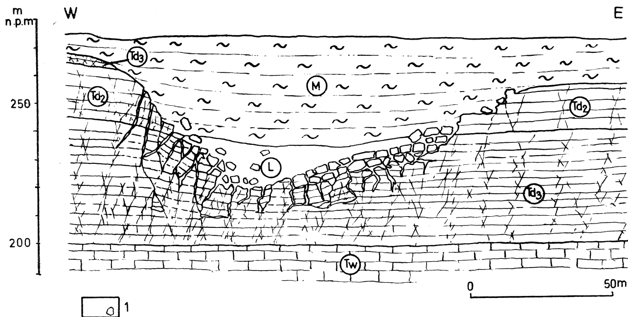
Fig. 5. Przekrój geologiczny przez kopalną dolinę erozyjną B—B': 1 — osady lądowe: piaski, iły i martwice wapienne; T d 3 — warstwy tarnowickie; pozostałe oznaczenia jak w objaśnieniach do fig. 4
