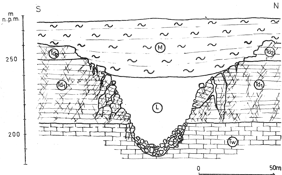
Fig. 7. Przekrój geologiczny przez kopalną dolinę erozyjną D—D': oznaczenia jak w objaśnieniach do fig. 4 i 5
