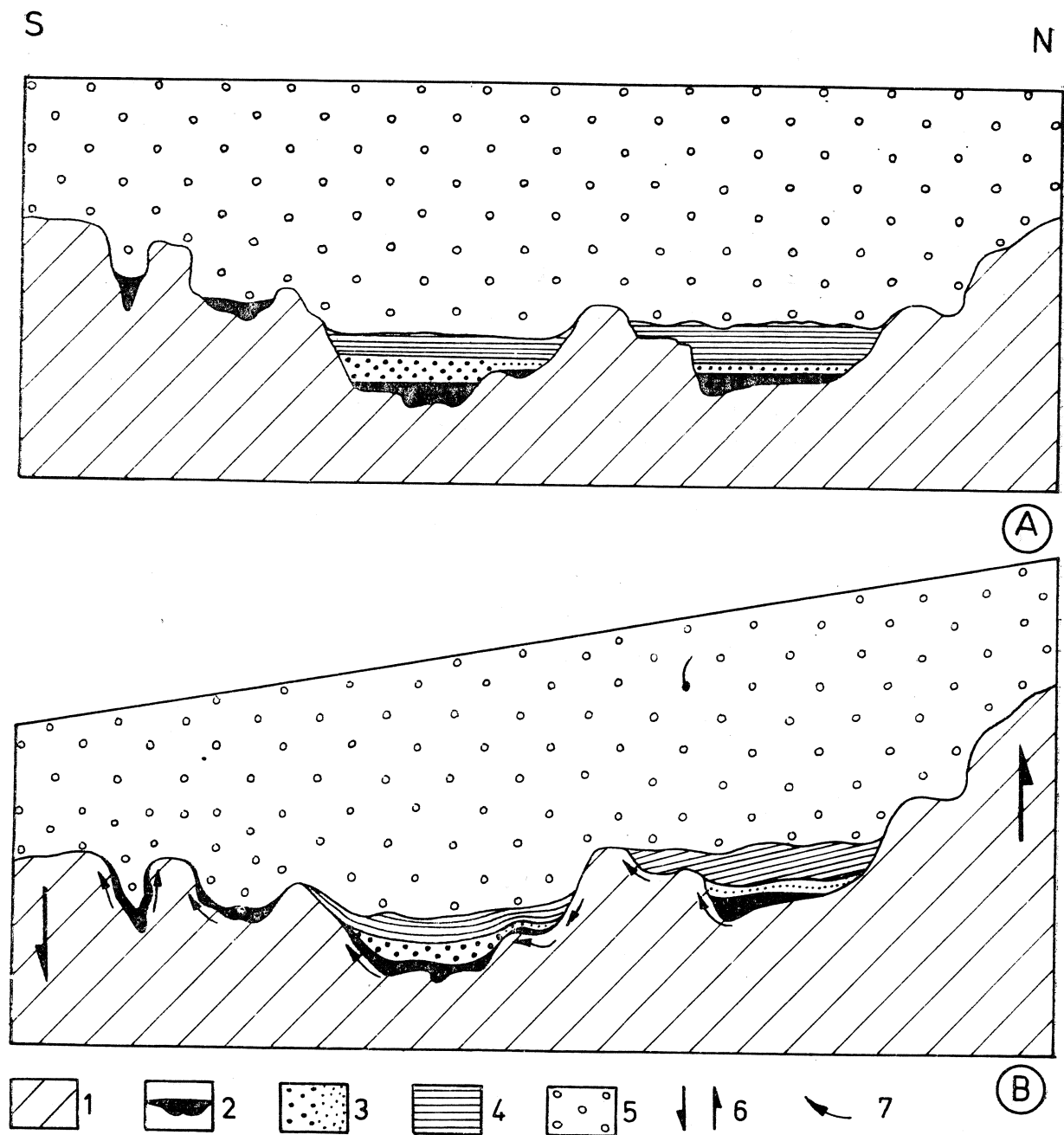
Fig. 7. Schemat powstania deformacji w osadach plejstocenijskich w Szaflarach. A — stadium przed deformacją (Mindel); B — stadium tworzenia się deformacji (Mindel-Riss) wskutek tektonicznego wychylenia skałki; 1 — biały wapień krynowidowy (bajos); 2 — regolit; 3 — przerobiony regolit i żwiry dolne; 4 — ił wstęgowy; 5 — żwiry górne; 6 — kierunki przemieszczeń tektonicznych skałki; 7 — kierunki spłyzywania osadu wskutek tektonicznego wychylenia skałki
