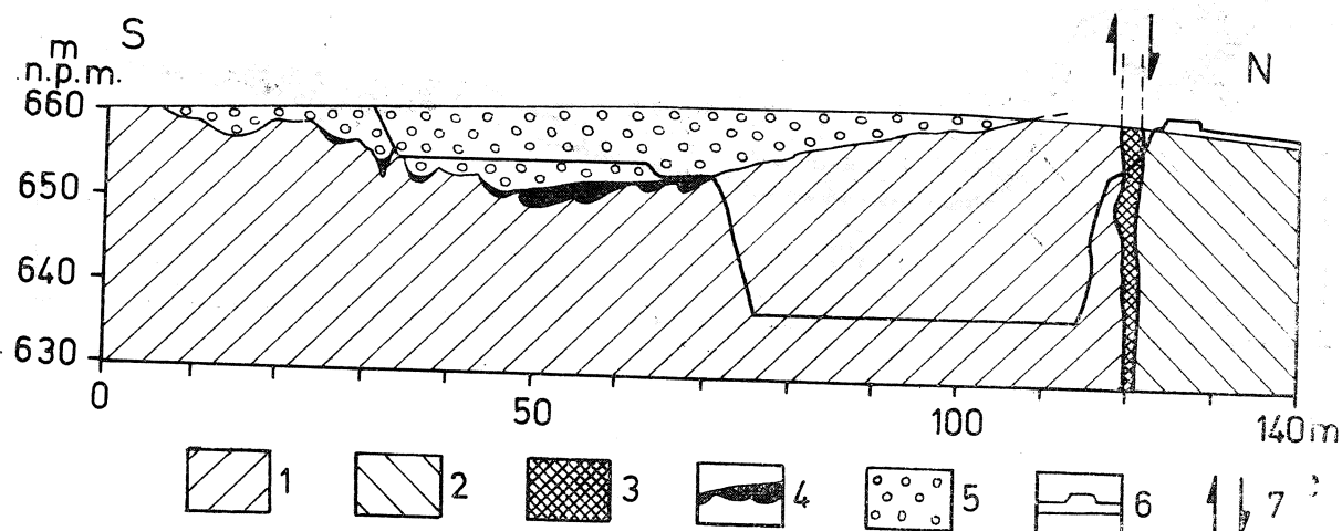
Fig. 6. Schematyczny przekrój geologiczny w południowo-zachodniej części kamieniołomu w Szaflarach. 1 — utwory jurajskie i kredowe jednostki czorsztyńskiej; 2 — utwory jurajskie i kredowe jednostki magurskiej; 3 — brekcja tektoniczna w strefie uskoku; 4 — utwory plejstocénskie starsze od pokrywy fluwioglacjału Mindel; 5 — pokrywa żwirowo-gliniasta fluwioglacjału Mindel; 6 — hałdy; 7 — kierunki przemieszczeń tektonicznych w plejstocenie
