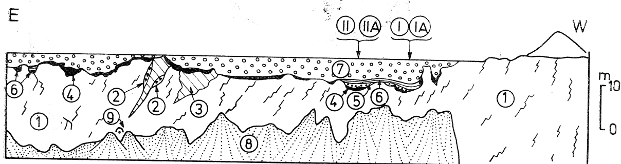
Fig. 3. Profil geologiczny południowej ściany kamieniołomu w Szaflarach z zaznaczoną lokalizacją profili I—II. 1 — biały krynoidowy (bajos); 2 — wapienne brekcje sedimentacyjne (tyton); 3 — czerwony muszlowiec (tyton); 4 — regolit i przerobiony regolit; 5 — żwiry dolne; 6 — ił wstęgowy; 7 — żwiry górne; 8 — usypisko
