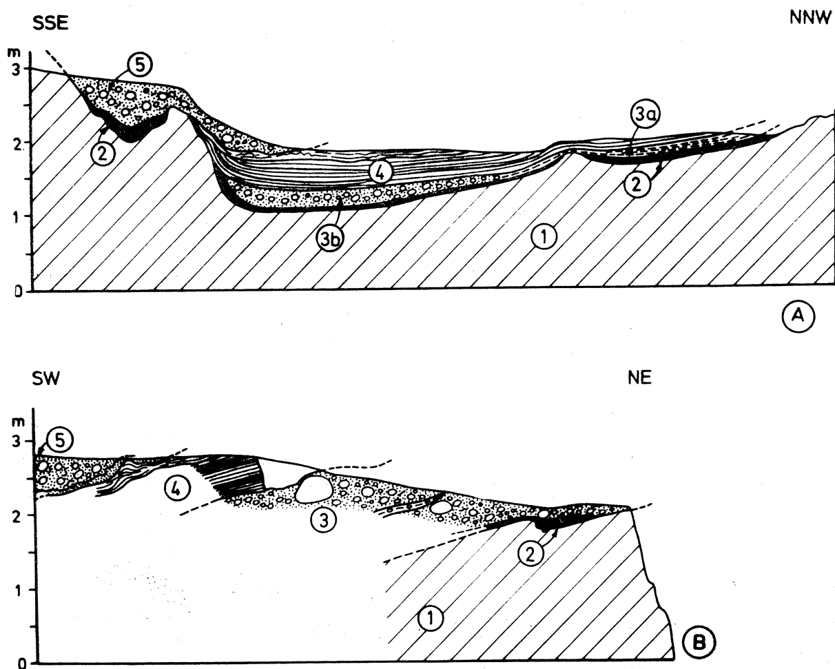
Fig. 5. Kamieniołom w Szaflarach, profile IIA (A) i II (B), stan z 1968 r. 1 — biały wapień krynowidowy (bajos); 2 — regolit; 3a — przerobiony regolit; 3b — żwiry dolne; 4 — ił wstęgowy; 5 — żwiry górne (Mindel) z warstwą piaszczystej gliny w spągu Fig. 5. Szaflary quarry, profiles IIA (A) and II (B), exposures in 1968. 1 — white crinoid limestone (Bajocian); 2 — regolith; 3a — reworked regolith; 3b — lower gravel; 4 — banded clay; 5 — upper gravel (Mindel) with sandy clay at the bottom
