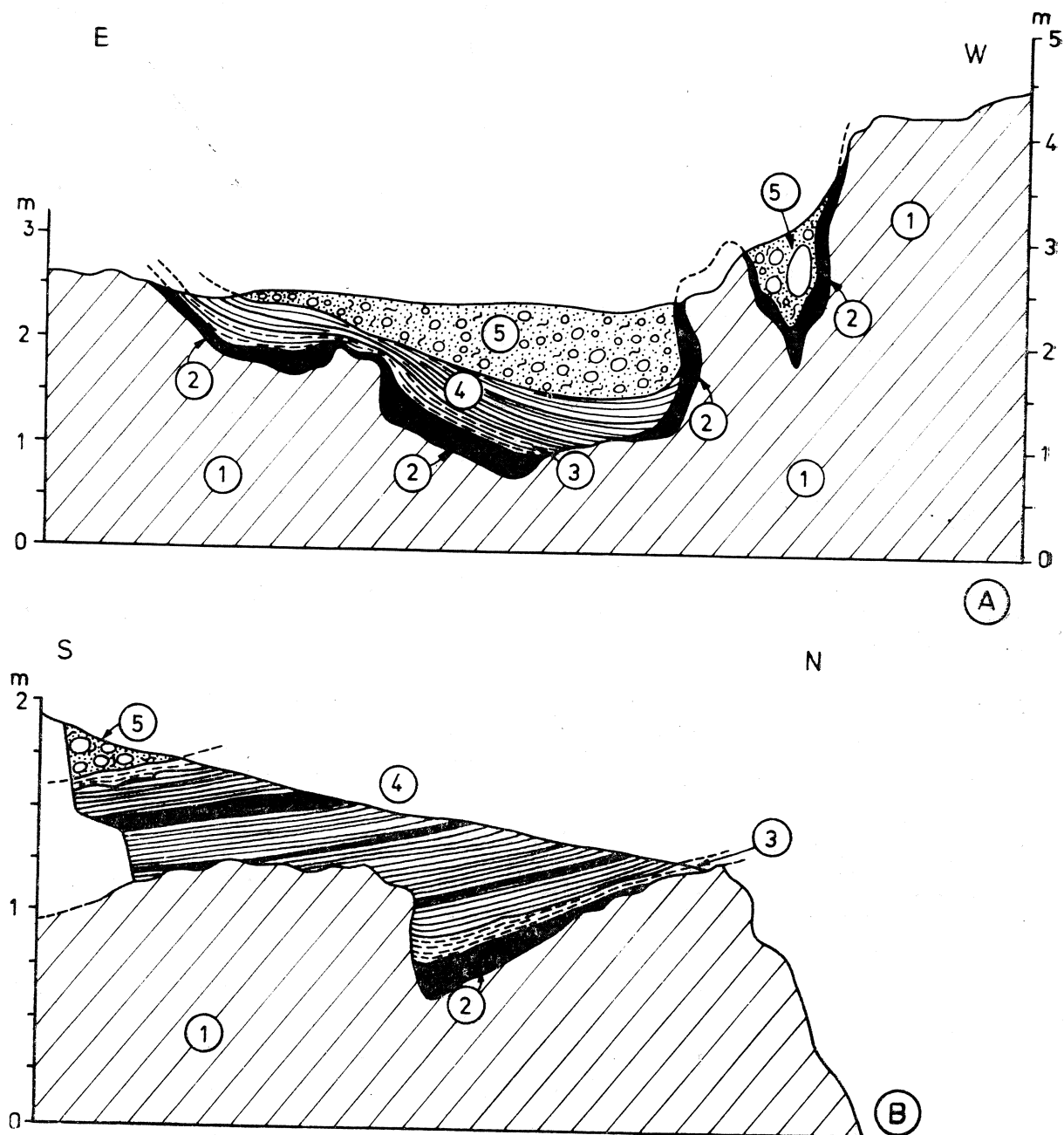
Fig. 4. Kamieniołom w Szaflarach, profile IA (A) i I (B), stan z 1968 r. 1 — biały wapień krynowidowy (bajos); 2 — regolit; 3 — przerobiony regolit; 4 — ił wstęgowy; 5 — żwiry górne (Mindel)
