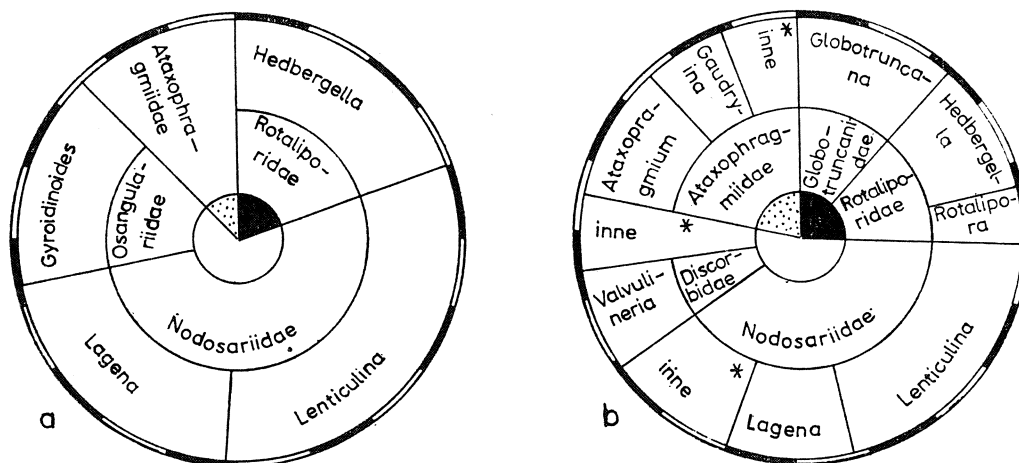
Fig. 10. Wykresy ilościowe składu zespołów otwornic z szarozielonych zapiaszczonych margli z glaukonitem (Kmg). a — część spągowa (uśredniona); b — część stropowa (uśredniona). W środkowym kole: pole czarne oznacza otwornice planktoniczne, pole białe — otwornice bentoniczne o skorupkach wapiennych, pole kropkowane — otwornice bentoniczne o skorupkach aglutynujących
