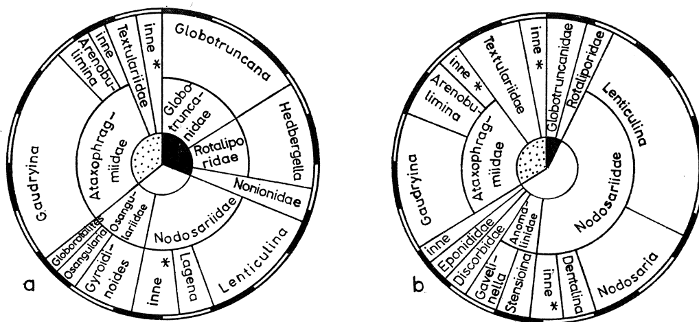
Fig. 15. Wykresy ilościowe składu zespołów otwornic z ciemnoszarych margli ilastych (Kmi 2 ). a — dolna część ogniwa (uśrednione); b — część przystopowa (uśrednione). Dalsze objaśnienia jak dla fig. 10
