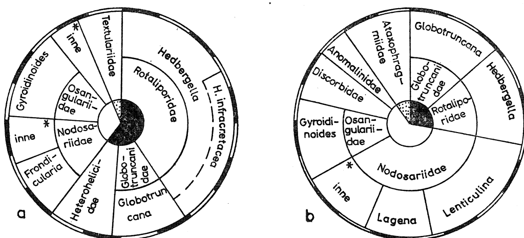
Fig. 11. Wykresy ilościowe składu zespołów otwornic z ciemnoszarych margli wapnistych (Km). a — część spągowa (anormalnie); b — część stropowa (uśrednione). Dalsze objaśnienia jak dla fig. 10
