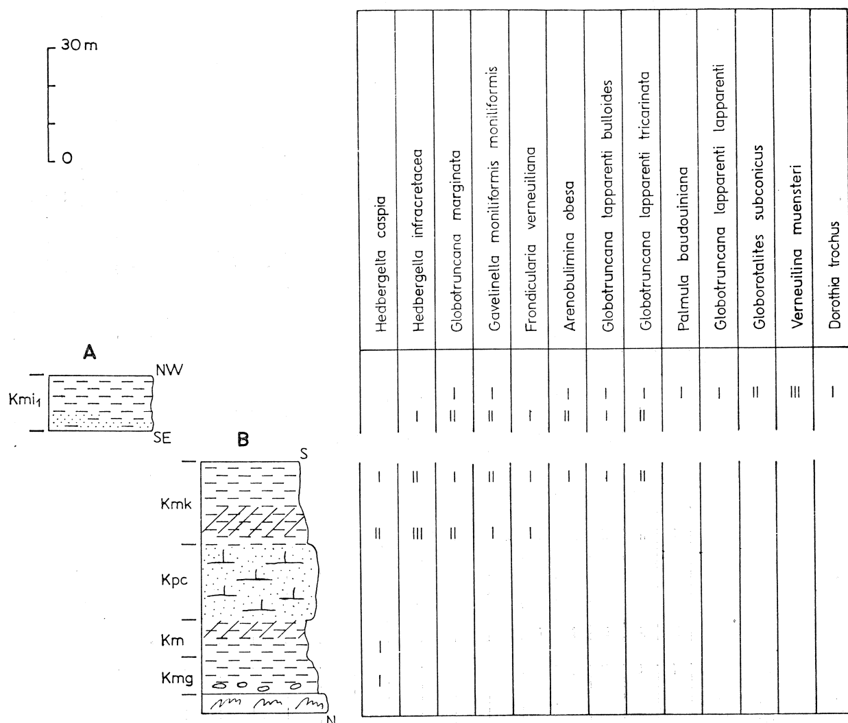
Fig. 8. Profil VI: A — odsłonięcie w Starym Waliszowie, B — odsłonięcie we wsi Mielnik. Opis warstw w tekście
