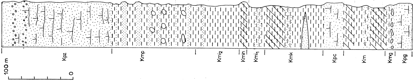
Fig. 18. Rozmieszczenie makro- i mikrofauny w profilu litostratygraficznym górnej kredy z rowu Nysy. a — 1—6 okazów w próbie; b — 7—16 okazów w próbie; c — więcej niż 16 okazów w próbie
