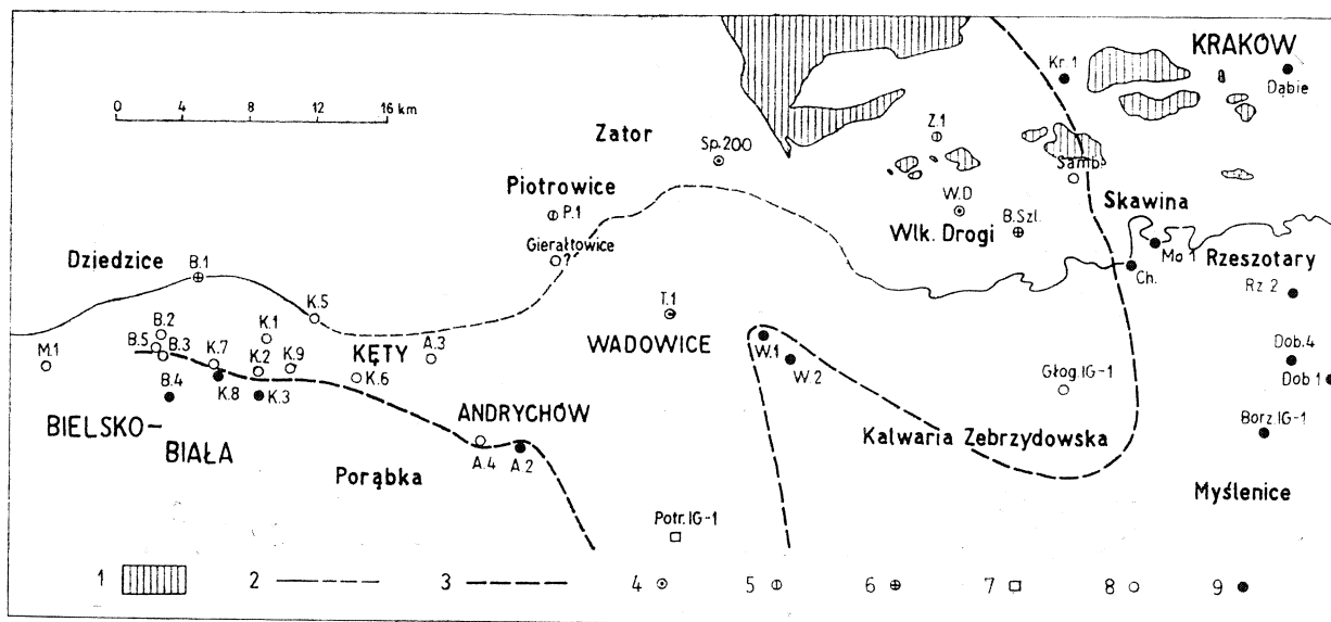
Fig. 1. Szkic sytuacyjny ważniejszych wierceń w obszarze Bielsko — Kraków. 1 — utwory mezozoiczne na powierzchni; 2 — północny brzeg fliszowych Karpat, miejscami z miocenem parautochtonicznym; 3 — przypuszczalna granica zasięgu warstw brzeżnych a równocześnie Górnośląskiego Zagłębia Węglowego; 4 — otwory, które nawierciły w stropie karbonu produktywnego warstwy libiąskie s. 1.; 5 — otwory, które nawierciły w stropie karbonu produktywnego warstwy łaziskie s. 1.; 6 — otwory, które nawierciły w stropie karbonu produktywnego warstwy orzeskie s. 1.; 7 — otwory, które nawierciły w stropie karbonu produktywnego warstwy siódłowe (?); 8 — otwory, które nawierciły w stropie karbonu produktywnego warstwy brzeżne; 9 — otwory, które nawierciły karbon dolny i utwory starsze
