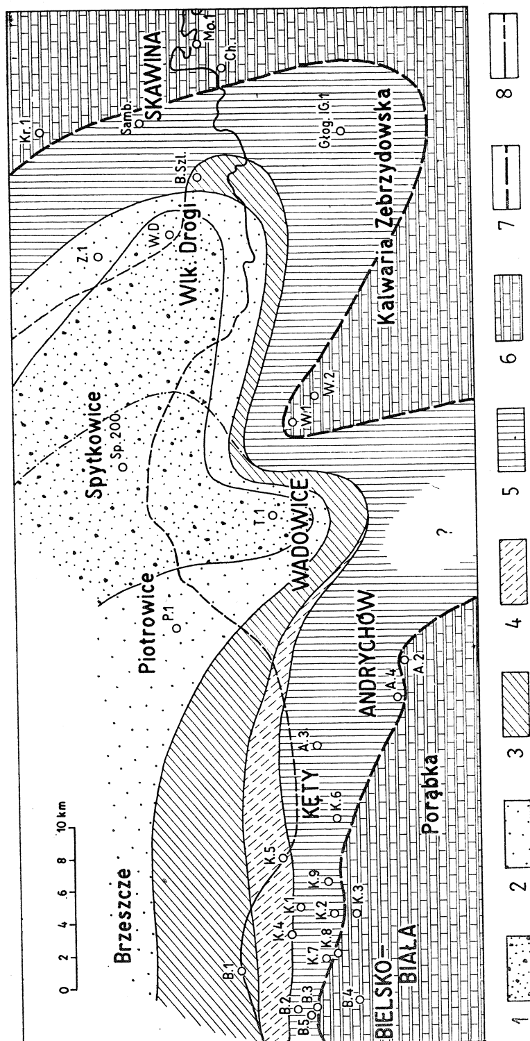
Fig. 5. Szkic geologiczny południowo-wschodniej części Górnośląskiego Zagłębia Węglowego w rejonie Bielsko — Skawina. 1 — warstwy libiąskie; 2 — warstwy łaziskie; 3 — warstwy orzeskie; 4 — warstwy rudzkie; 5 — warstwy brzeźne; 6 — karbon dolny, dewon i utwory starsze; 7 — przypuszczalna południowa granica Górnośląskiego Zagłębia Węglowego w świetle dotychczasowych wierceń i prac geofizycznych; 8 — północny brzeg utworów fliszowych Karpat, miejscami z mioceniem parautochtonicznym. Objaśnienie nazw wierceń jak w fig. 1
