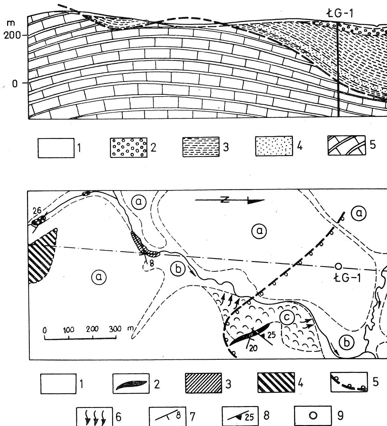
Fig. 6. Szkic geologiczny i przekrój przez okolice odwiertu Łęki Górne 1. Przekrój: 1 — czwartorzęd; 2 — sarmat (?); 3—4 — baden: 3 — iłolupki; 4 — piaski; 5 — warstwy inoceramowe (łupki ilaste i piaskowce).
