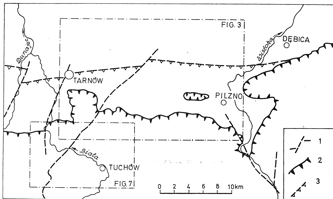
Fig. 1. Sytuacja geologiczna omawianych obszarów. 1 — uskoki; 2 — brzeg Karpat fliszowych; 3 — czoło nasunięcia utworów miocenyjskich
