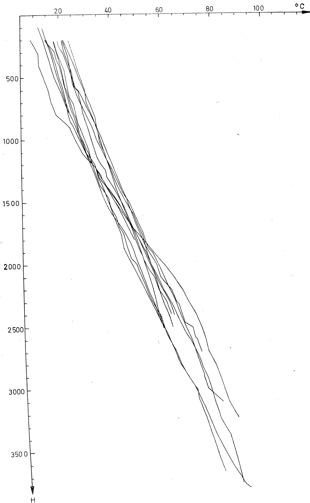
Fig. 4. Geotermogramy z obszaru póln-wschodniej Polski
