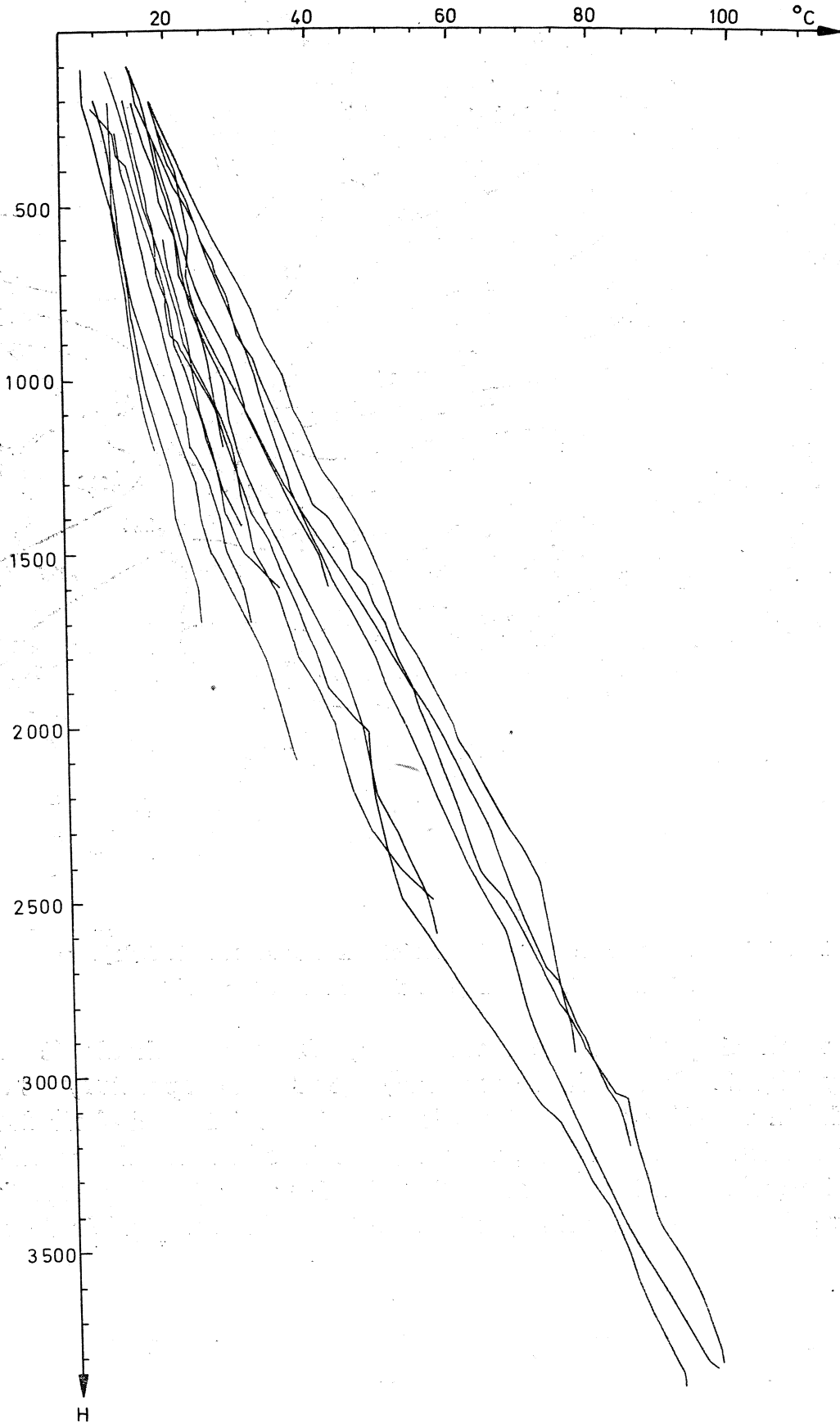
Fig. 3. Geotermogramy z obszaru na pół-wschód od linii Teisseyre'a
