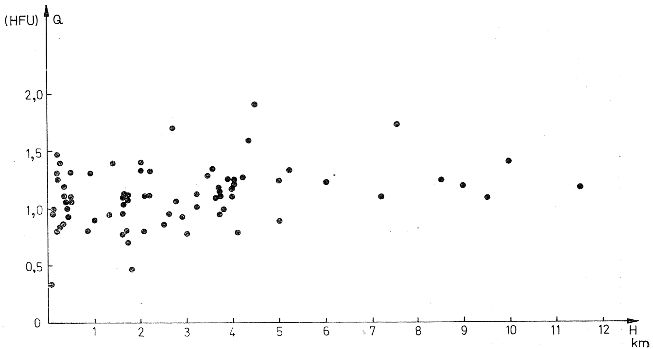
Fig. 6. Zależność strumienia ciepłego od miąższości piętra osadowego w obszarach platformowych
