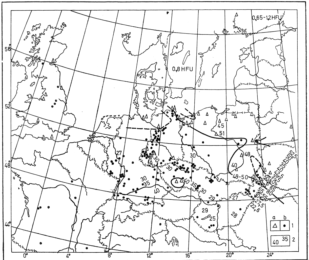
Fig. 9. Strumień ciepły w Europie centralnej. 1 a — wartości Q \leq 1,30 ; 1 b — wartości Q > 1,30 ; 2 — głębokości „Moho” (według pracy pod redakcją Sollogub, Prossen, Miltzer, 1971)
