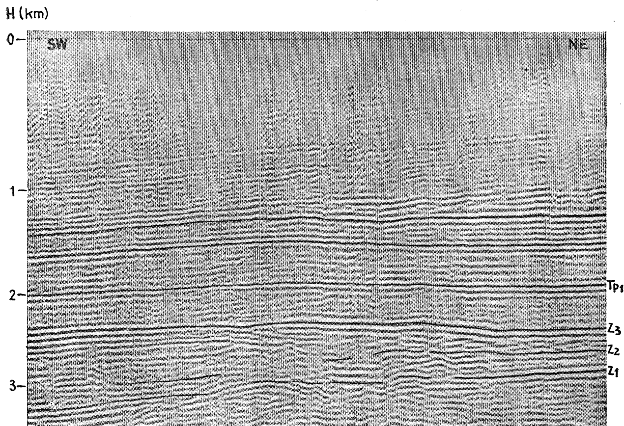
Fig. 6. Czasowy przekrój sejsmiczny 46-V-70T z rejonu Rekowa. Nieciągłości w korelacji granic refleksyjnych Z_1 i Z_2 spowodowane blokową budową. Objaśnienia przy fig. 3
