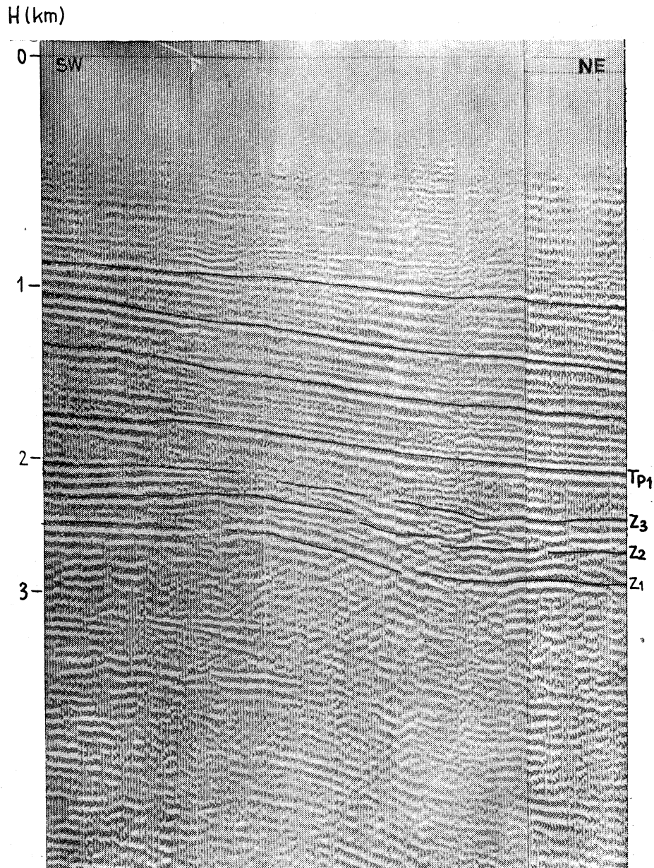
Fig. 7. Czasowy przekrój sejsmiczny 41-V-70T z rejonu Kamienia Pomorskiego, przedstawiający budowę blokową kompleksu permian. Antyklina w środkowej części zdjęcia bardzo przypomina zapis na profilach sejsmicznych z rejonu rafy Babimostu. Objasnienia przy fig. 3
