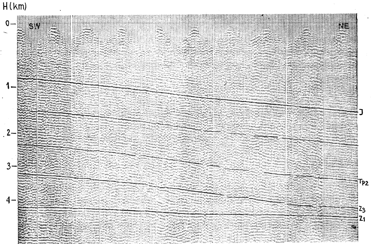
Fig. 5. Czasowy przekrój sejsmiczny 16-XIII-70T z rejonu Chabowa. Widoczna typowa dla głębszych partii basenu ceechsztyńskiego niezgodność zalegania między refleksyjną granicą podsolną Z_1 a granicami młodszymi. Objasnienia przy fig. 3
