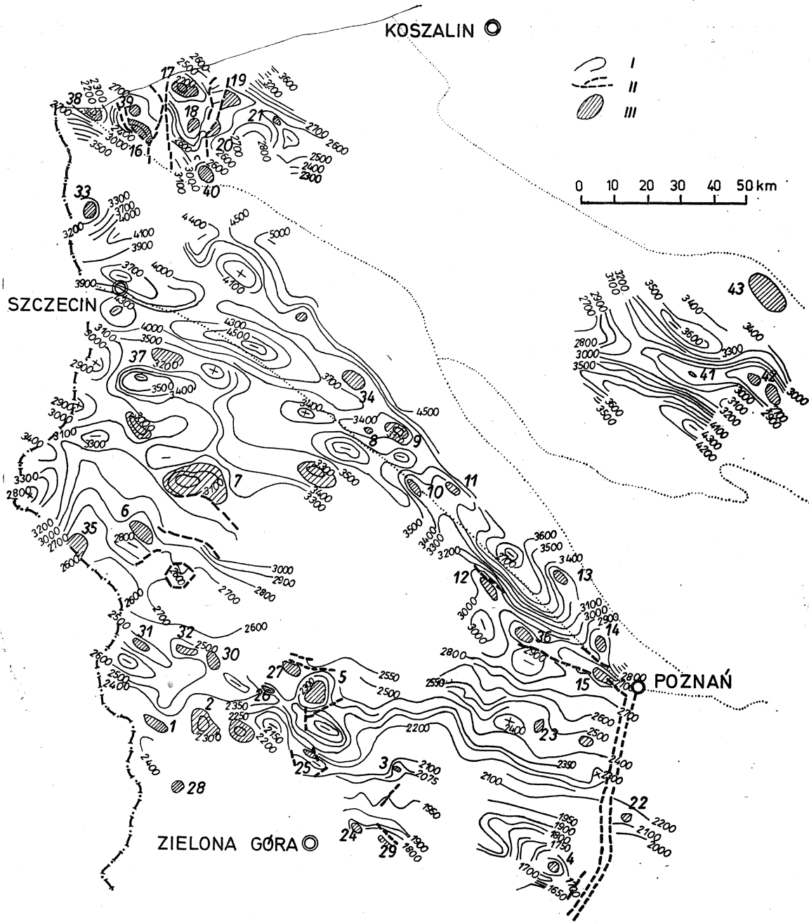
Fig. 2. Mapa głębokościowa cechszyńskiej granicy refleksyjnej Z_3 w zachodniej Polsce. (Topography of the reflection boundary Z_3 in Western Poland). I — izobaty granicy refleksyjnej Z_3 (isobaths); II — uskoki (faults); III — obiekty strukturalne rozpoznane zdjęciem powierzchniowym (tectonic structures): Struktury lokalne (tectonic structures): 1 — Cybinka; 2 — Gądków; 3 — Babimost; 4 — Zakowo; 5 — Staropole; 6 — Dębno; 7 — Myślibórz; 8 — Pławno; 9 — Radęcin; 10 — Drawiny; 11 — Huta Szklana; 12 — Chrzypsko; 13 — Obrzycko; 14 — Rokienica; 15 — Bytyń; 16 — Dargobądz; 17 — Kamień Pomorski; 18 — Rekowo; 19 — Świeržno; 20 — Benice; 21 — Gryfice. Podniesienia lokalne (elevations): 22 — Donatowo; 23 — Buk; 24 — Klenica; 25 — Radoszyn; 26 — Łągów; 27 — Wielowieś; 28 — Maszewo; 29 — Bojadła; 30 — Smogóry; 31 — Górzycza; 32 — Ośno; 33 — Trzebież; 34 — Suliszewo; 35 — Czelin; 36 — Pniewy; 37 — Chabowo; 38 — Łunowo; 39 — Warnowo; 40 — Wysoka Kamińska; 41 — Krajenka; 42 — Zabartowo; 43 — Sepólno
