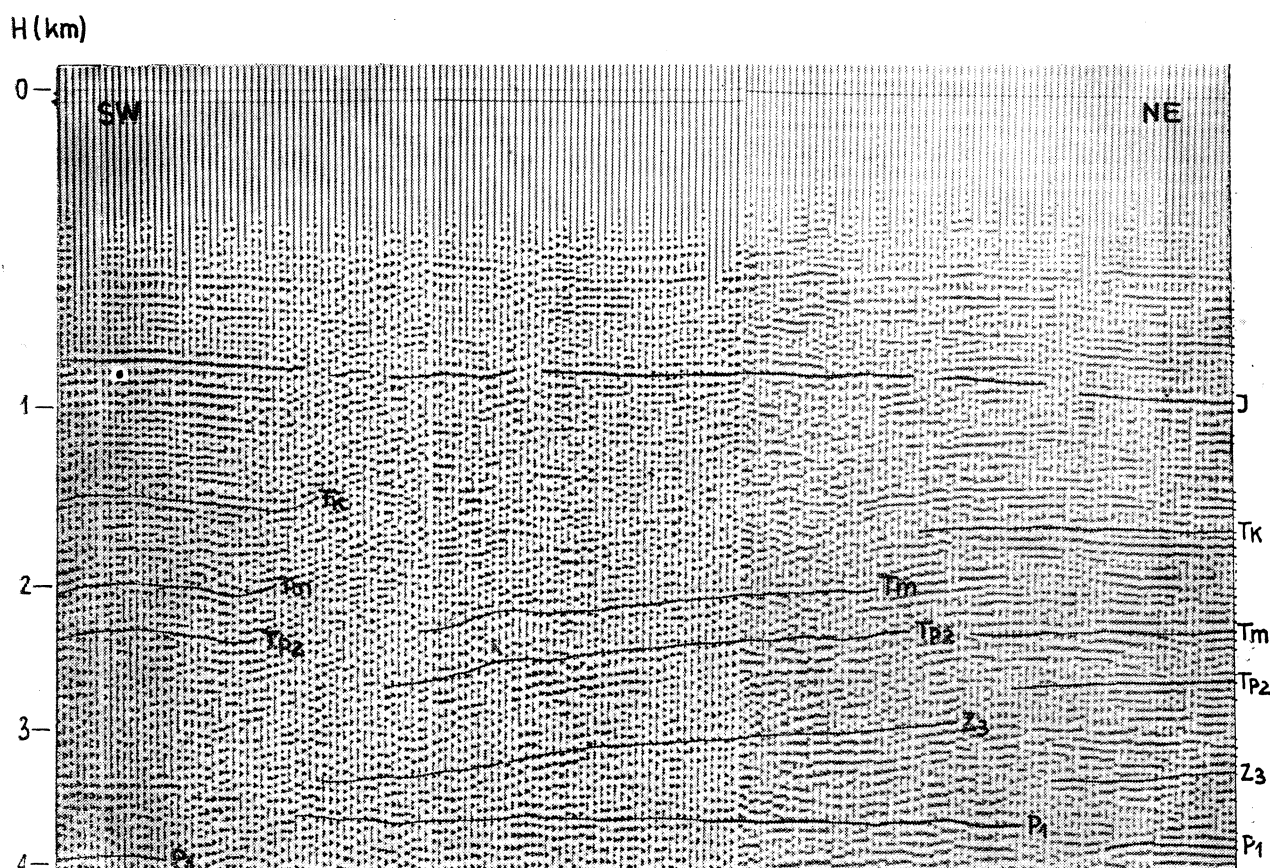
Fig. 4. Czasowy przekrój sejsmiczny 18-X-71T i 5-XIII-72T z rejonu Środy, przedstawiający blokową tektonikę i niezgodne zaleganie granicy refleksyjnej P_1 (czerwony spągowiec) w stosunku do granic młodszych. Objaśnienia przy fig. 3
