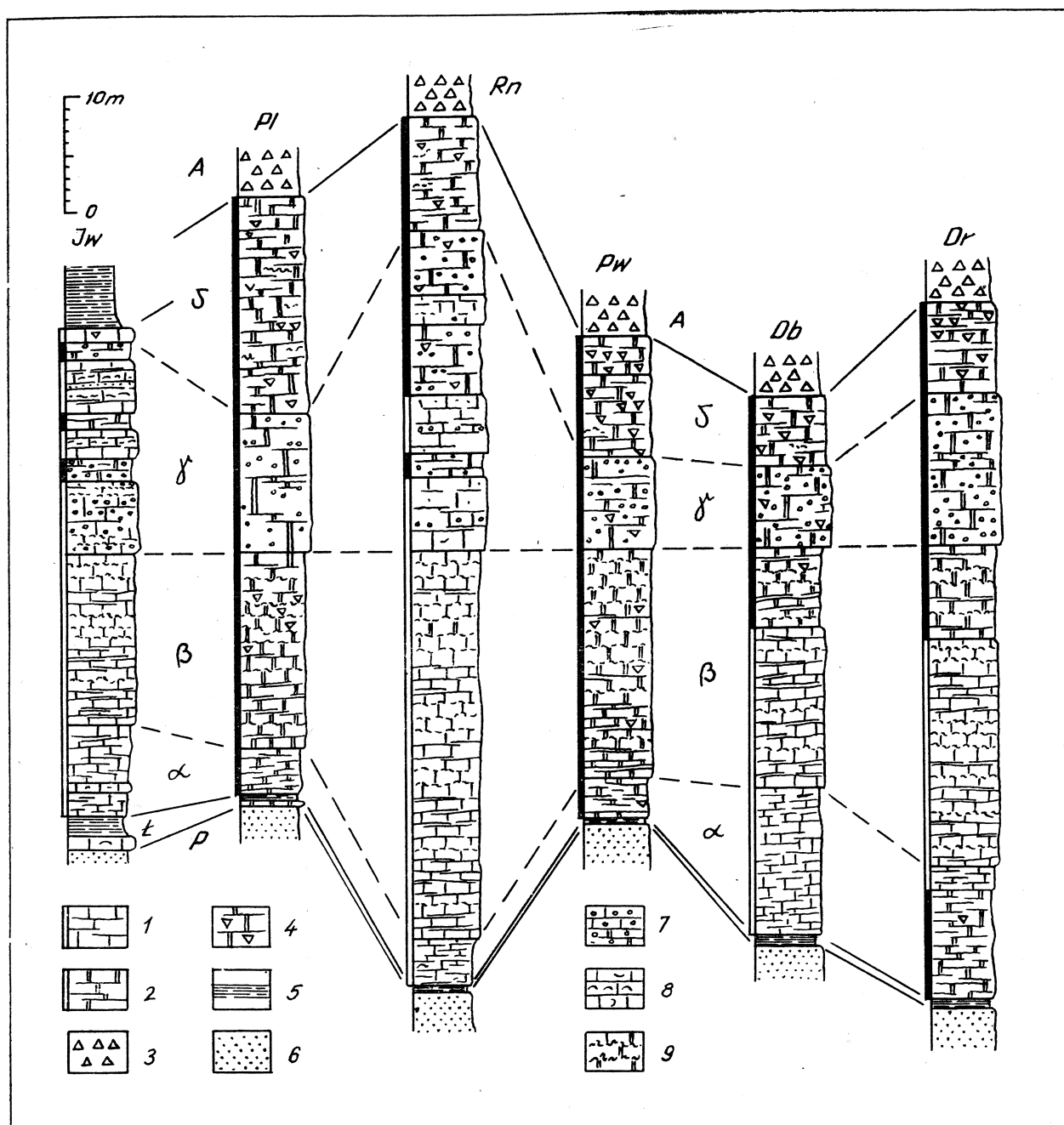
Fig. 2. Korelacja litostratygraficzna poziomów wapienia cechsztyńskiego w niecce północnosudeckiej i w południowej części monokliny przedsudeckiej. 1 — wapień; 2 — dolomity; 3 — anhydryt; 4 — dolomity z gniazdami anhydrytu; 5 — łupki; 6 — piaskowce; 7 — wapień i dolomity detrytyczne z onkoidami i intraklastami; 8 — wapień z fauną; 9 — wapień i dolomity ze stylolitami; P — biały spągowiec (lub czerwony spągowiec); Ł — łupki miedzionośne; C — czerwone łupki i mułowce; A — anhydryty; Iw — Iwiny; Pl — Polkowice; Rd — Rudna; Pw — Pawłów; Db — Dobrzeń; Dr — Drołtowice
