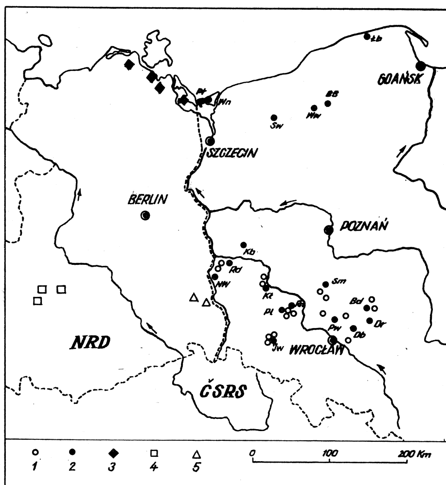
Fig. 1. Mapka rozmieszczenia profili z rozpoznanymi poziomami litostratigraficznymi wapienia cechsztyńskiego. 1 — profile z zachodniej Polski nie zamieszczone na fig. 2—4; 2 — profile z zachodniej Polski zamieszczone na fig. 2—4; 3 — profile z Meklenburgii; 4 — profile z rejonu Mansfeldu; 5 — Profile z Łużyc. Objasnienia literowe profili są podane na fig. 2—4
