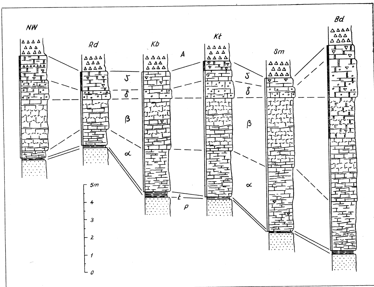
Fig. 3. Korelacja litostratygaficzna poziomów wapienia cechsztyńskiego w środkowej i północnej części monokliny przedsudeckiej, oraz na peryklinie Żar. NW — Nowa Wioska; Rd — Raduszec; Kb — Kosobudz; Kł — Kielcz; Sm — Smiłowo; Bd — Bogdaj (pozostałe objaśnienia jak na fig. 2)
