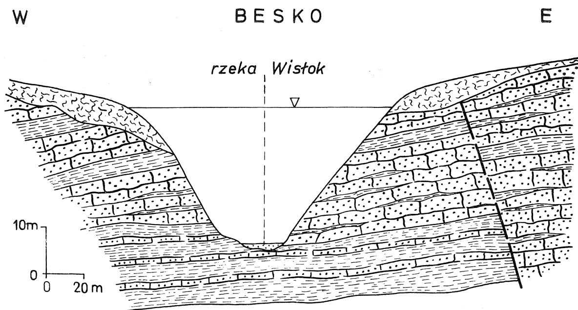
Fig. 7. Schematyczny przekrój geologiczny warstw krośnieńskich w dolinie Wisłoka koło Beska. Objaśnienie znaków na fig. 2
