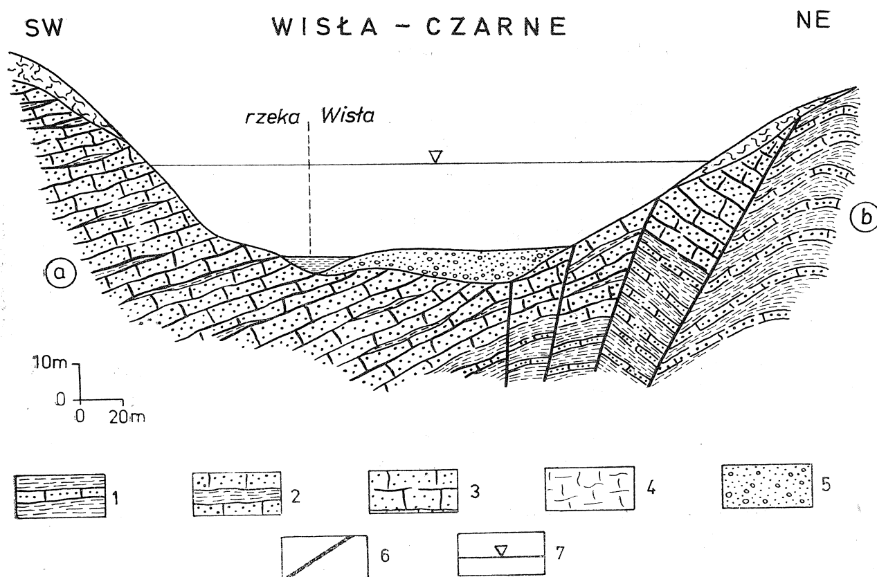
Fig. 2. Schematyczny przekrój doliny Wisły w miejscowości Wisła-Czarne. 1 — flisz łupkowy; 2 — flisz normalny; 3 — flisz piaszczysty; 4 — glina zwietrzelinowa; 5 — osad rzeczny; 6 — uskoki; 7 — przewidywana wysokość piętrzenia rzeki; a — warstwy istebniańskie dolne; b — warstwy godulskie górne
