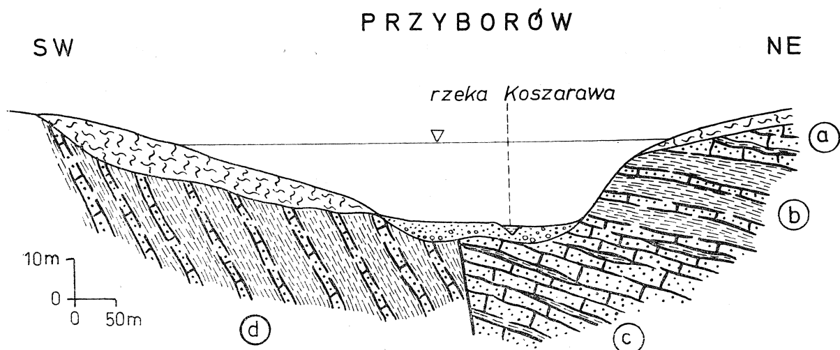
Fig. 3. Schematyczny przekrój geologiczny doliny Koszarawy w okolicy Przyborowa. a — warstwy inoceramowe; b — pstre łupki; c — piaskowce ciężkowickie; d — warstwy hieroglifowe. Inne symbole jak na fig. 2
