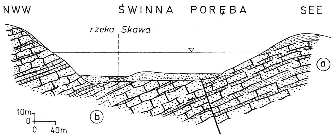
Fig. 5. Schematyczny przekrój geologiczny przez dolinę Skawy koło Świnnej Poręby. a — warstwy istebniańskie górne; b — warstwy istebniańskie dolne. Objaśnienia innych symboli na fig. 2
