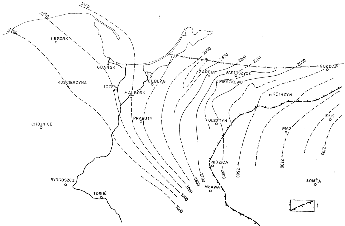
Fig. 2. Izolinie średnich prędkości do stropu kambru, w m/sec; 1 — zasięg kambru Фиг. 2. Изолинии средних скоростей до кровли кембрия, в м/сек; 1 — Граница распространения отложений кембрия
