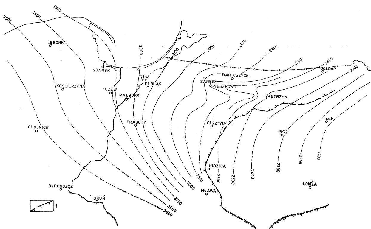
Fig. 1. Izolinie średnich prędkości do stropu prekambru, w m/sec; 1 — zasięg kambru Фиг. 1. Изолинии средних скоростей до кровли докембрия, в м/сек; 1 — Граница распространения отложений кембрия
