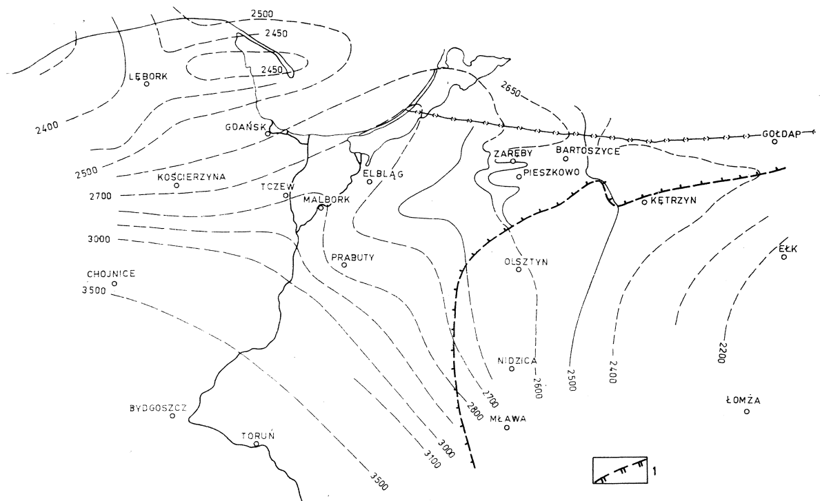
Fig. 3. Izolinie średnich prędkości do stropu syluru, w m/sec; 1 — zasięg syluru Фиг. 3. Изолинии средних скоростей до кровли силура, в м/сек; 1 — Граница распространения отложений силура
