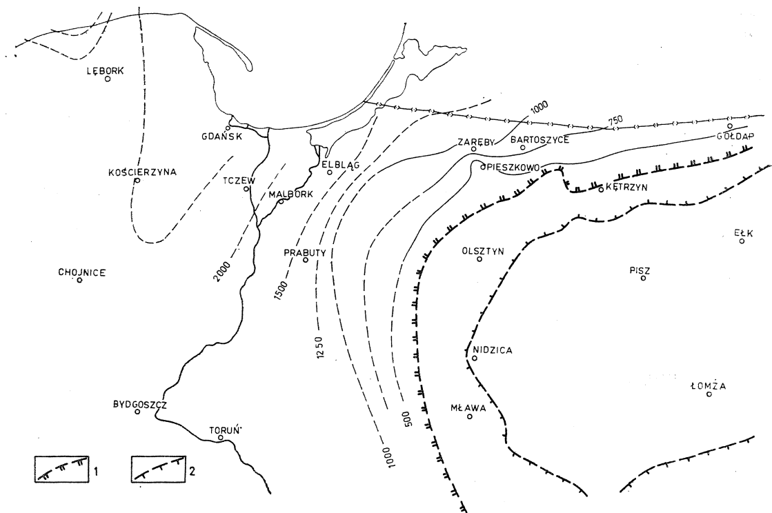
Fig. 7. Izolinie ogólnej miąższości utworów kambru, ordowiku i syluru w metrach; 1 — zasięg syluru; 2 — zasięg kambru
