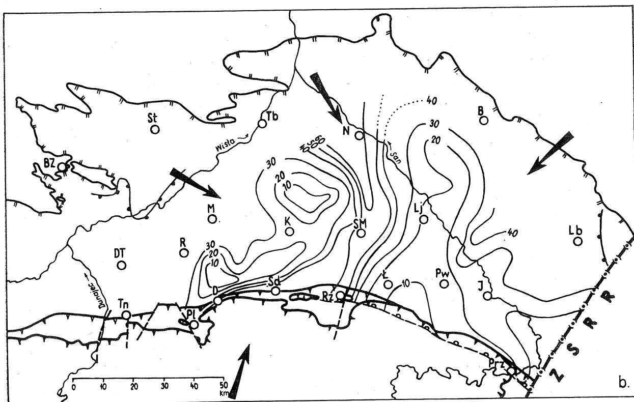
Fig. 5. Mapa miąższości (a) i zapiaszczenia (b) II kompleksu piaszczystego dolnego sarmatu, oznaczenia jak na fig. 2
