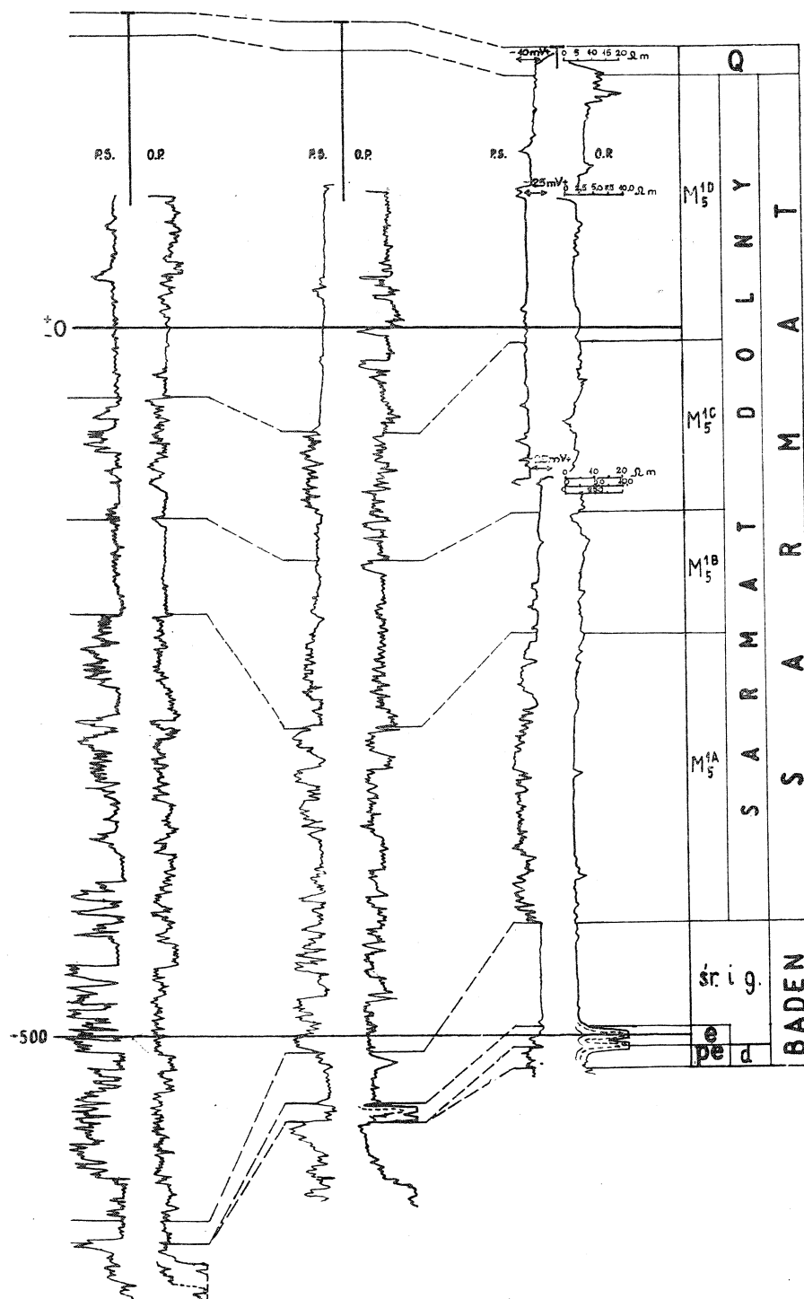
Fig. 1. Przekrój korelacyjny utworów miocennych. PS — wykres potencjałów samoistnych; OP — wykres oporności pozornej (sonda gradientowa spągowa); pe — seria podewaporatowa; e — seria ewaporatowa; M_5^A — I kompleks piaszczysty; M_5^B — kompleks ilasto-mułowcowy; M_5^C — II kompleks piaszczysty; M_5^D — kompleks ilasto-mułowcowo-piaszczysty
