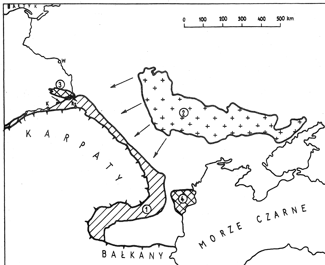
Fig. 7. Szkic pozakarpaccich obszarów alimentacyjnych zapadliska przedkarpackiego. 1 — zapadlisko przedkarpackie; 2 — krystaliczny masyw ukraiński; 3 — Góry Świętokrzyskie; 4 — masyw dobrudzki. Strzałkami zaznaczono przypuszczalny kierunek transportu materiału klastycznego
