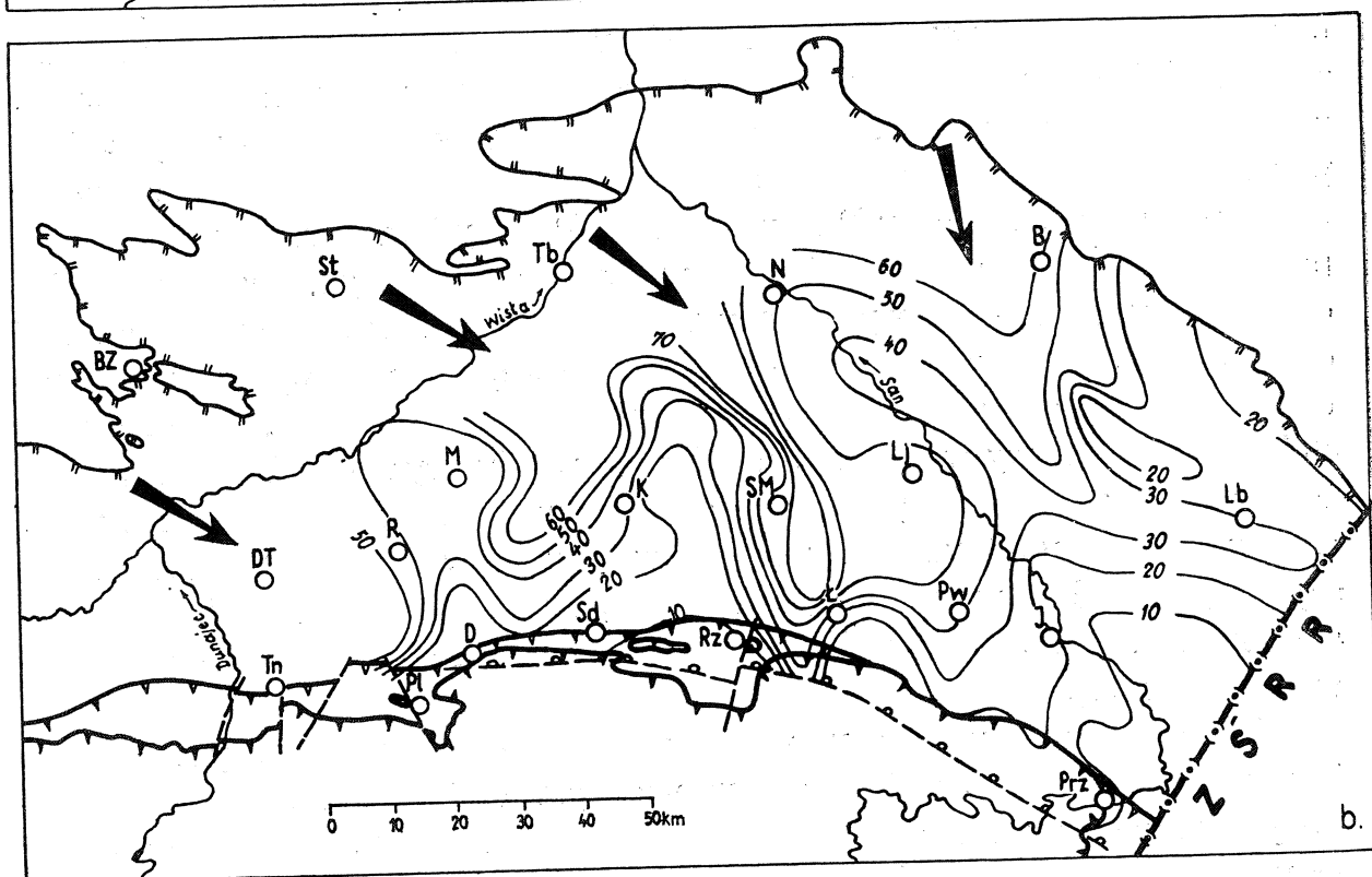
Fig. 3. Mapa miąższości (a) i zapiaszczania (b) I kompleksu piaszczystego dolnego sarmatu. Objaśnienia jak na fig. 2
