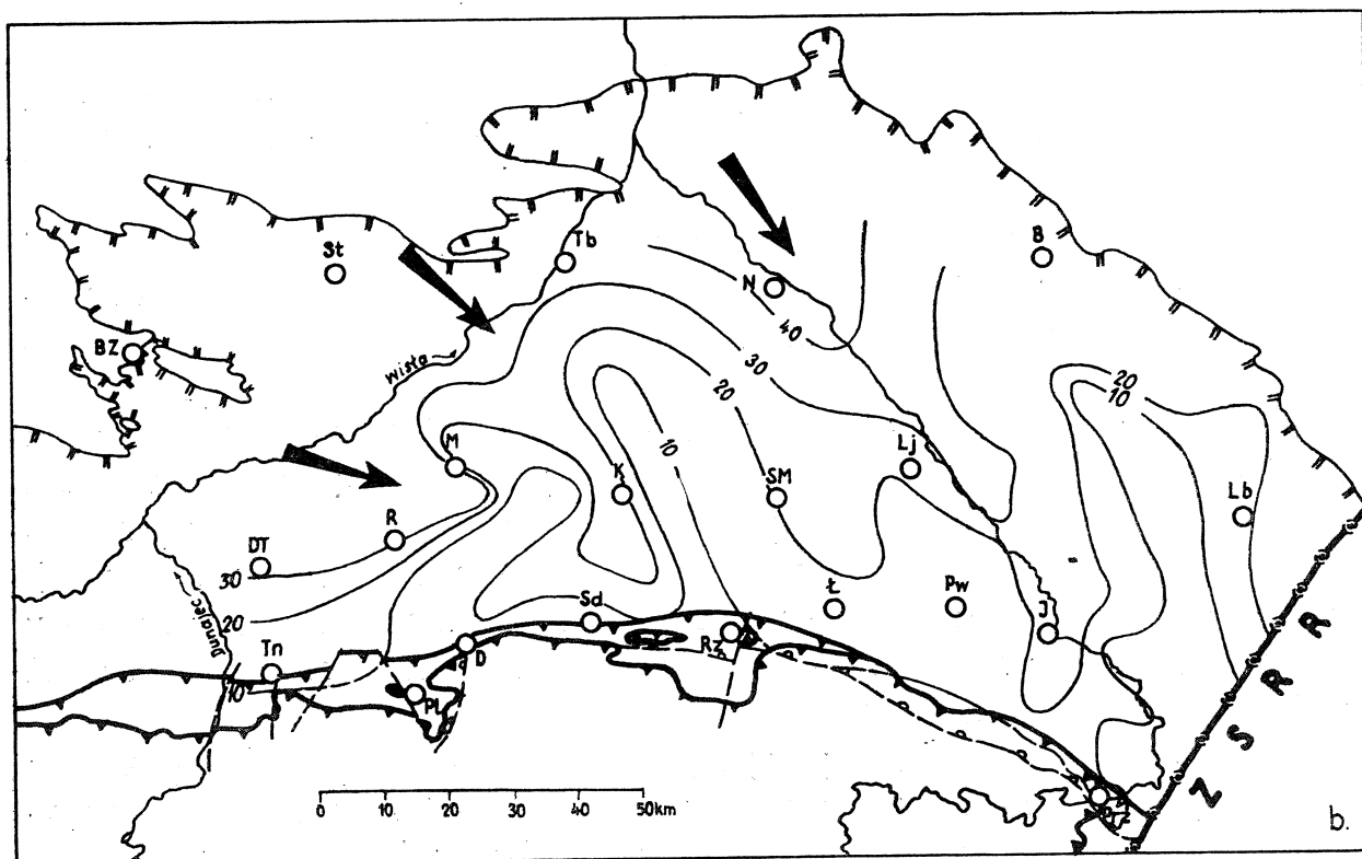
Fig. 4. Mapa miąższości (a) i zapiaszczenia (b) kompleksu ilasto-mułowcowego dolnego sarmatu, oznaczenia jak na fig. 2
