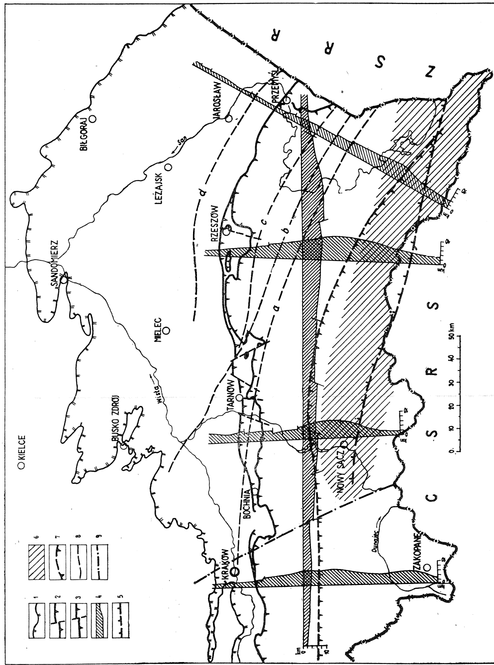
Fig. 9. Syntetyczny szkic rozwoju zapadliska przedkarpackiego w wyższym badanie i dolnym sarmacie. 1 — pólnocna granica zasięgu morskich utworów miocenu; 2 — czoło górotworu fliszowomiocenijskiego; 3 — erozyjny brzeg Karpat; 4 — kłady poziome refrakcyjnych profili sejsmicznych (wykonanych przez P. P. G., Warszawa), 5 — przypuszczalna południowa krawędź zapadliska przedkarpackiego; 6 — prawdopodobne rozmieszczenie autochtonicznych klastycznych utworów starszego miocenu; 7 — przypuszczalny erozyjny brzeg Karpat w badanie; 8 — osie zbiornika miocenijskiego; a — w wyższym badanie, b — w czasie sedymentacji I kompleksu piaszczysto-iloasto-mułowcowo-piaszczystego; c — w czasie sedymentacji II kompleksu piaszczystego, d — w czasie sedymentacji kompleksu łożysk; 9 — regionalna dyslokacja w podłożu miocenu. Miejscowości jak na fig. 2.
