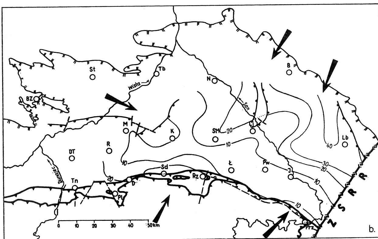
Fig. 6. Mapa miąższości (a) i zapiaszczenia (b) kompleksu ilasto-mułowcowo-piaszczystego dolnego sarmatu, oznaczenia jak na fig. 2
