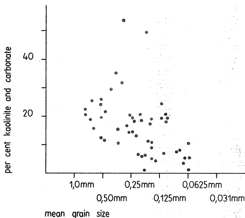
Fig. 2. Showing content of kaolinite and carbonate versus grain size (microscopic data) Fig. 2. Wykres ilustrujący zawartość kaolinitu i węglanów w zależności od rozmiarów ziarna (dane mikroskopowe)
