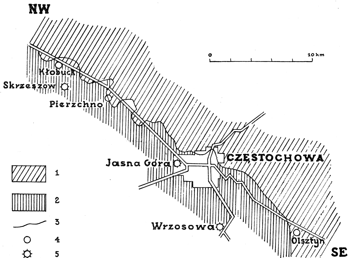
Fig. 1. Schematyczna lokalizacja odsłonieć, z których zebrano okazy. 1 — dogger; 2 — malm; 3 — granica między malmem i doggerem wg S. Z. Różyckiego; 4 — miejsca pobrania prób; 5 — wzgórza świadki Fig. 1. Index map to investigated localities. 1 — Dogger; 2 — Malm; 3 — geological boundary (according to S. Z. Różycki); 4 — localization of samples; 5 — monad- nocks
