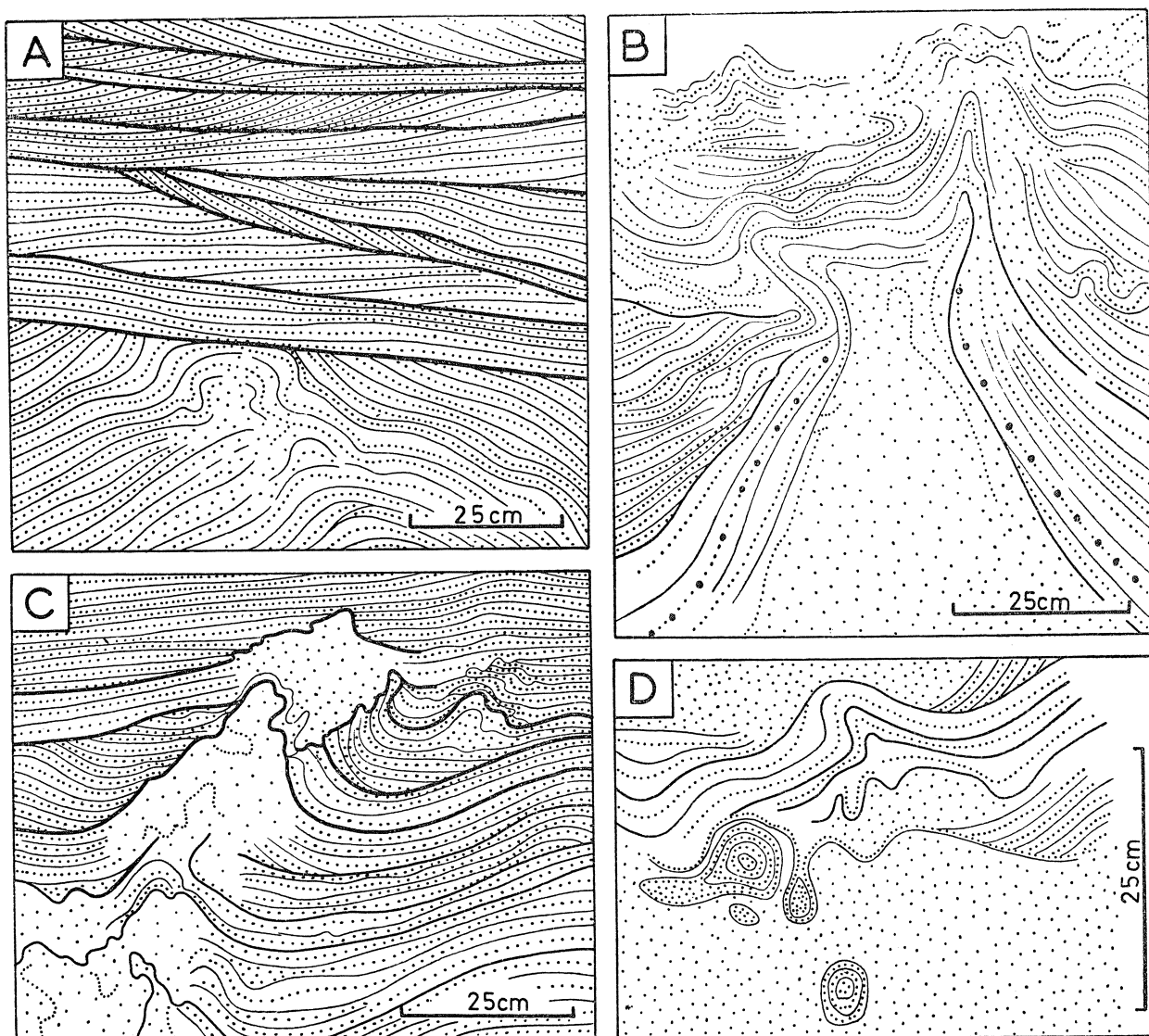
Fig. 5. Struktury sedimentacyjne i ich deformacja w piaskach sarmatu z Kolonii Rudka. Objaśnienia jak na fig. 2. A — warstwowane przekątnie piaski sarmatu. W dolnej części rysunku struktura diapirowa ścięta erozyjnie; B — struktura o charakterze diapiiru przebijająca nadległe piaski; C — częściowe zaburzenie kilku jednostek sedimentacyjnych przez tworzącą się strukturę diapirową; D — struktury kropłowe w piaskach
