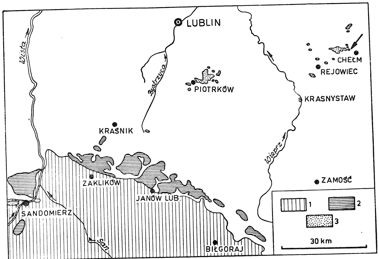
Fig. 1. Zasięg facji sarmatu na Wyżynie Lubelskiej i terenach sąsiednich. 1 — iły krakowieckie; 2 — osady węglanowe i detrytyczne; 3 — piaski z konglomeratami piaskowców; Strzałka wskazuje lokalizację badanej piaskowni
