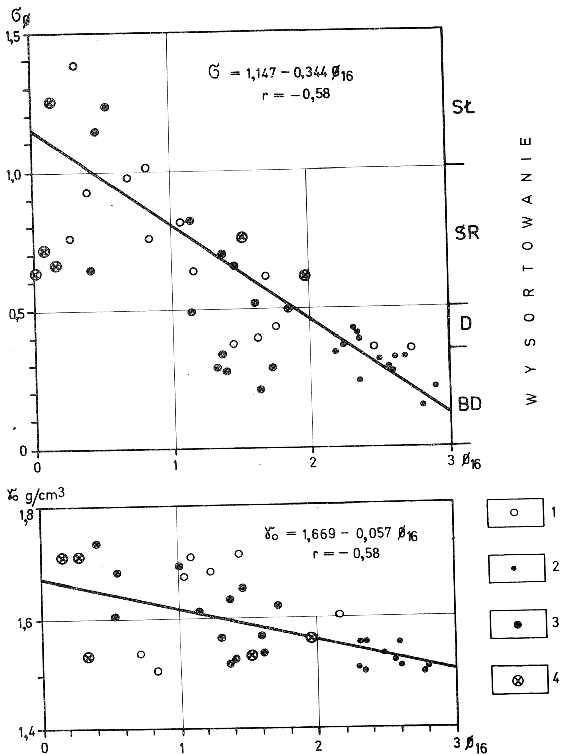
Fig. 6. Zależność pomiędzy wysortowaniem piasku \sigma\phi a wielkością ziarna ( \phi_{16} ) oraz pomiędzy gęstością ( \gamma_0 ) a wielkością ziarna ( \phi_{16} ). BD — bardzo dobrze wysortowane; D — dobrze wysortowane; SR — średnio wysortowane; SL — słabo wysortowane; 1 — piaski kompleksu górnego; 2 — piaski kompleksu dolnego, część górna; 3 — część środkowa; 4 — część dolna
