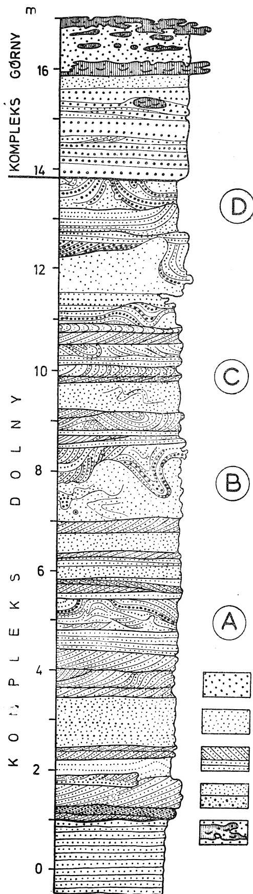
Fig. 2. Profil górnej części piaskowni w Kolonii Rudka koło Chełmu. 1 — piaski grubo i średnioziarniste; 2 — piaski drobnoziarniste; 3 — osady laminowane przekątnie lub równoległe; 4 — osady bezstrukturalne; 5 — piaskowce z fauną
