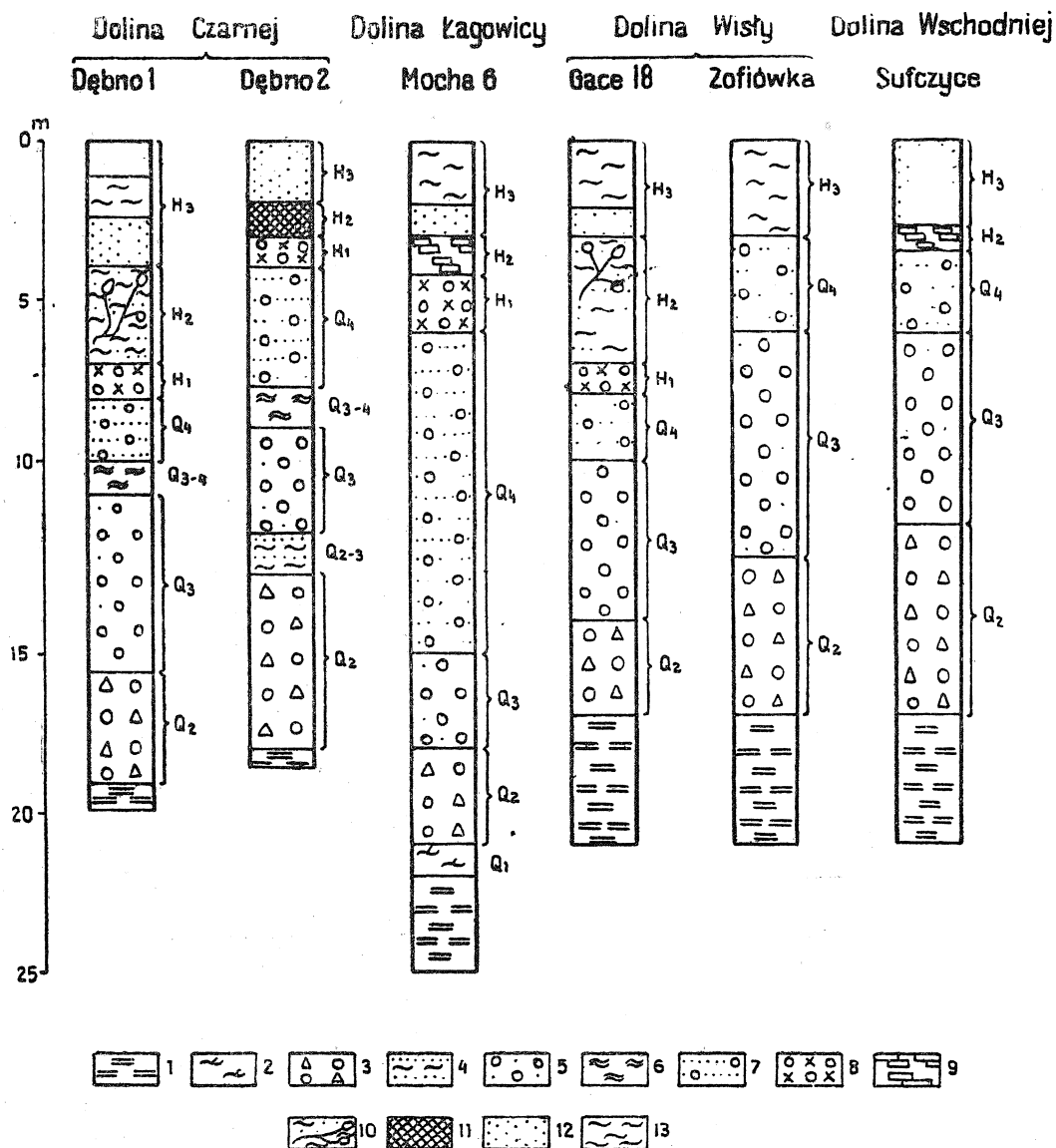
Fig. 4. Profile geologiczne z otworów wiertniczych wykonanych w dolinach południowo-wschodniej części regionu świętokrzyskiego. Starsze podłoże: 1; plejstocen: zlodowacenie najstarsze — Q_1 : 2 — mułki lessopodobne; zlodowacenie południowopolskie — Q_2 : 3 — żwiry gruboziarniste; interglacja wielka — Q_{2-3} : 4 — mułki przewarstwione piaskami; zlodowacenie środkowopolskie — Q_3 : 5 — żwiry średnioziarniste; interglacja eemski — Q_{3-4} : 6 — mułki; zlodowacenie północnopolskie; Q_4 : 7 — piaski rzeczne; holocen: holocen starszy — H_1 : 8 — żwiry facji korytowej; holocen, okres atlantycki — H_2 : 9 — torfy, 10 — piaski i mułki z florą, 11 — gleba kopalna; holocen młodszy — H_3 : 12 — piaski drobnoziarniste (rzeczne) 13 — mady
