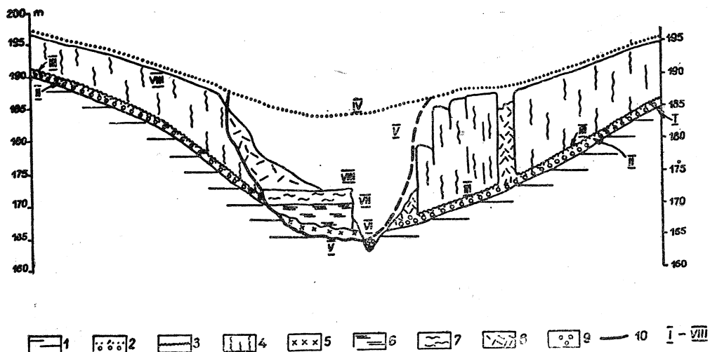
Fig. 6. Schematyczny przekrój geologiczny przez wąwóz w Zborówku koło Pacanowa. Tercjorzęd: 1 — ily krakowieckie; starszy plejstocen od preglacjalu po interglacjal eemski: 2 — żwiry i piaski; interglacjal eemski: 3 — gleba kopalna; złodowacenie północnopolskie: 4 — less; holocen starszy — h 1 : 5 — żwiry i piaski facji korytowej; holocen — okres atlantycki, h 2 ; 6 — namuły torfiaste; holocen młodszy — h 3 : 7 — mady; 8 — koluwia; 9 — współczesne osady rzeczne (żwiry); I — powierzchnia denudacyjna podczwartorzędowa; II — akumulacyjno-denudacyjna pokrywa piaszczysto-żwirowa; III — akumulacyjna pokrywa humusowa; IV — pierwotna pokrywa lessowa; V — erozyjna dolina holoceni — h 1 ; VI — powierzchnia żwirów korytowej facji; VII — powierzchnia akumulacyjna z atlantyckiego okresu holocenu; VIII — akumulacyjne dno dzisiejszego wąwozu z dzisiejszą dolinką erozyjną tnące to dno
