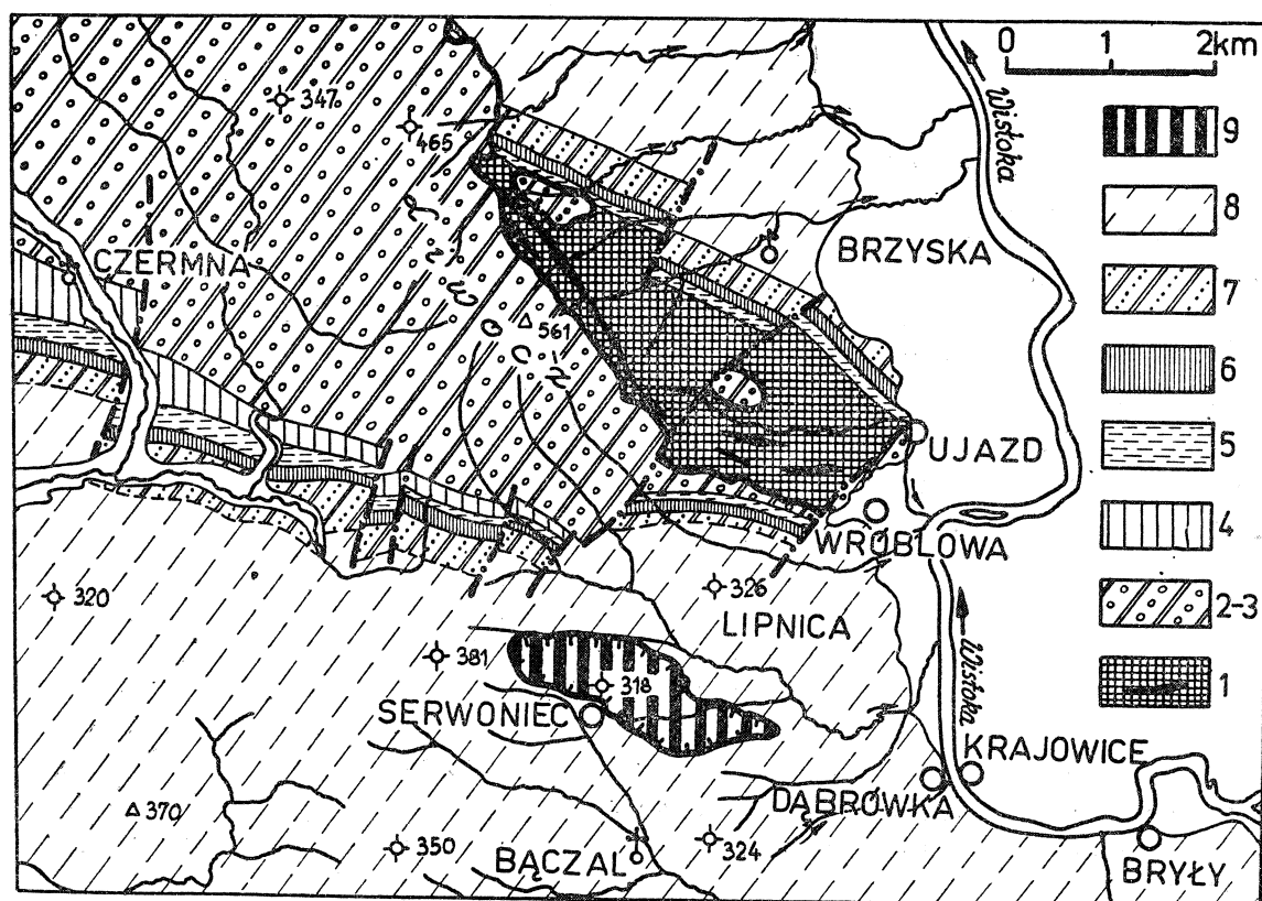
Fig. 7. Szkic tektoniczny okolic Liwocza. 1 — łupki liwockie (dolna kreda) ze smugami łupków czerwonych; 2—3 — warstwy godulskie i piaskowce istebniańskie (kreda górna); 4 — piaskowiec ciężkowicki; 5 — łupki pstre eocenu; 6 — łupki menilitowe z rogówcami w spągu; 7 — warstwy krośnieńskie dolne; 8 — warstwy krośnieńskie środkowe i górne (na południe od fałdu Liwocza także nierozdzielone); 9 — eocen magurskich płatów tektonicznych
