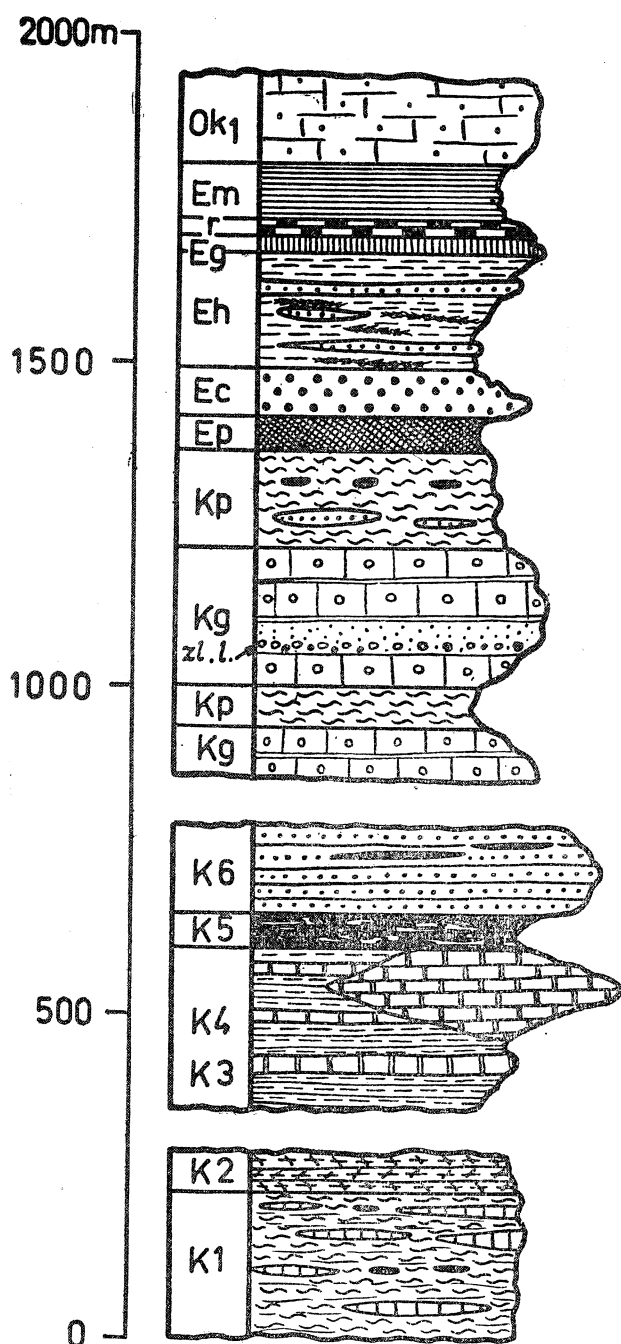
Fig. 3. Profil stratygraficzny. Walanżyn — hoteryw: K 1 — górne łupki cieszyńskie (grodziskie, łupki liwockie właściwe); Barem — apt: K 2 — łupki wierzowskie; Alb — dolny cenoman: warstwy lgockie — K 3 — łupki ilaste czarne z cienkoławicowymi piaskowcami kwarcytowymi; K 4 — piaskowce z „Krzemyka”. Cenoman górny — turon: warstwy godulskie — K 5 — łupki ilaste pstre; K 6 — piaskowce cienko-, średnio- i gruboławicowe. Senon — paleocen: Kg — piaskowce istebniańskie (zl. 1 — zlepienie z litotamniami); Kp — łupki istebniańskie. Eocen dolny: Ep — dolne pstre łupki; Ec — piaskowiec ciężkowicki. Eocen środkowy: Eh — górne pstre łupki z warstwami „hieroglifowymi”. Eocen górny: Eg — margle globigerinowe; r — rogowce; Em — łupki menilitowe. Oligocen: Ok 1 — warstwy krośnieńskie dolne — piaskowce gruboławicowe
