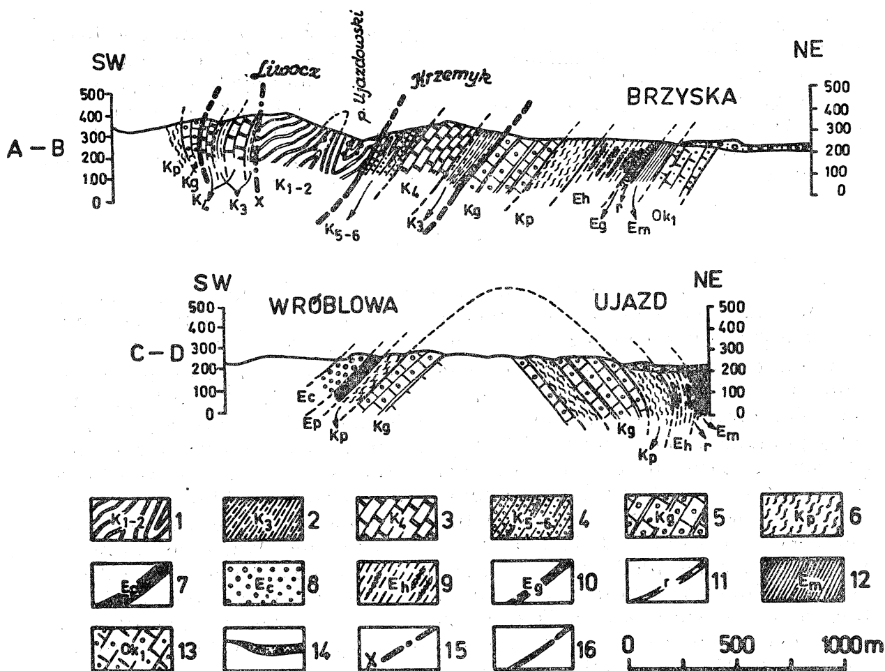
Fig. 6. Przekroje geologiczne przez wschodni koniec Liwocza. Walanżyn — hoteryw: 1 — górne łupki cieszyńskie (grodziskie, łupki liwocze właściwe); barem — apt: łupki wierzowskie. Alb — dolny cenoman: warstwy lgóckie — 2 — łupki ilaste czarne z cienkoławicowymi piaskowcami kwarcytowatymi; 3 — piaskowce z „Krzemyka”. Cenoman górny — turon: warstwy godulskie — 4 — łupki ilaste pstrye, piaskowce cienko-, średnio- i gruboławicowe. Senon — paleocen: warstwy istebniańskie — 5 — piaskowce gruboławicowe, zlepienie z litotamniami; 6 — łupki ilaste szare i ciemnoszare. Eocen dolny: 7 — dolne pstrye łupki; 8 — piaskowiec ciężkowicki. Eocen środkowy: 9 — górne pstrye łupki z warstwami hieroglifyowymi. Eocen górny: 10 — margle globigerinowe; 11 — rogowce; 12 — łupki menilitowe. Oligocen: warstwy krośnieńskie dolne — piaskowce gruboławicowe; 14 — aluwia; 15 — uskoki; 16 — nasunięcia
