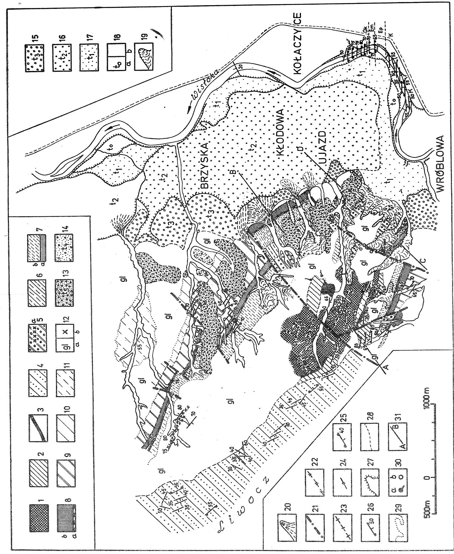
Fig. 2. Szczegółowa mapa geologiczna Liwocza. Kreda dolna: 1 — łupki czarne i piaskowce strzałkowe (warstwy ciemno-zielone); 2 — łupki czarne i piaskowce kwar- cytowe, piaskowce jasne gruboławicowe (warstwy egocenie). Kreda górna: 3 — piaskowce i łupki; 4 — piaskowce i łupki; 5 — piaskowce i łupki; 6 — piaskowce i łupki; 7a — piaskowce i łupki; 7b — piaskowce i łupki; 8a — piaskowce i łupki; 8b — piaskowce i łupki; 9 — piaskowce i łupki; 10 — piaskowce i łupki; 11 — piaskowce i łupki; 12a — piaskowce i łupki; 12b — piaskowce i łupki; 13 — piaskowce i łupki; 14 — piaskowce i łupki; 15 — piaskowce i łupki; 16 — piaskowce i łupki; 17 — piaskowce i łupki; 18 — piaskowce i łupki; 19 — piaskowce i łupki; 20 — piaskowce i łupki; 21 — piaskowce i łupki; 22 — piaskowce i łupki; 23 — piaskowce i łupki; 24 — piaskowce i łupki; 25 — piaskowce i łupki; 26 — piaskowce i łupki; 27 — piaskowce i łupki; 28 — piaskowce i łupki; 29 — piaskowce i łupki; 30a — piaskowce i łupki; 30b — piaskowce i łupki; 31 — piaskowce i łupki.
