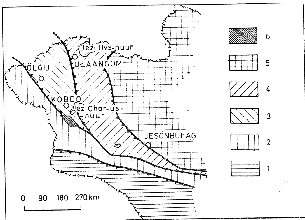
Fig. 2. Strefy strukturalno-facjalne Zachodniej Mongolii (uproszczone na podstawie V. V. Bezzubceva et al., 1963): 1 — Barunchurajska (waryscyjska); 2 — Altajska (późnokaledońska); 3 — Charchirinska (takońska); 4 — Jeziorowa (salairska); 5 — Prekambryjski masyw Changaju, przebudowany fałdowaniami salairskimi; 6 — Obszar objęty fig. 5
