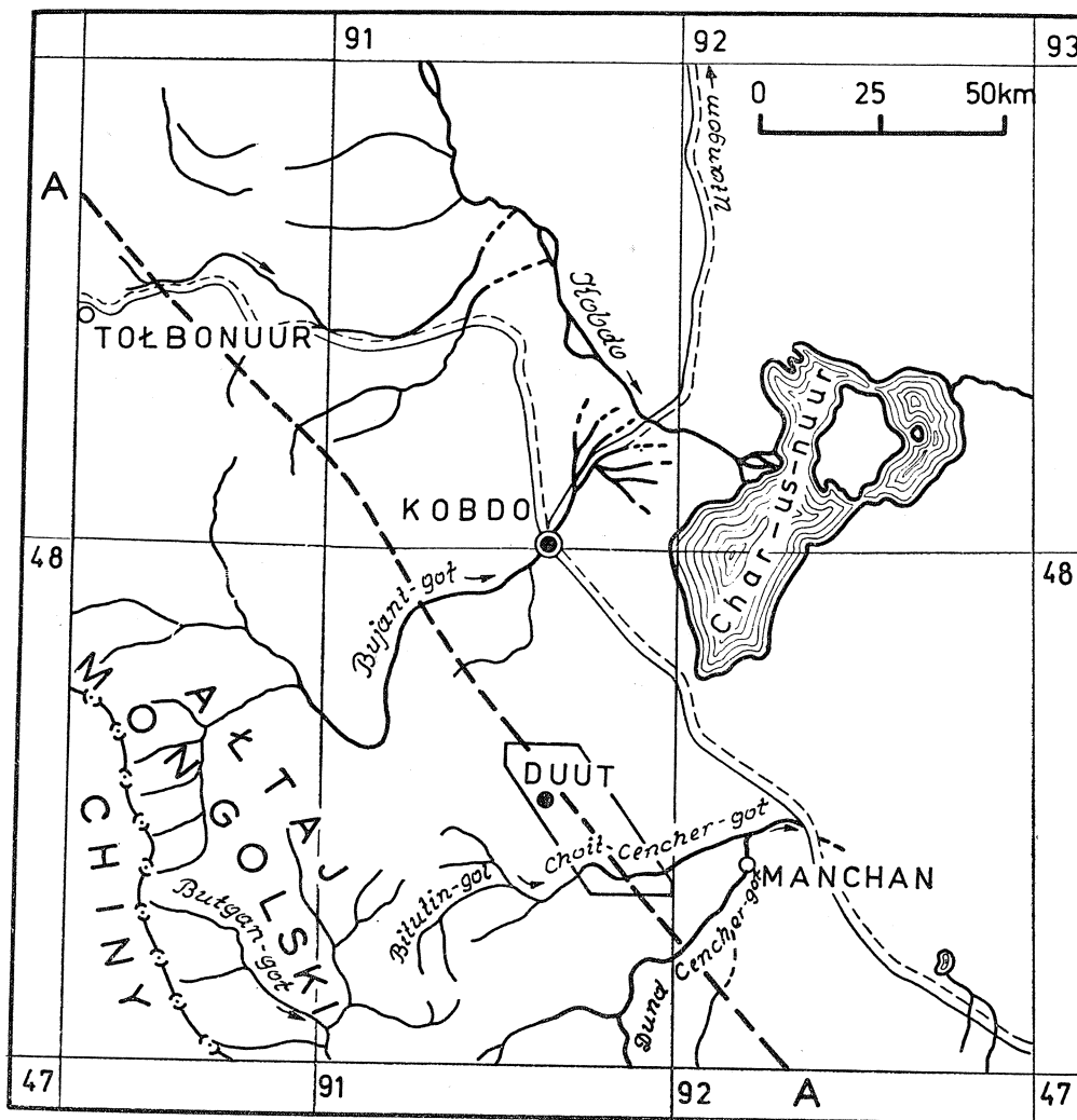
Fig. 1. Szkic środkowej części Kotliny Wielkich Jezior w Mongolii Zachodniej: A—A = Tolbonurska strefa dyslokacyjna. W ramce obszar przedstawiony na fig. 5 Fig. 1. Sketch-map of the central part of the Great Lakes Basin in Western Mongolia: A—A the Tolbonoor fault zone. Area shown in Fig. 5 in box
