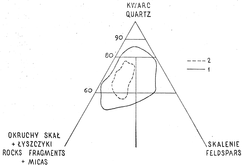
Fig. 4. Zmienność niektórych piaskowców paleogeńskich: 1 — piaskowce magurskie; 2 — piaskowce fliszu podhalańskiego Fig. 4. Variability in some Palaeogene sandstones: 1 — Magura Sandstone; 2 — sandstones from the Podhale Flysch
