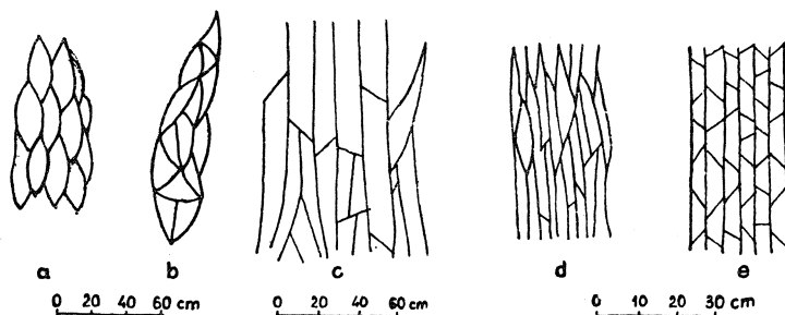
Fig. 3. Inne struktury dysjunktywne bazaltu: a — soczewki bazaltu; b — wklęsłe i wypukłe wieloboki bazaltu; c — miecze bazaltu; d — listwy; e — trapezy bazaltu Fig. 3. Other fracture structures in basalts: a — basalt lenses; b — basalt polygons with concave and convex faces; c — basalt blades; d — basalt flags; e — basalt trapezoids
