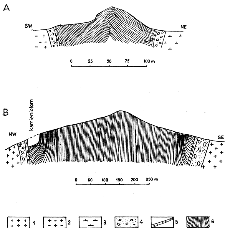
Fig. 5. Przekroje przez komin wulkaniczne: A — „Czartowska Skała” koło wsi Pomocne; B — „Szwedzkie Szańce” na SE od Lutyni; 1 — łupki łuszczykowe; 2 — zielenice; 3 — łupki kwarcytowo-sericytowe; 4 — materiał pyroklastyczny; 5 — partia brzeżna bazaltu; 6 — partia słupów bazaltowych
