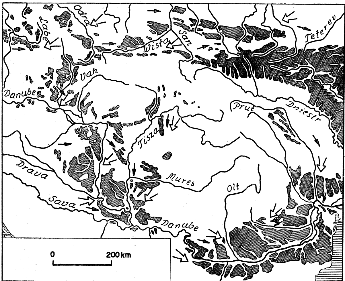
Fig. 1. Rozmieszczenie lessów we wschodniej części Europy środkowej. Opracował H. Maruszczak na podstawie map opublikowanych przez E. Rühlego i M. Sokołowską (1955), D. Jaranowa (1956), P. K. Zamorij i G. M. Molawkę (1956), G. Raileanu et al. (1959), J. Sekyrę (1960) i M. Pécsiego (1962). Kierunki wiatrów przeważających, zrekonstruowane dla głównej fazy akumulacji lessu w okresie ostatniego zlodowacenia, oznaczone schematycznie strzałką podwójną. Kierunki wiatrów przeważających obecnie oznaczone strzałką pojedynczą. Fig. 1. Distribution of loess in East-Central Europe. Elaborated by the author on the basis of maps published by E. Rühle and M. Sokołowska (1955), D. Jaranoff (1956), P. K. Zamorij and G. M. Molawko (1956), G. Raileanu et al. (1959), J. Sekyra (1960) and M. Pécsi (1962). Prevailing wind directions reconstructed for the main phase of loess accumulation during the last glaciation are marked schematically by a double arrow. Recent wind directions marked by a single arrow.
