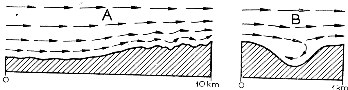
Fig. 2. Schematyczne przekroje ilustrujące zmiany układu i szybkości wiatrów przyziemnych skierowanych prostopadle do: A — progu morfologicznego oddzielającego niżej położoną płaską równinę od silniej urzeźbionej wyżyny (przedgórze), B — osi małej doliny. Długość strzałek oznaczających kierunek wiatru proporcjonalna do jego szybkości. Rysunek A zestawiony w oparciu o dane ilustrujące zmiany szybkości wiatru w zależności od wysokości nad powierzchnią terenu i charakteru jego urzeźbienia. Rysunek B natomiast oparty na zestawionych przez R. Geigera (1957) schematach układu wiatrów na polanach i zrębach śródlęśnych
