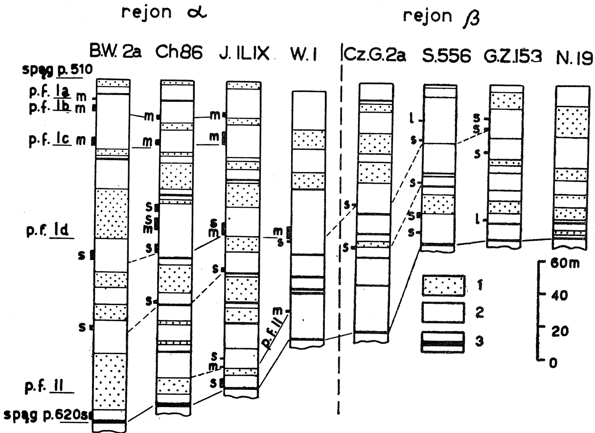
Fig. 2. Korelacja poziomów faunistycznych w górnej części warstw porubskich w północno-wschodniej części Górnośląskiego Zagłębia Węglowego. 1 — piaskowce; 2 — iły i mułowce; 3 — pokład węgla; m — fauna morska; s — fauna słodkowodna; L — fauna lingulowa; pf — poziom faunistyczny
