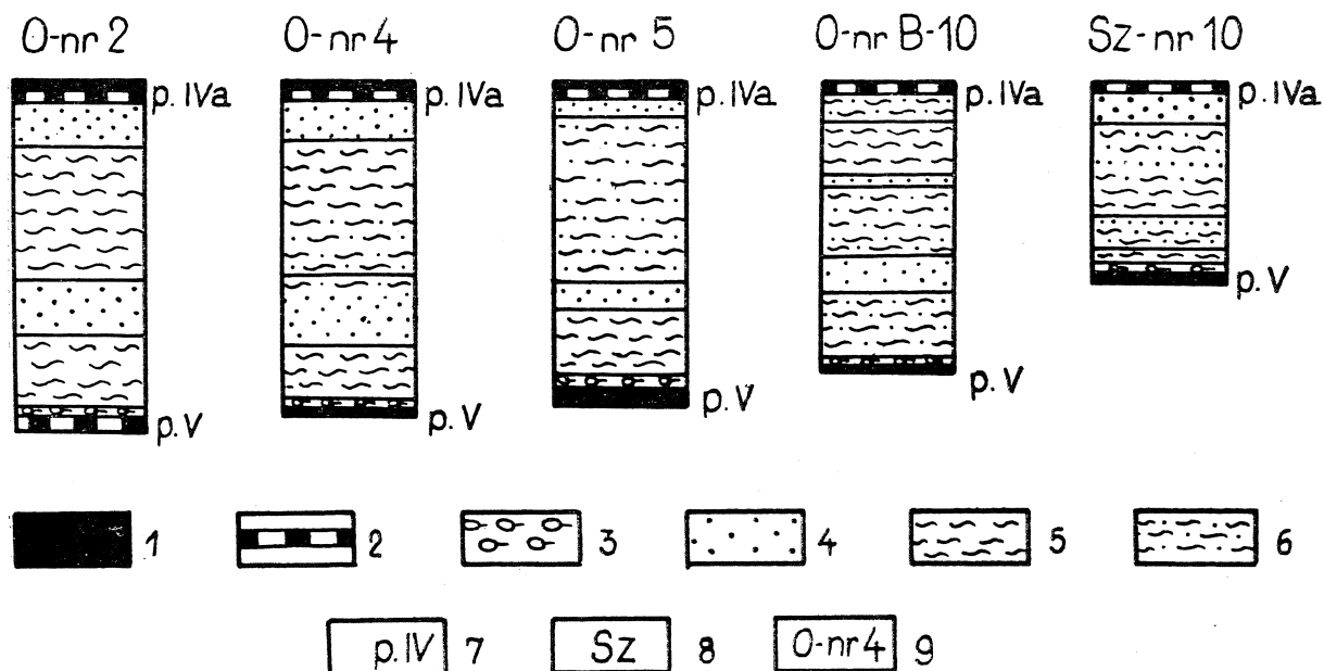
Fig. 8. Przykład zmienności faz cyklotemu wzdłuż biegu warstw w kierunku S — N. 1 — węgiel; 2 — ił węglisty; 3 — muszlowiec; 4 — piaskowiec; 5 — iłowiec; 6 — piaszczysty iłowiec; 7 — numer pokładu węgla; 8 — sztolnia; 9 — numer otworu wiertniczego
