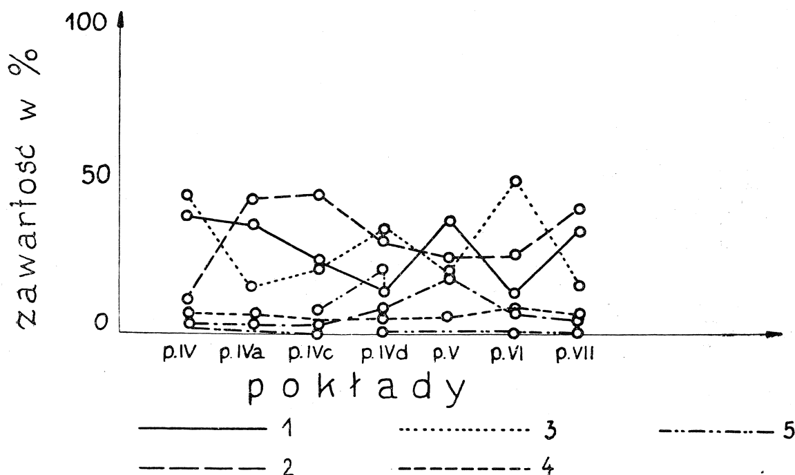
Fig. 9. Diagram udziału różnych odmian węgla i skały płonnej w budowie petrograficznej poszczególnych pokładów. Zestawiono wg danych z badań GJG — Katowice (10). 1 — witryt; 2 — klaryt; 3 — duryt; 4 — fuzyt; 5 — łupek palny; 6 — skała płonna
