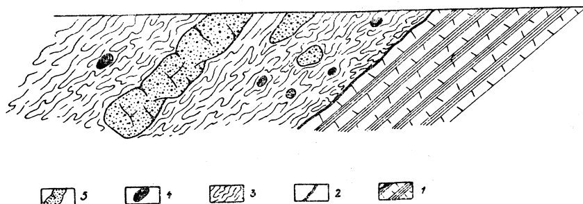
Fig. 8. Schemat kontaktu warstw krośnieńskich z utworami płata Kluczowej: 1 — Łupki krośnieńskie, 2 — Granica kontaktu, 3 — Łupki magurskie, 4 — Okruchy margli brunatnych, 5 — Piaskowiec glaukonitowy brekcyjowy
