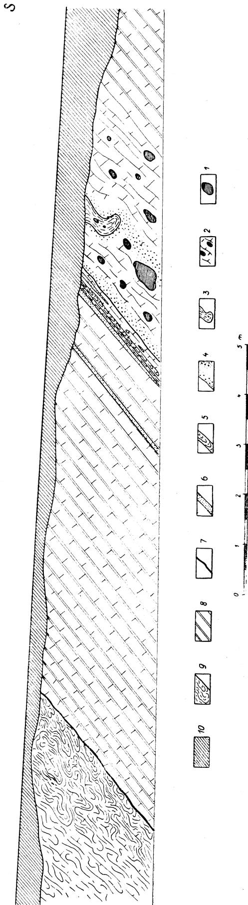
Fig. 2. Schemat odsłonięcia wschodniej ściany drogi z Kołaczyc do Kluczowej: 1 — Otoczaki różnych typów łupków i margli oraz piaskowców pochodzenia magurskiego, 2 — Łupki krośnieńskie z drobnym materiałem magurskim, 3 — Soczewka łupków magurskich, 4 — Łupki krośnieńskie z domieszką rdzawego piasku i żwirku kwarcowego, 5 — Wkładka osuwiskowa z łupkami magurskimi, 6 — Piaskowiec rdzawy z detrytusem łupków magurskich, 7 — Kontakt łupków krośnieńskich z utworami płyta, 8 — Łupki krośnieńskie bez otoczek materiału magurskiego, 9 — Utwory płyta Kluczowej, 10 — Gliny zwietrzelinowe Fig. 2. Scheme showing outcrop of eastern wall of the road from Kołaczyc to Kluczowa: 1 — Pebbles of different types of shales, marls and sandstones from Magura nappe, 2 — Krosno shales with fine Magura material, 3 — Lenticle of Magura shales, 4 — Krosno shales with admixture of rusty sand quartz grit, 5 — Bed with slump structures of Magura shales, 6 — Rusty sandstone with breccia of Magura shales, 7 — Contact of Krosno shales with deposits of the outlier, 8 — Krosno shales without pebbles of Magura material, 9 — Deposits of Kluczowa outlier, 10 — Residual clays
