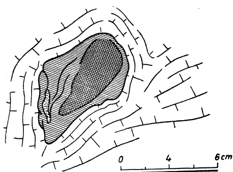
Fig. 7. Łupki krośnieńskie z otoczką syderytu w Kluczowej
