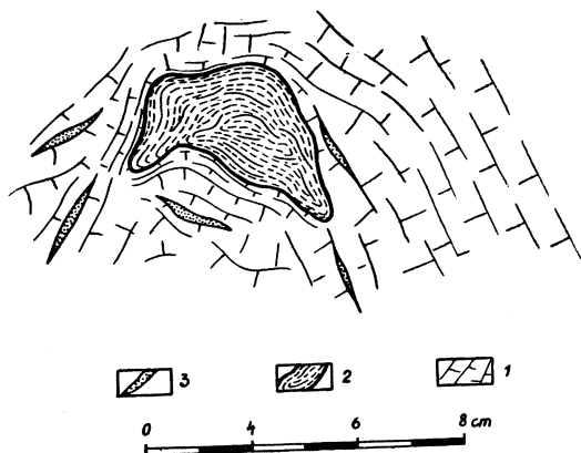
Fig. 6. Fragment odsłonięcia łupków krośnieńskich z soczewką łupków magurskich w Kluczowej: 1 — Łupki krośnieńskie, 2 — Łupki magurskie, 3 — Soczewki białoszarego i szarzielonego piasku
