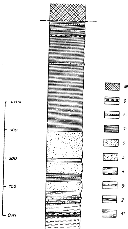
Fig. 11. Profil litologiczno-stratygraficzny serii menilitowo-krośnieńskiej w Nawsiu: 1 — Warstwy hieroglifowe, 2 — Margle globigerynowe, 3 — Warstwy podrogowcowe, 4 — Łupki menilitowe z rogowcami, 5 — Piaskowiec kliwski, 6 — Piaskowce krośnieńskie gruboławicowe, 7 — Łupki krośnieńskie z cienkimi wkładkami piaskowców płytowych i skorupowych, 8 — Wkładki piaskowców gruboławicowych, 9 — Ławica osuwiskowa z otoczkami i okruchami margli węglowieckich, 10 — Margle węglowieckie płyta podśląskiego
