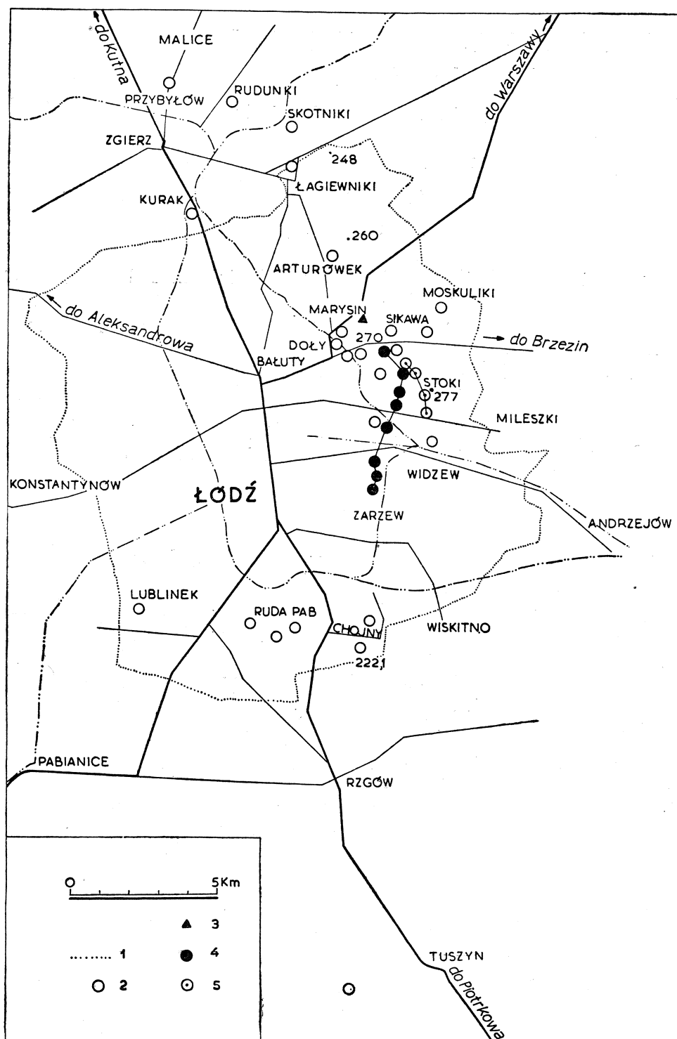
Fig. 1. Rozmieszczenie stanowisk lessu w obrębie Łodzi. 1 — granice miasta; 2 — zbadane stanowiska lessów; 3 — odkrywka w glinie warciańskiej; 4 — przekrój (fig. 5); 5 — przekrój (fig. 6)
