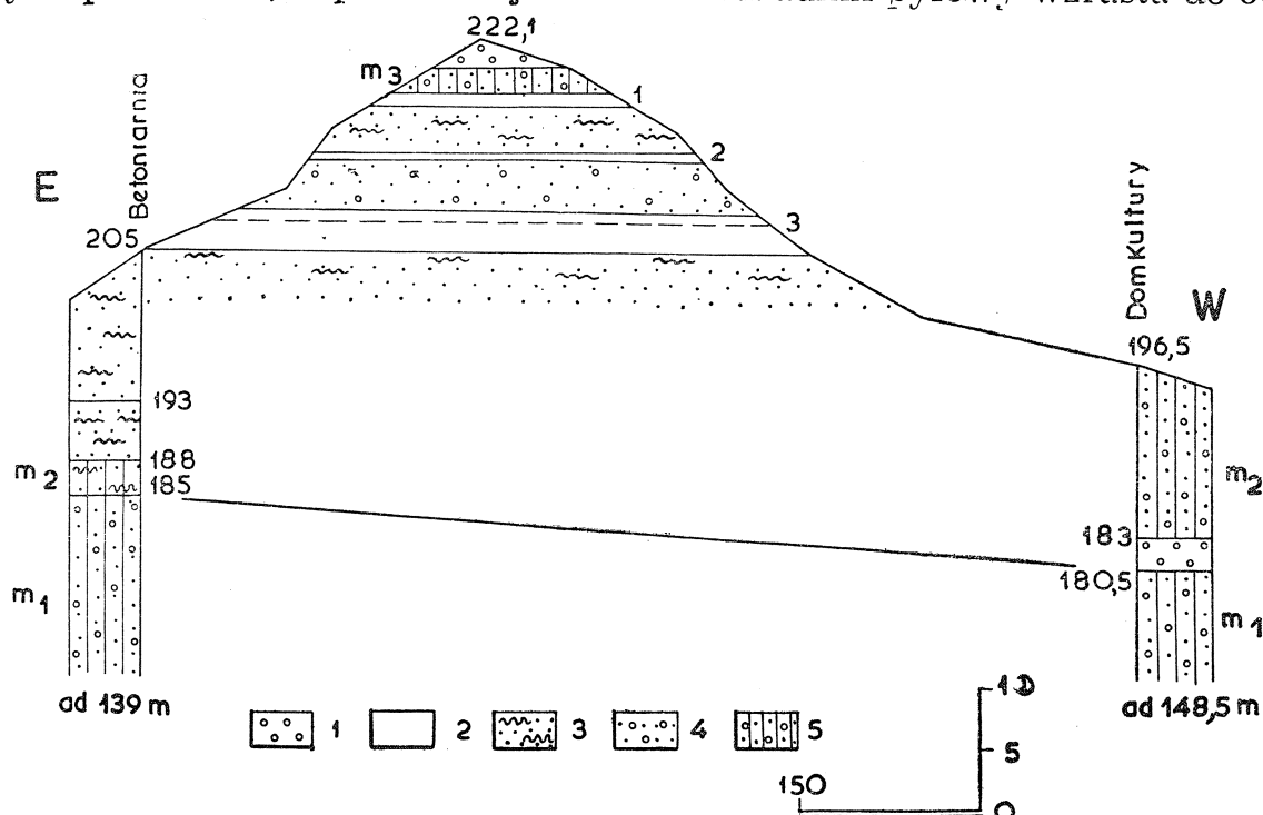
Fig. 3. Górki Nowe — Przekrój korelacyjny utworów czwartorzędowych. m_1 — morena krakowska; m_2 — morena środkowopolska; m_3 — morena stadium Warty; 1, 2, 3 — poziomy lessu; 1 — żwiry; 2 — lessy; 3 — piaski pylaste, 4 — piaski ze żwirem; 5 — glina zwałowa
