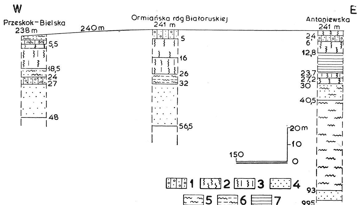
Fig. 4. Widzew (Antoniew — Stoki). 1 — glina; 2 — less żółty; 3 — less ilasty żółty; 4 — piaski; 5 — muły popielate; 6 — il szary, mulisty; 7 — ily warwowe Фиг. 4. Видзев (Антонев — Стоки). 1 — глина, 2 — желтый лёсс, 3 — желтый иластый лёсс, 4 — пески, 5 — серые алевриты, 6 — серый алевритовый ил, 7 — варвовые илы
