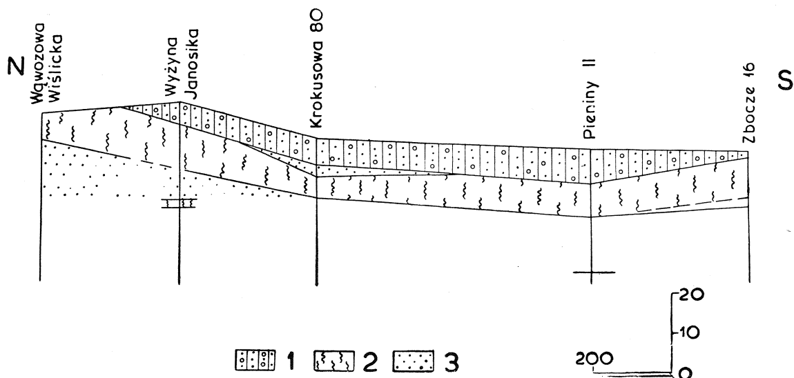
Fig. 5. Stoki. 1 — glina zwałowa; 2 — lessy; 3 — piaski Фиг. 5. Стоки. 1 — отвальная глина, 2 — лёссы, 3 — пески
