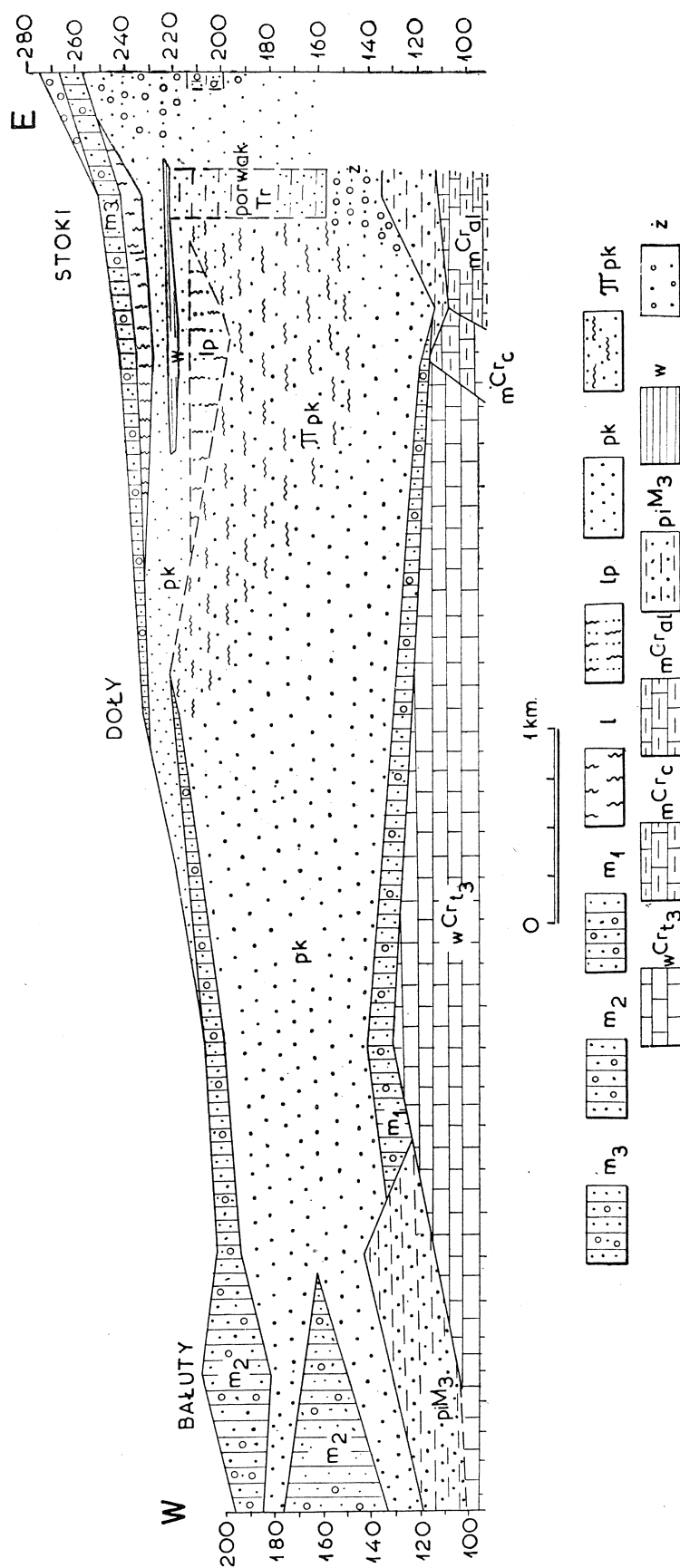
Fig. 2. Przekrój geologiczny Łódź W—E. m_3 — morena stadium Warty; m_2 — morena środkowopolska; m_1 — morena krakowska; l — lessy; lp — lessy piaszczyste; pk — piaski; l_{pk} — pyły piaszczyste; z — żwir; w — ily warwowe; m_3 — piaski ilaste miocenijskie; w_{Crt_3} — wapienie turońskie; m_{Cr_c} — margle cenomańskie; m_{Cr_{al}} — margle albskie
