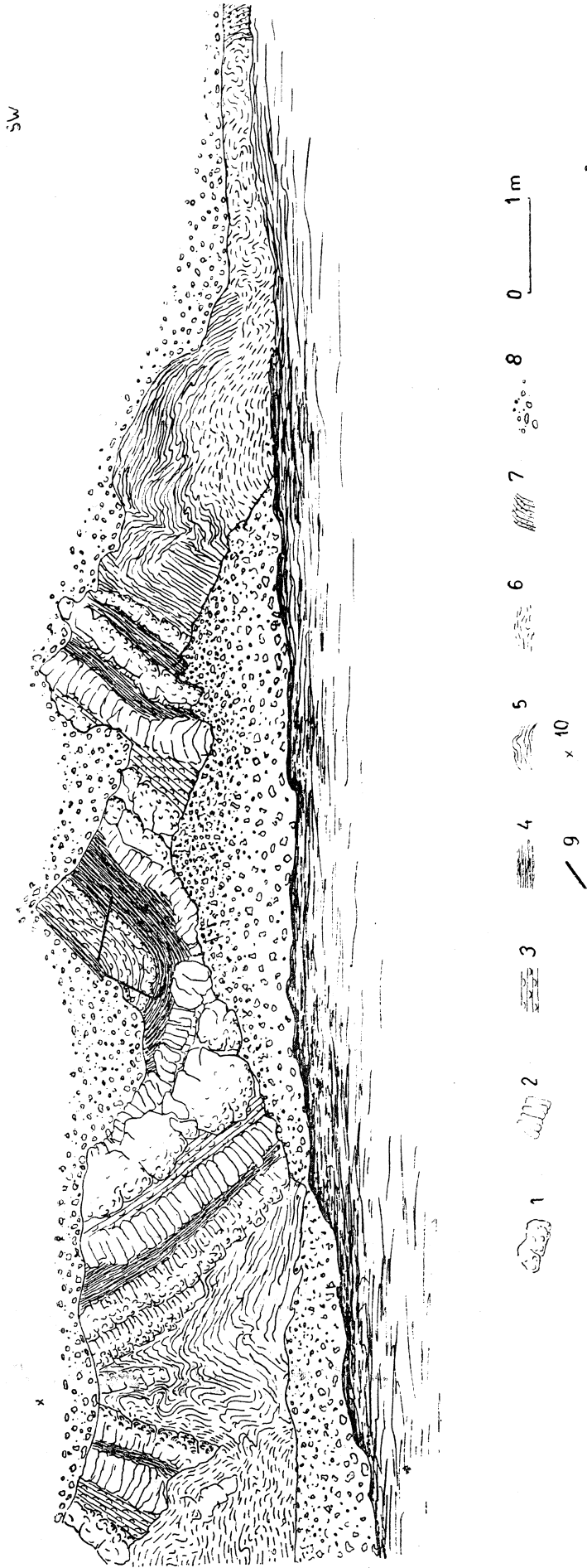
Fig. 5. Szkic południowo-zachodniej części odkrywki poziomu z egzotykami w Bukowcu (wg fotografii wykonana p. Jadwiga Strzepka). 1 — muszlowiec; 2 — wapień marglisty; 3 — łupki oliwkowobrunatne z fragmentami skorup; 4 — łupki margliste, zielone; 5 — łupki brunatne (menilitowe); 6 — łupki szare z egzotykami; 7 — cienko ławicowe piaskowce krośnieńskie; 8 — gruz zwietrzelinowy; 9 — linie uskoku; 10 — fragment przedstawiony na fotografii na tabl. XII fig. 1.
