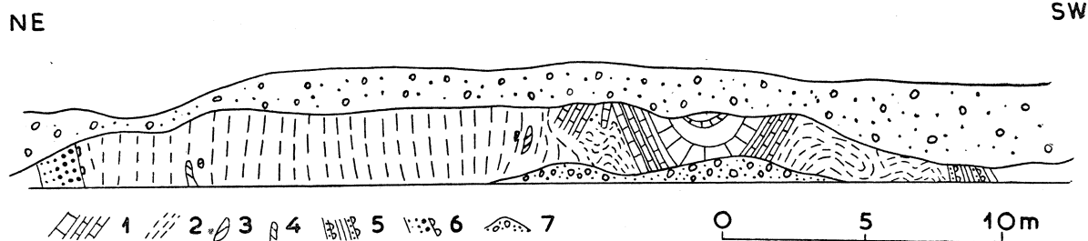
Fig. 4. Schematyczny rysunek odsłonięcia w Bukowcu (stan w roku 1957). 1 — ławice muszlowców przekładane łupkami zielonymi (szczegóły przedstawione na fig. 5); 2 — łupki szare z egzotykami; 3 — pakiet łupków zielonych; 4 — ławica ankerytu; 5 — cienkoławicowe piaskowce krośnieńskie; 6 — gruboławicowe piaskowce krośnieńskie; 7 — żwiry osypiska i terasy
