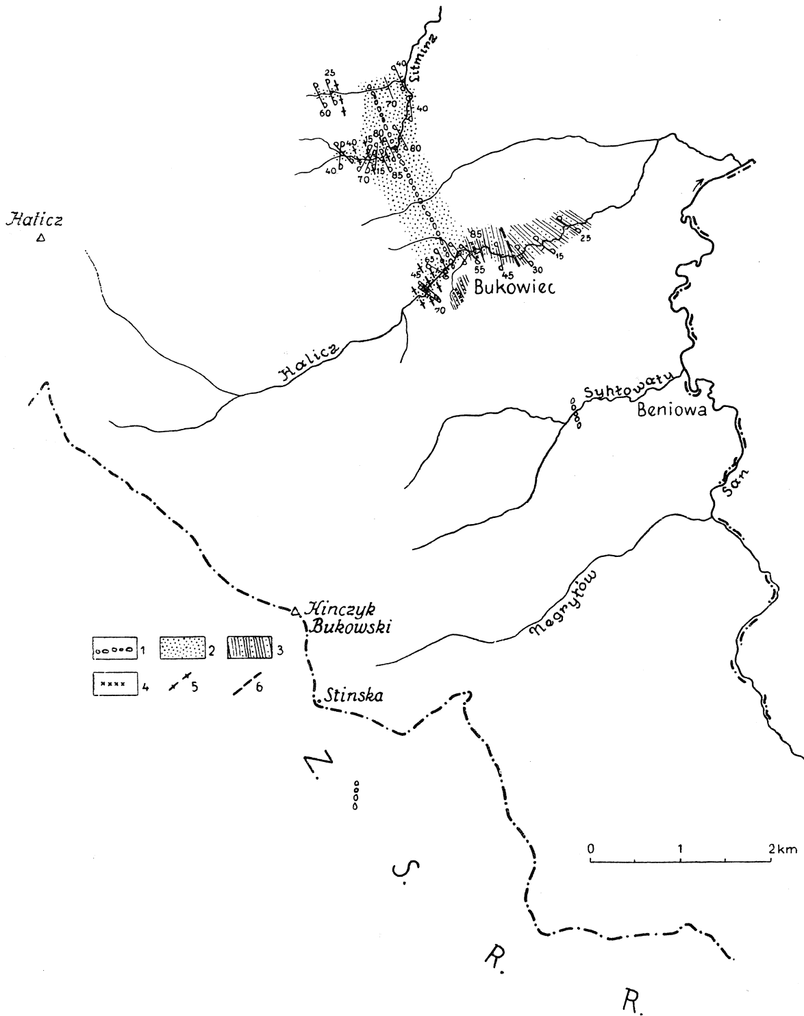
Fig. 1. Szkic geologiczny okolic Bukowca. 1 — poziom z egzotykami; 2 — warstwy krośnieńskie z przewagą piaskowców gruboławicowych; 3 — warstwy krośnieńskie z przewagą łupków; 4 — łupki jasielskie; 5 — oś antykliny; 6 — oś synkliny Fig. 1. Geological sketch of the vicinity of Bukowiec. 1 — exotic-bearing shales; 2 — thick-bedded sandstones of the Krosno beds; 3 — thin-bedded sandstones and shales of the Krosno beds; 4 — Jasło shales; 5 — axis of anticline; 6 — axis of syncline
