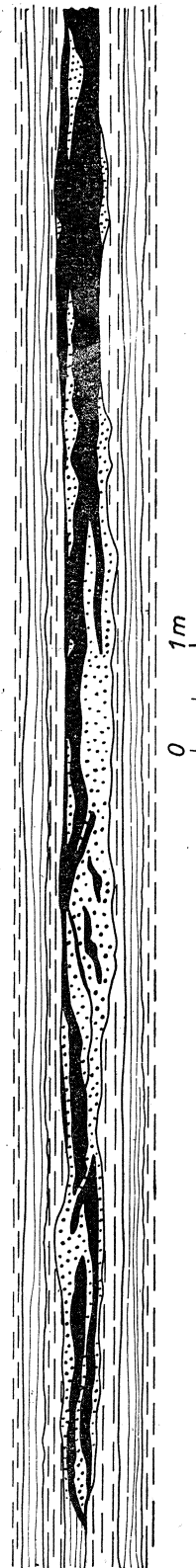
Fig. 7. Ławica osuwiskowa. Czarną barwą zaznaczone łupki redeponowane przez osuwisko Fig. 7. Slump-deposited bed. Shale fragments redeposited by the slump are shown in black
