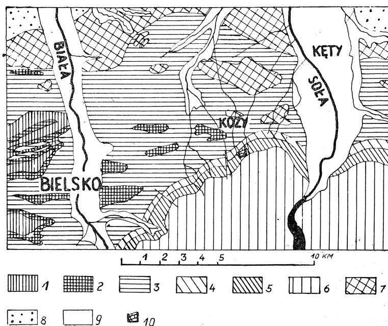
Fig. 2. Mapa geologiczna obszaru pomiędzy dolinami rzek Białej i Soły. 1 — dolne łupki cieszyńskie; 2 — wapień cieszyński; 3 — górne łupki cieszyńskie; 4 — warstwy wierzowskie; 5 — warstwy lgockie; 6 — warstwy godulskie; 7 — płaszczowina podśląska; 8 — miocen; 9 — aluwia; 10 — kamieniołom w Kozach; 1—3 — płaszczowina cieszyńska, 4—6 — płaszczowina godulska Fig. 2. Geological Map of the area situated between the valleys of Soła and Biała Rivers. 1 — Lower Cieszyn shales (Infravalanginian); 2 — Cieszyn limestones (Infravalanginian); 3 — Upper Cieszyn shales (Valanginian); 4 — Verovice shales (Barremian); 5 — Lgota Beds (Aptian — Lower Albanian); 6 — Godula Beds (Albanian — Cenomanian — Turonian); 7 — Sub-Silesian nappe; 8 — Miocene; 9 — Alluvia; 10 — The quarry at Kozy; 1—3 — Cieszyn nappe, 4—6 — Godula nappe
