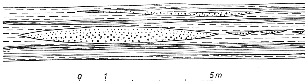
Fig. 9. Ławice soczewkowate. Widoczna gradacja ziarn w pionie i w poziomie Fig. 9. Lenticular beds displaying horizontal and vertical gradation
