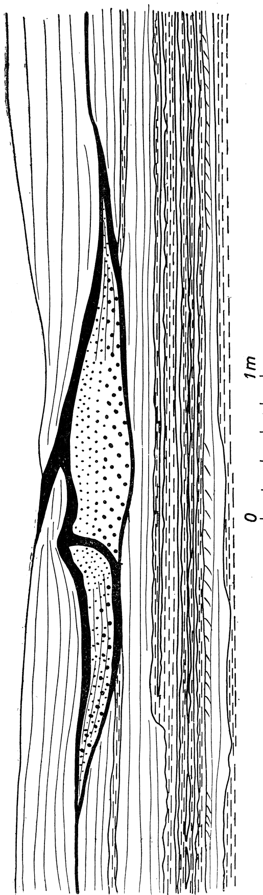
Fig. 10. Soczewka gruboziarnistego piasku wcięta erozyjnie w ławicę laminowaną. Widoczna gradacja ziarn w pionie i w poziomie. Czarną barwą zaznaczone redeponowane piaszczyste łupki mikowe Fig. 10. A lense of coarse grained sandstone cut in the underlying laminated bed. Sandy micaceous silts are shown in black
