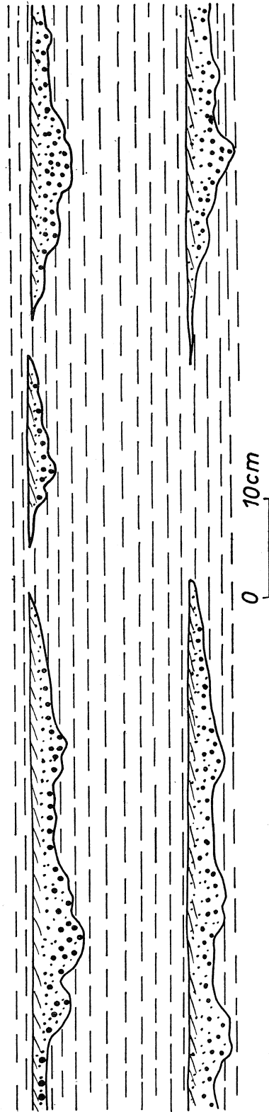
Fig. 8. Cienkie, soczewkowate ławice gruboziarnistego piaskowca Fig. 8. Thin lenticular beds of coarse-grained sandstone
