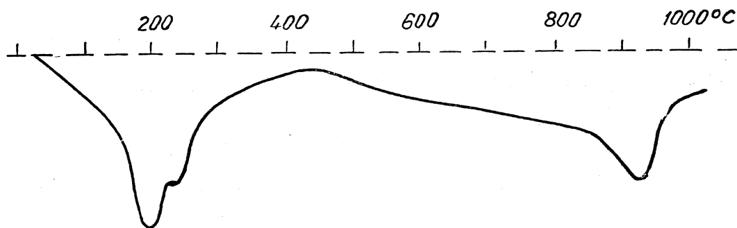
Fig. 3. Krzywa termiczna różnicowa próbki z głęb. 19,40 m, z otworu wiertniczego nr 43
