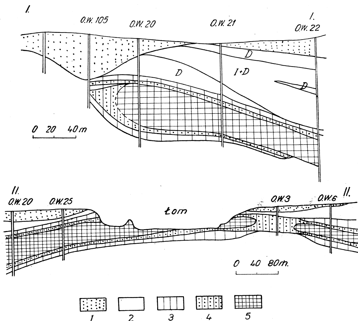
Fig. 2. Profile geologiczne przez złożę w Nowym Ładzie (wg R. Nielubowicza). I I — profil po upadzie; II II — profil po rozciągłości; 1 — dyluwium; 2 — górny cechsztyń (D — dolomit, I — iłolupek); 3 — górny cechsztyń — ciemny łupek z włóknistym gipsem; 4 — górny cechsztyń — gips; 5 — górny cechsztyń — anhydryt; o. w. — otwory wiertnicze
