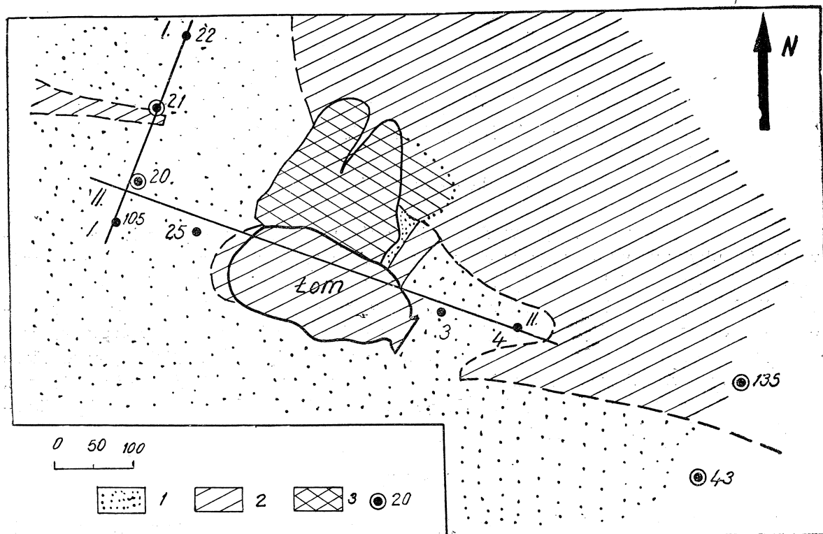
Fig. 1. Schematyczna mapa geologiczna rejonu łomu w Nowym Ładzie (wg. R. Nielubowicza). 1 — dyluwium; 2 — górny cechsztyń; 3 — hałdy; 4 — otwory wiertnicze zbadane petrograficznie; I I, II II — profile geologiczne (patrz fig. 2)
