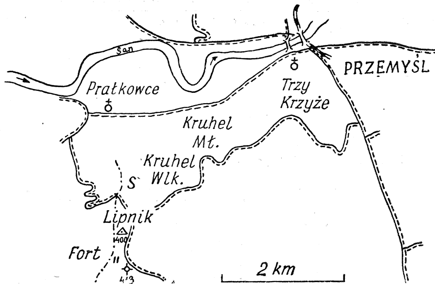
Fig. 1. Mapka okolicy Przemyśla Fort — ruiny starego fortu na wzgórzu (413 m) z odkrywkami opisanymi w tekście; S — skałka jurajska
