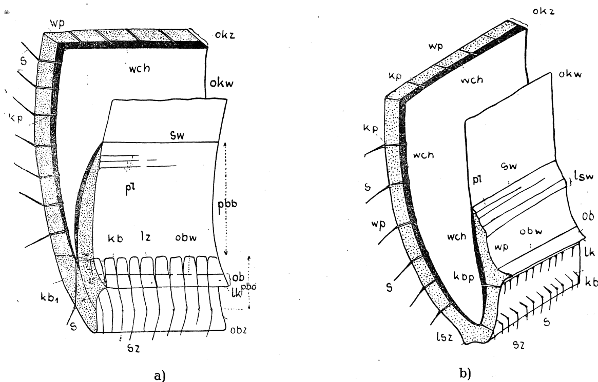
Fig. 4. a — brzeg skorupki jednoskładkowy, b — dwuskładkowy (schematycznie według Zalanii'ego); okz — okładka zewnętrzna; okw — okładka wewnętrzna; wp — warstwa zwapniała; wch — warstwa chitynowa wewnętrzna; s — szczec; kp — kanalik powierzchniowy poprzeczny; kb — kanalik brzeżny; sw — skraj wewnętrzny; sz — skraj zewnętrzny; ob — obwódka; lk — linia kantu; obw — wewnętrzna linia obwódki; obz — zewnętrzna linia obwódki; lz — linia zrostu; pbb — pole brzeżne bliższe; pbd — pole brzeżne dalsze; lsz — listwa zewnętrzna; lsw — listwa wewnętrzna.
