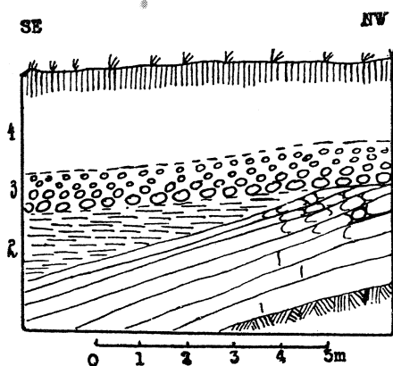
Ryc. 6. Profil łomu 5.
